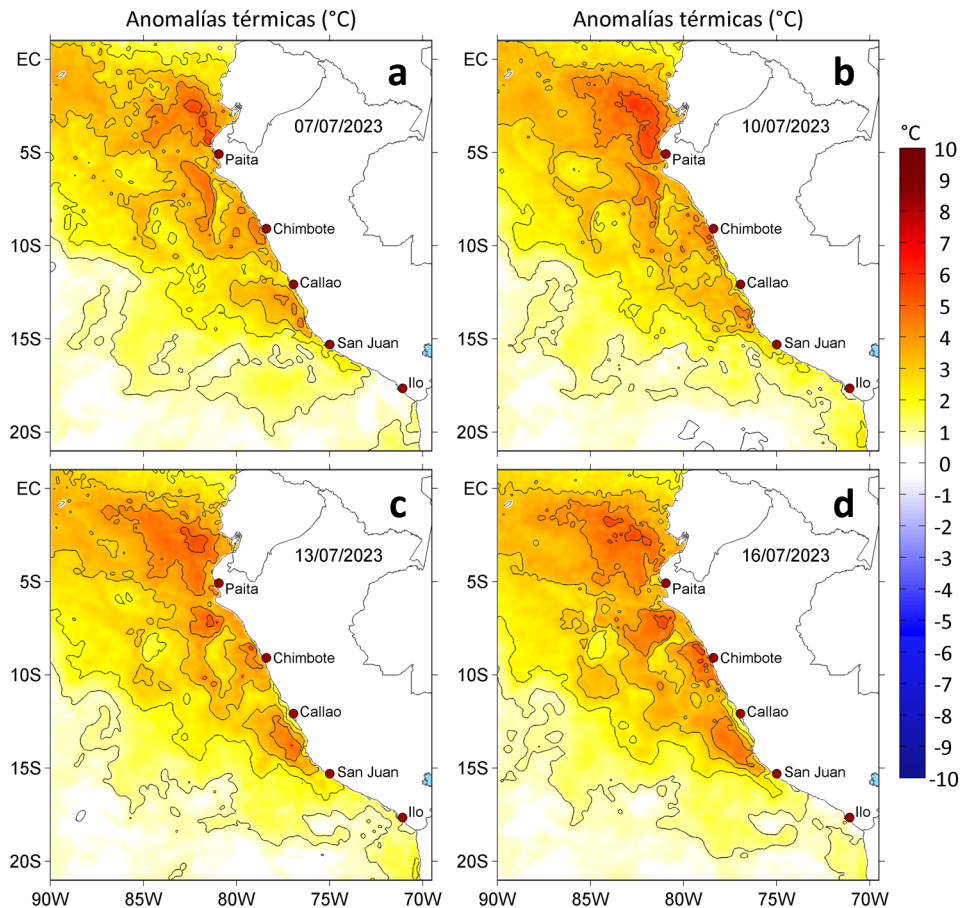
Figura 3. Anomalías de la temperatura superficial del mar ( ^{\circ}\text{C} ) para el a) 07, b) 10, c) 13 y d) 16 de julio de 2023. Las anomalías se calcularon respecto de la climatología para el periodo 2007-2016. Datos: OSTIA-UKMO-L4-GLOB-v2.0 (UK Met Office, 2012; Donlon et al, 2012).
