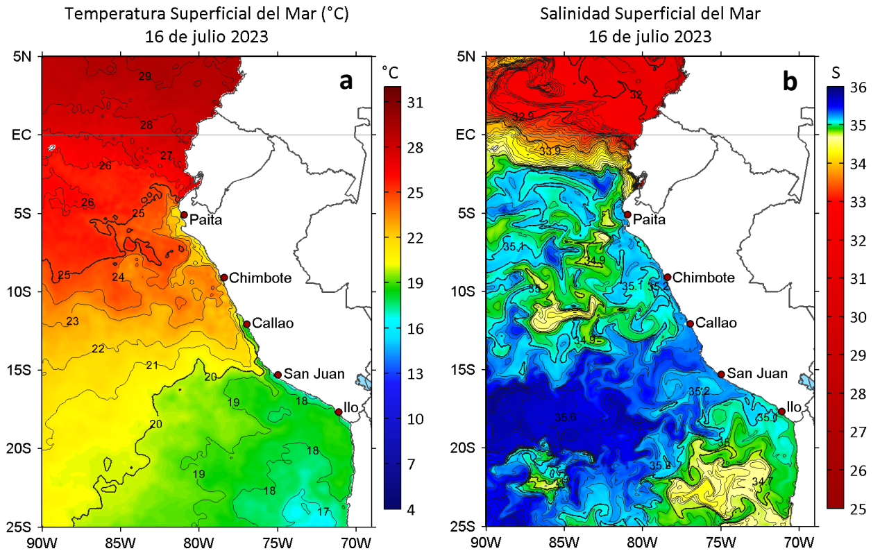
Figura 2. a) Temperatura superficial del mar ( ^{\circ}\text{C} ) y b) Salinidad superficial del mar para el 16 de julio de 2023. Datos: OSTIA-UKMO-L4-GLOB-v2.0 (UK Met Office, 2012; Donlon et al, 2012) y del GLOBAL_ANALYSISFORECAST_PHY_001_024 (Lellouche, J. M. et al, 2013), respectivamente.
