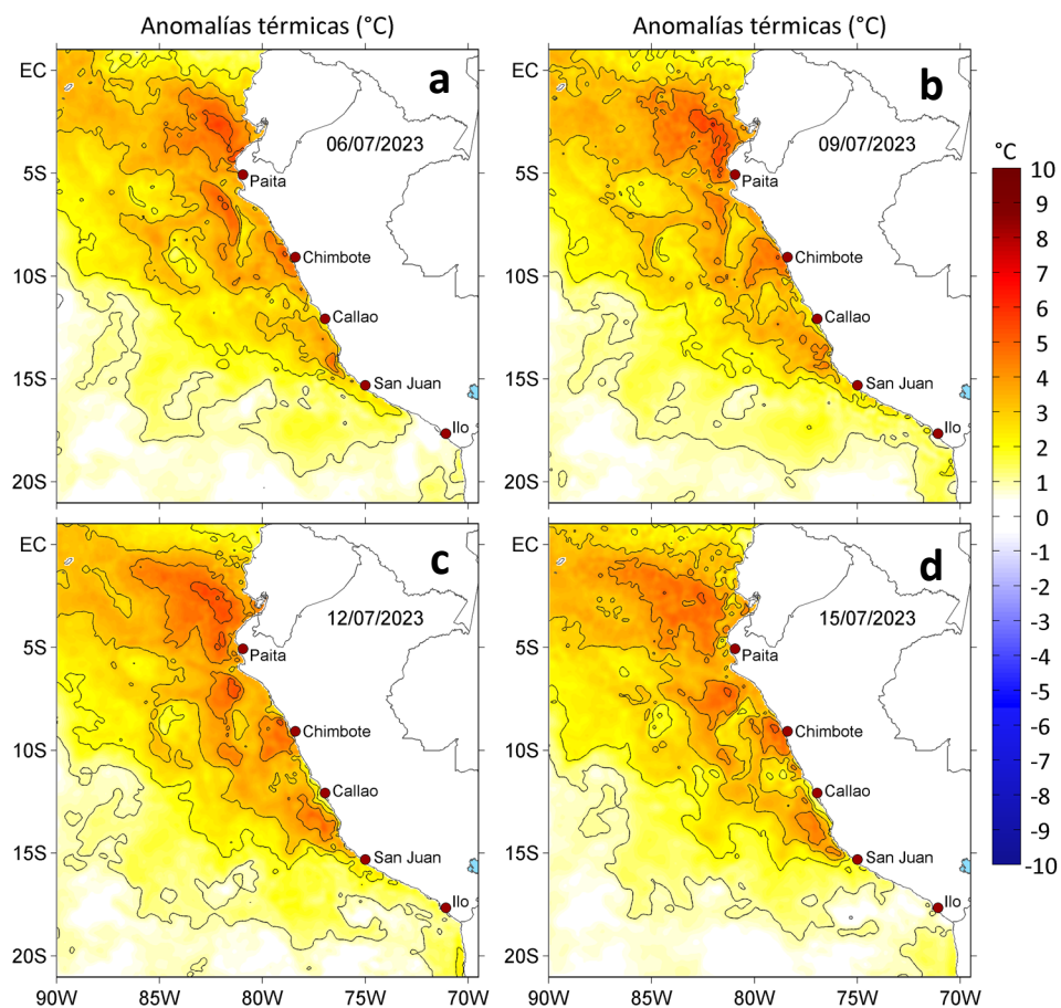
Figura 3. Anomalías de la temperatura superficial del mar ( ^{\circ}\text{C} ) para el a) 06, b) 09, c) 12 y d) 15 de julio de 2023. Las anomalías se calcularon respecto de la climatología para el periodo 2007-2016. Datos: OSTIA-UKMO-L4-GLOB-v2.0 (UK Met Office, 2012; Donlon et al, 2012).
