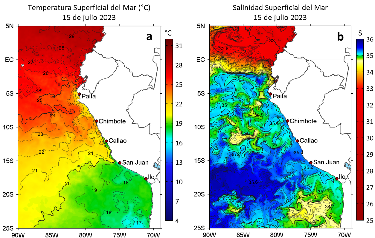
Figura 2. a) Temperatura superficial del mar ( ^{\circ}\text{C} ) y b) Salinidad superficial del mar para el 15 de julio de 2023. Datos: OSTIA-UKMO-L4-GLOB-v2.0 (UK Met Office, 2012; Donlon et al, 2012) y del GLOBAL_ANALYSISFORECAST_PHY_001_024 (Lellouche, J. M. et al, 2013), respectivamente.
