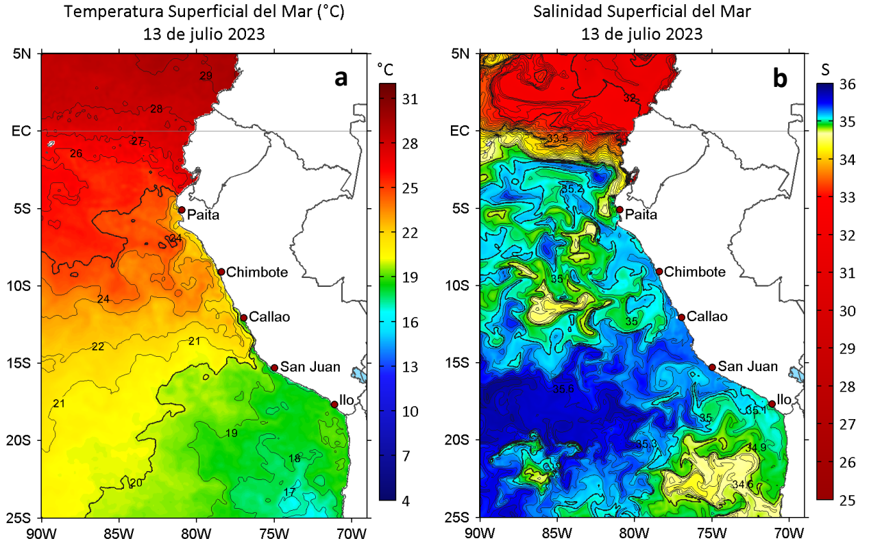
Figura 2. a) Temperatura superficial del mar ( ^{\circ}\text{C} ) y b) Salinidad superficial del mar para el 13 de julio de 2023. Datos: OSTIA-UKMO-L4-GLOB-v2.0 (UK Met Office, 2012; Donlon et al, 2012) y del GLOBAL_ANALYSISFORECAST_PHY_001_024 (Lellouche, J. M. et al, 2013), respectivamente.
