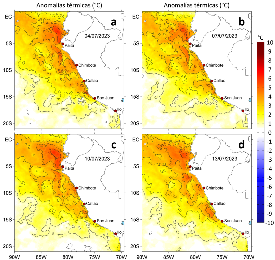
Figura 3. Anomalías de la temperatura superficial del mar ( ^{\circ}\text{C} ) para el a) 04, b) 07, c) 10 y d) 13 de julio de 2023. Las anomalías se calcularon respecto de la climatología para el periodo 2007-2016. Datos: OSTIA-UKMO-L4-GLOB-v2.0 (UK Met Office, 2012; Donlon et al, 2012).
