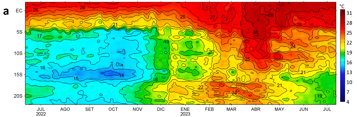
Anomalías de la Temperatura Superficial del mar (°C), franja costera de 60 m.n. 11 de junio 2022 - 12 de julio 2023
