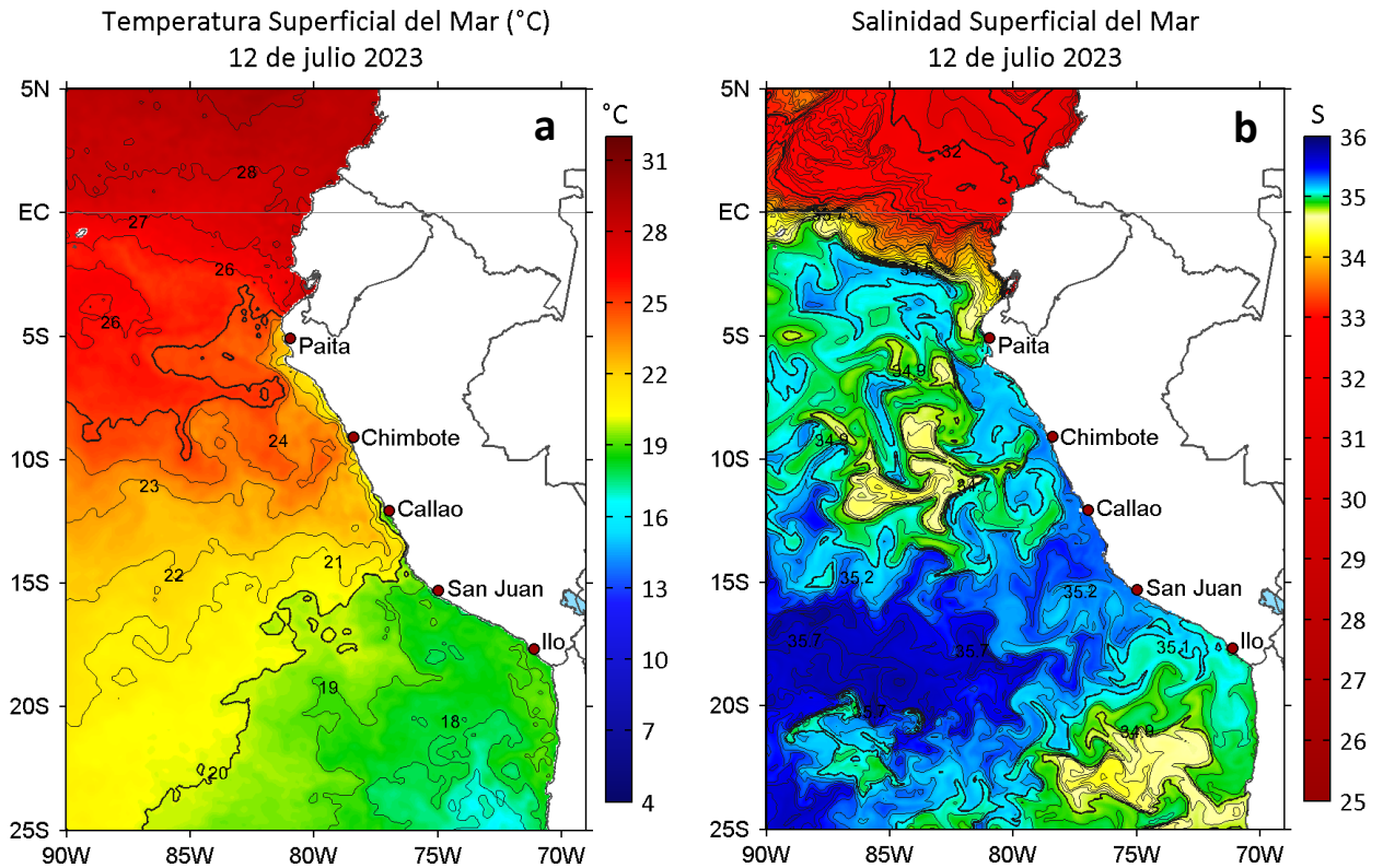
Figura 2. a) Temperatura superficial del mar ( ^{\circ}\text{C} ) y b) Salinidad superficial del mar para el 12 de julio de 2023. Datos: OSTIA-UKMO-L4-GLOB-v2.0 (UK Met Office, 2012; Donlon et al, 2012) y del GLOBAL_ANALYSISFORECAST_PHY_001_024 (Lellouche, J. M. et al, 2013), respectivamente.
