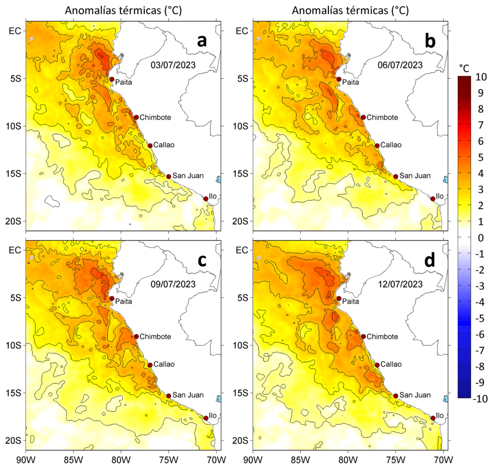
Figura 3. Anomalías de la temperatura superficial del mar ( ^{\circ}\text{C} ) para el a) 03, b) 06, c) 09 y d) 12 de julio de 2023. Las anomalías se calcularon respecto de la climatología para el periodo 2007-2016. Datos: OSTIA-UKMO-L4-GLOB-v2.0 (UK Met Office, 2012; Donlon et al, 2012).
