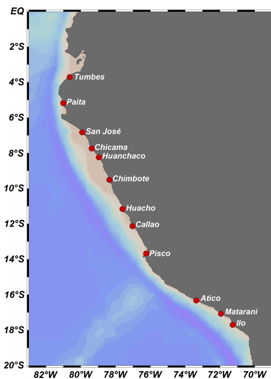
Figura 1. Localización de las estaciones oceanográficas del IMARPE (círculos de color rojo) en el litoral peruano.
