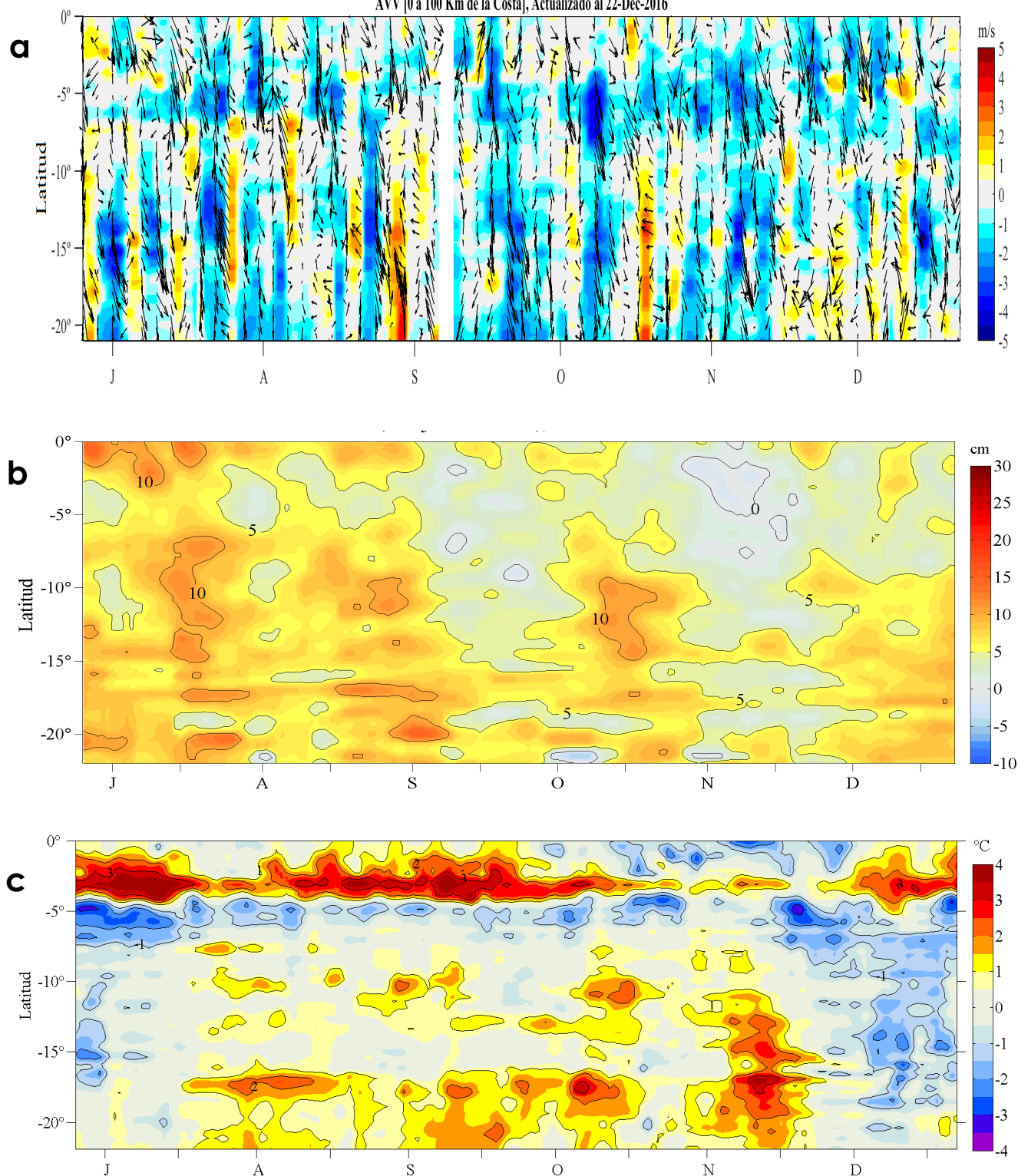
Figura 4. Evolución de las anomalías diarias de: a) velocidad del viento (m/s), b) nivel medio del mar (cm), c) temperatura superficial del mar (°C) para el último semestre actualizado al 22 de diciembre de 2016. Datos: de IFREMER/CERSAT para (a), del Servicio de Monitoreo del Ambiente Marino Copernicus (CMEMS, según sus siglas en inglés) para (b) del satélite AVHRR v2 del Centro Nacional de Datos Climáticos de la Administración Nacional del Océano y la Atmósfera (NCDC/NOAA, según sus siglas en inglés) para (c). Las anomalías fueron calculadas para una franja de 100 km adyacente a la costa entre el ecuador y 21°S según los promedios climatológicos diarios de 2000-2014 para (a), de 1993-2013 para (b) y de 1982-2011 para (c). La barra de colores a la derecha muestra la escala de las anomalías en cada caso. Procesamiento: LHF/AFIOF/DGIOCC/IMARPE.
