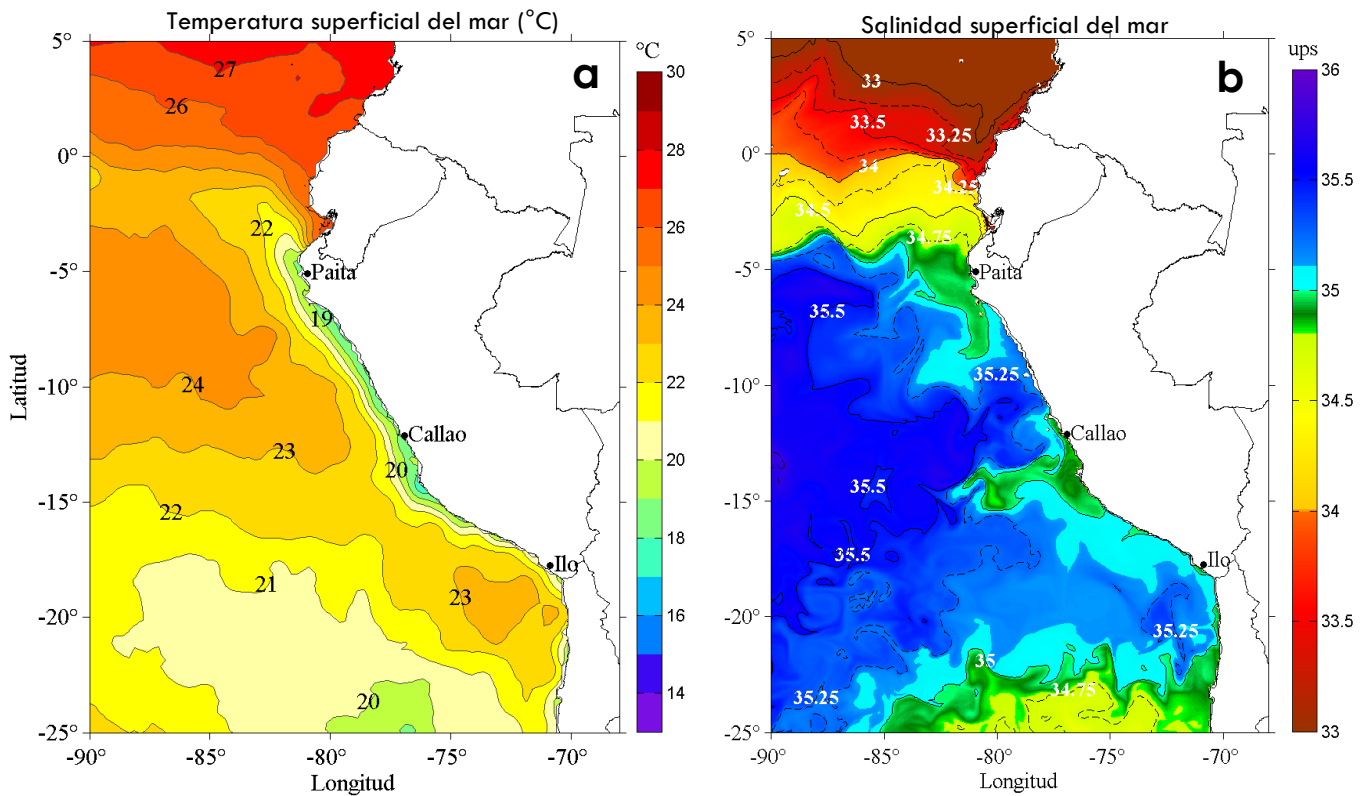
Figura 1. Distribución espacial promedio de: a) Temperatura Superficial del Mar (°C) y b) Salinidad Superficial del Mar, para la semana del 16 al 22 de diciembre de 2016 en el océano Pacífico tropical oriental. Datos: AVHRR v2 del Centro Nacional de Datos Climáticos de la Administración Nacional del Océano y la Atmósfera (NCDC/NOAA, según sus siglas en inglés) para (a) y del HYbrid Coordinate Ocean Model (HYCOM; Halliwell et al., 1998; 2000; Bleck, 2001) para (b). Las escalas de colores de la temperatura como de la salinidad superficial del mar se presentan a la derecha de cada gráfico. Procesamiento: LHFm/AFIOF/DGIOCC/IMARPE.
