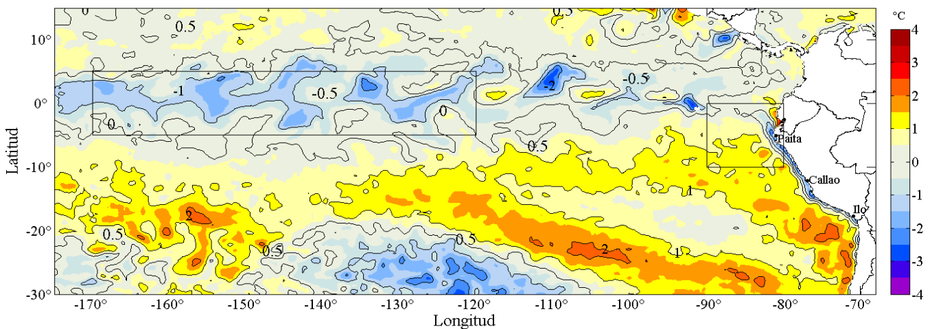
Figura 2. Anomalías promedio de la temperatura superficial del mar (°C) en el océano Pacífico tropical para la semana del 16 al 22 de diciembre de 2016. Las regiones Niño 3.4 y Niño 1+2 en los sectores central y oriental del océano, respectivamente, están delimitadas con una línea de color gris. Datos: AVHRR Global Reyn_SmithOlv2R (Reynolds, et al., 2007) de CMB/EMC/NCEP de la Administración Nacional del Océano y la Atmósfera (NOAA, según sus siglas en inglés). Las anomalías se calcularon con respecto de la climatología para el período 1982-2011. Procesamiento: IMARPE.
