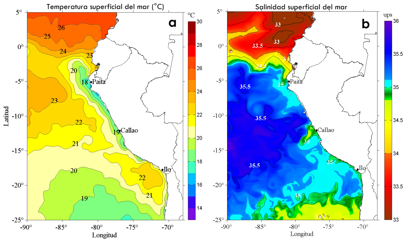
Figura 1. Distribución espacial promedio de: a) Temperatura Superficial del Mar (°C) y b) Salinidad Superficial del Mar, para la semana del 18 al 24 de noviembre de 2016 en el océano Pacífico tropical oriental. Datos: AVHRR v2 del Centro Nacional de Datos Climáticos de la Administración Nacional del Océano y la Atmósfera (NCDC/NOAA, según sus siglas en inglés) para (a) y del HYbrid Coordinate Ocean Model (HYCOM; Halliwell et al., 1998; 2000; Bleck, 2001) para (b). Las escalas de colores de la temperatura como de la salinidad superficial del mar se presentan a la derecha de cada gráfico. Procesamiento: LHFM/AFIOF/DGIOCC/IMARPE.
