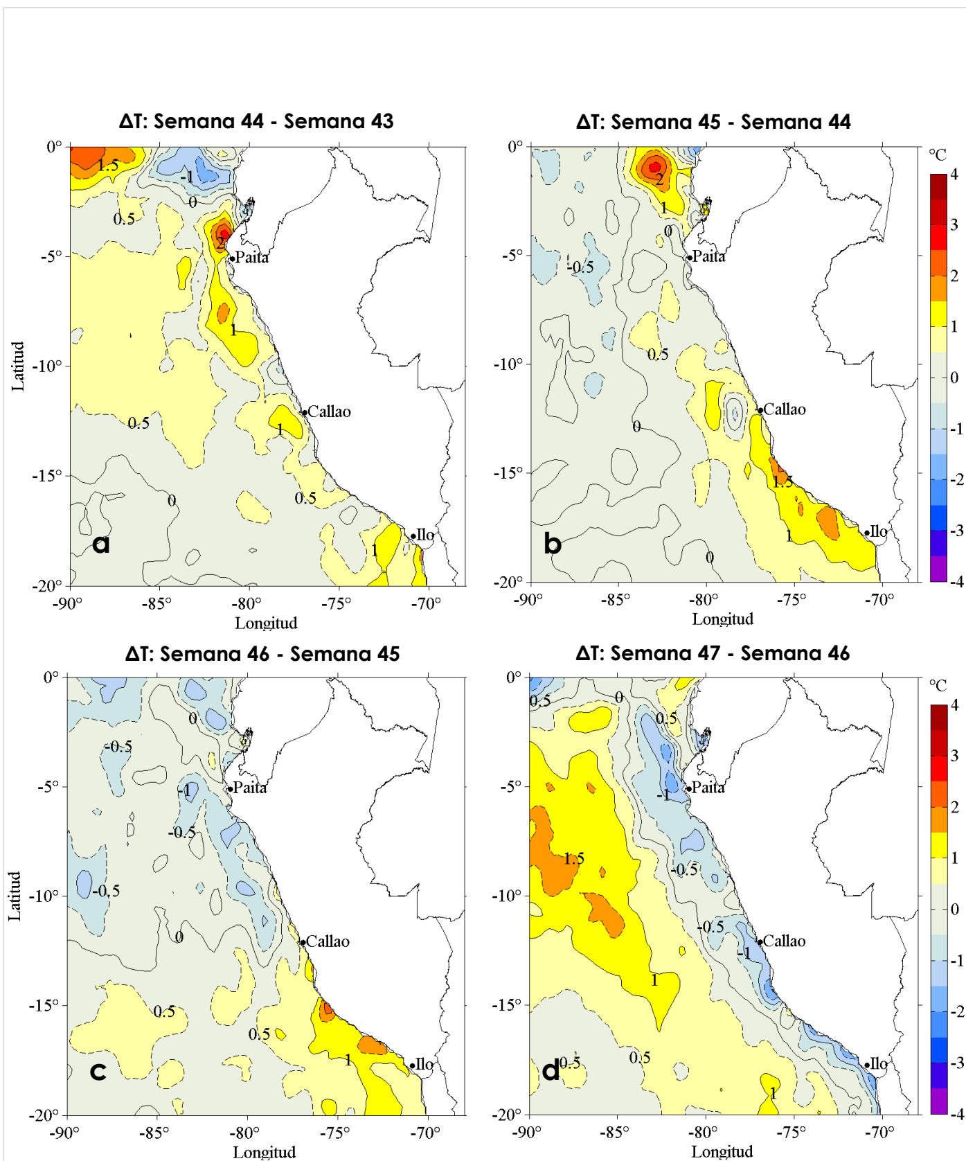
Figura 3. Variación semanal de la anomalía de la temperatura superficial del mar promedio (°C) en el océano Pacífico tropical oriental entre: a) la cuadragésimo cuarta (28 de octubre - 03 de noviembre) y cuadragésimo tercera (21 - 27 de octubre) semana, b) la cuadragésimo quinta (04 - 10 de noviembre) y cuadragésimo cuarta (28 de octubre - 03 de noviembre) semana, c) la cuadragésimo sexta (11 - 17 de noviembre) y cuadragésimo quinta (04 - 10 de noviembre) semana, y d) la cuadragésimo séptima (18 - 24 de noviembre) y cuadragésimo sexta (11 - 17 de noviembre) semana del presente año. Los mapas, que indican el grado de calentamiento o enfriamiento de una semana a otra, provienen del sensor AVHRR v2 del Centro Nacional de Datos Climáticos de la Administración Nacional del Océano y la Atmósfera (NCDC/NOAA, según sus siglas en inglés). Las anomalías térmicas se calcularon de acuerdo con la climatología para el período 1982-2011. La barra de colores de las anomalías térmicas se presenta a la derecha. Procesamiento: LHFM/AFIOF/DGIOCC/IMARPE.
