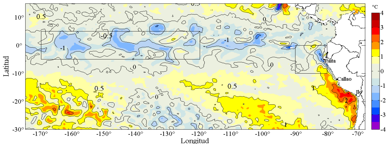
Figura 2. Anomalías promedio de la temperatura superficial del mar (°C) en el océano Pacífico tropical para la semana del 18 al 24 de noviembre de 2016. Las regiones Niño 3.4 y Niño 1+2 en los sectores central y oriental del océano, respectivamente, están delimitadas con una línea de color gris. Datos: AVHRR Global Reyn_SmithOlv2R (Reynolds, et. al., 2007) de CMB/EMC/NCEP de la Administración Nacional del Océano y la Atmósfera (NOAA, según sus siglas en inglés). Las anomalías se calcularon con respecto de la climatología para el período 1982-2011. Procesamiento: IMARPE.
