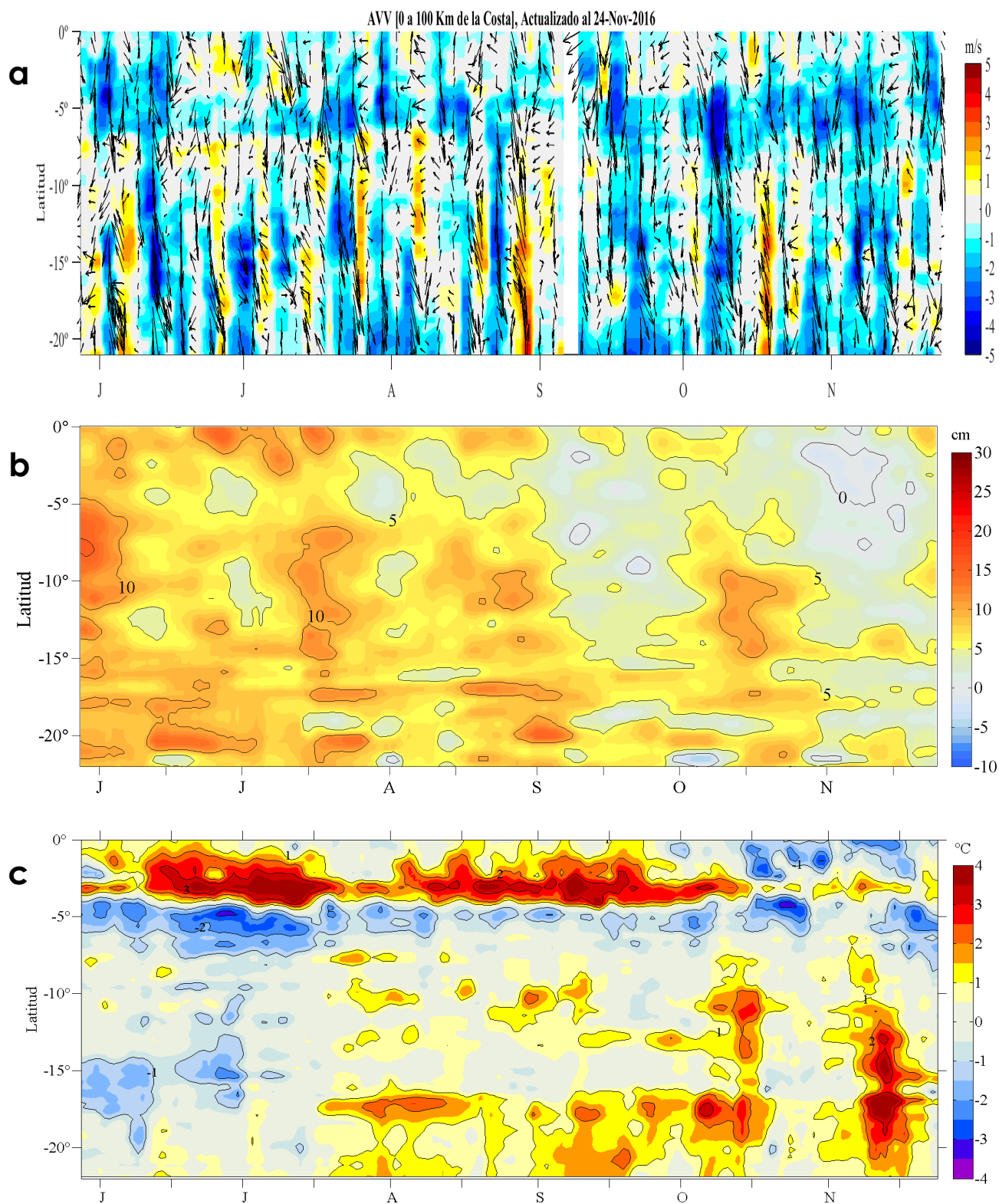
Figura 4. Evolución de las anomalías diarias de: a) velocidad del viento (m/s), b) nivel medio del mar (cm), c) temperatura superficial del mar (°C) para el último semestre actualizado al 24 de noviembre de 2016. Datos: de IFREMER/CERSAT para (a), del Servicio de Monitoreo del Ambiente Marino Copernicus (CMEMS, según sus siglas en inglés) para (b) del satélite AVHRR v2 del Centro Nacional de Datos Climáticos de la Administración Nacional del Océano y la Atmósfera (NCDC/NOAA, según sus siglas en inglés) para (c). Las anomalías fueron calculadas para una franja de 100 km adyacente a la costa entre el ecuador y 21°S según los promedios climatológicos diarios de 2000-2014 para (a), de 1993-2013 para (b) y de 1982-2011 para (c). La barra de colores a la derecha muestra la escala de las anomalías en cada caso. Procesamiento: LHFm/AFIOF/DGIOCC/IMARPE.
