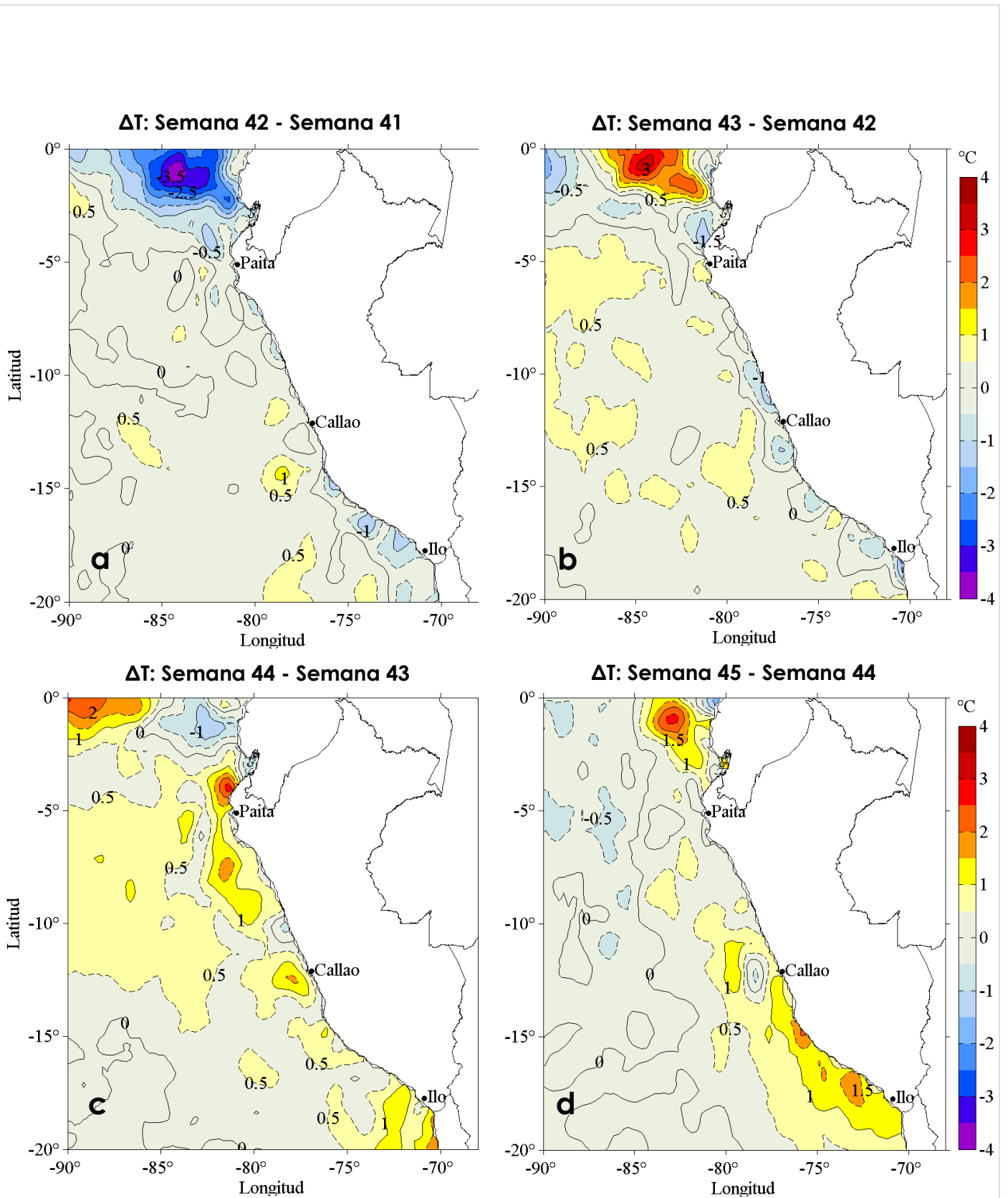
Figura 3. Variación semanal de la anomalía de la temperatura superficial del mar promedio (°C) en el océano Pacífico tropical oriental entre: a) la cuadragésimo segunda (14 - 20 de octubre) y cuadragésimo primera (07 - 13 de octubre) semana, b) la cuadragésimo tercera (21 - 27 de octubre) y cuadragésimo segunda (14 - 20 de octubre) semana, c) la cuadragésimo cuarta (28 de octubre - 03 de noviembre) y cuadragésimo tercera (21 - 27 de octubre) semana, y d) la cuadragésimo quinta (04 - 10 de noviembre) y cuadragésimo cuarta (28 de octubre - 03 de noviembre) semana del presente año. Los mapas, que indican el grado de calentamiento o enfriamiento de una semana a otra, provienen del sensor AVHRR v2 del Centro Nacional de Datos Climáticos de la Administración Nacional del Océano y la Atmósfera (NCDC/NOAA, según sus siglas en inglés). Las anomalías térmicas se calcularon de acuerdo con la climatología para el período 1982-2011. La barra de colores de las anomalías térmicas se presenta a la derecha. Procesamiento: LHFM/AFIOF/DGIOCC/IMARPE.
