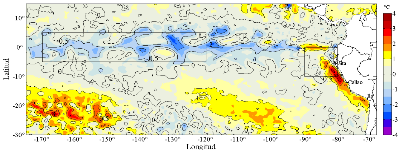
Figura 2. Anomalías promedio de la temperatura superficial del mar (°C) en el océano Pacífico tropical para la semana del 04 al 10 de noviembre de 2016. Las regiones Niño 3.4 y Niño 1+2 en los sectores central y oriental del océano, respectivamente, están delimitadas con una línea de color gris. Datos: AVHRR Global Reyn_SmithOlv2R (Reynolds, et al., 2007) de CMB/EMC/NCEP de la Administración Nacional del Océano y la Atmósfera (NOAA, según sus siglas en inglés). Las anomalías se calcularon con respecto de la climatología para el período 1982-2011. Procesamiento: IMARPE.
