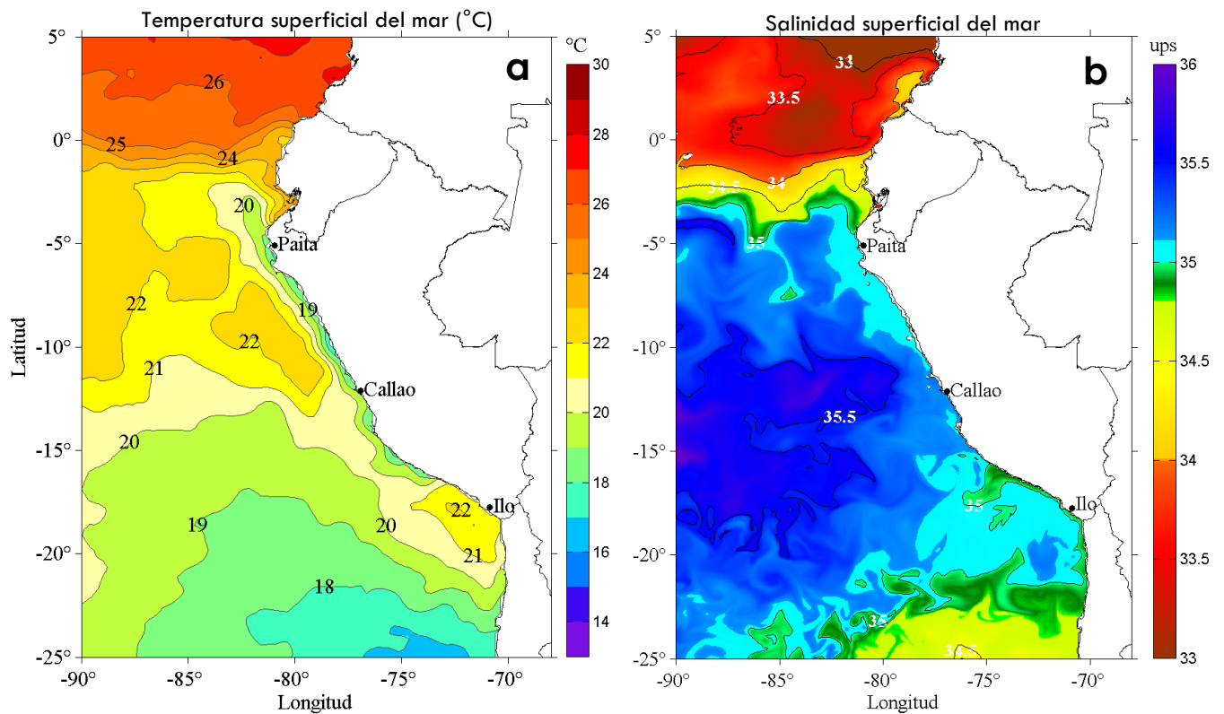
Figura 1. Distribución espacial promedio de: a) Temperatura Superficial del Mar (°C) y b) Salinidad Superficial del Mar, para la semana del 04 al 10 de noviembre de 2016 en el océano Pacífico tropical oriental. Datos: AVHRR v2 del Centro Nacional de Datos Climáticos de la Administración Nacional del Océano y la Atmósfera (NCDC/NOAA, según sus siglas en inglés) para (a) y del HYbrid Coordinate Ocean Model (HYCOM; Halliwell et al., 1998; 2000; Bleck, 2001) para (b). Las escalas de colores de la temperatura como de la salinidad superficial del mar se presentan a la derecha de cada gráfico. Procesamiento: LHFM/AFIOF/DGIOCC/IMARPE.
