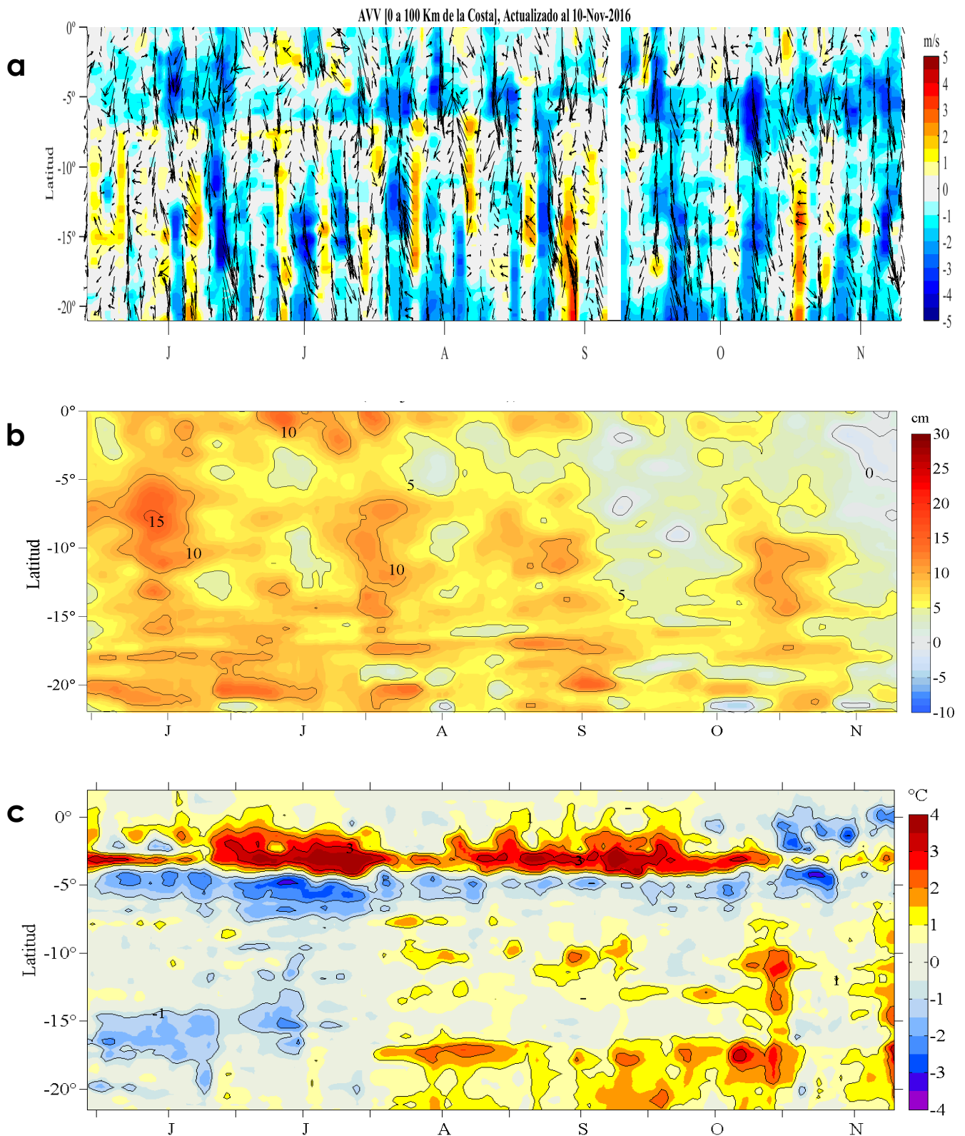
Figura 4. Evolución de las anomalías diarias de: a) velocidad del viento (m/s), b) nivel medio del mar (cm), c) temperatura superficial del mar (°C) para el último semestre actualizado al 10 de noviembre de 2016. Datos: de IFREMER/CERSAT para (a), del Servicio de Monitoreo del Ambiente Marino Copernicus (CMEMS, según sus siglas en inglés) para (b) del satélite AVHRR v2 del Centro Nacional de Datos Climáticos de la Administración Nacional del Océano y la Atmósfera (NCDC/NOAA, según sus siglas en inglés) para (c). Las anomalías fueron calculadas para una franja de 100 km adyacente a la costa entre el ecuador y 21°S según los promedios climatológicos diarios de 2000-2014 para (a), de 1993-2013 para (b) y de 1982-2011 para (c). La barra de colores a la derecha muestra la escala de las anomalías en cada caso. Procesamiento: LHF/AFIOF/DGIOCC/IMARPE.
