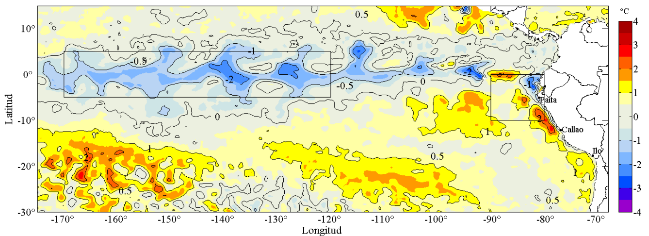
Figura 2. Anomalías promedio de la temperatura superficial del mar (°C) en el océano Pacífico tropical para la semana del 28 de octubre al 03 de noviembre de 2016. Las regiones Niño 3.4 y Niño 1+2 en los sectores central y oriental del océano, respectivamente, están delimitadas con una línea de color gris. Datos: AVHRR Global Reyn_SmithOIv2R (Reynolds, et al., 2007) de CMB/EMC/NCEP de la Administración Nacional del Océano y la Atmósfera (NOAA, según sus siglas en inglés). Las anomalías se calcularon con respecto de la climatología para el período 1982-2011. Procesamiento: IMARPE.
