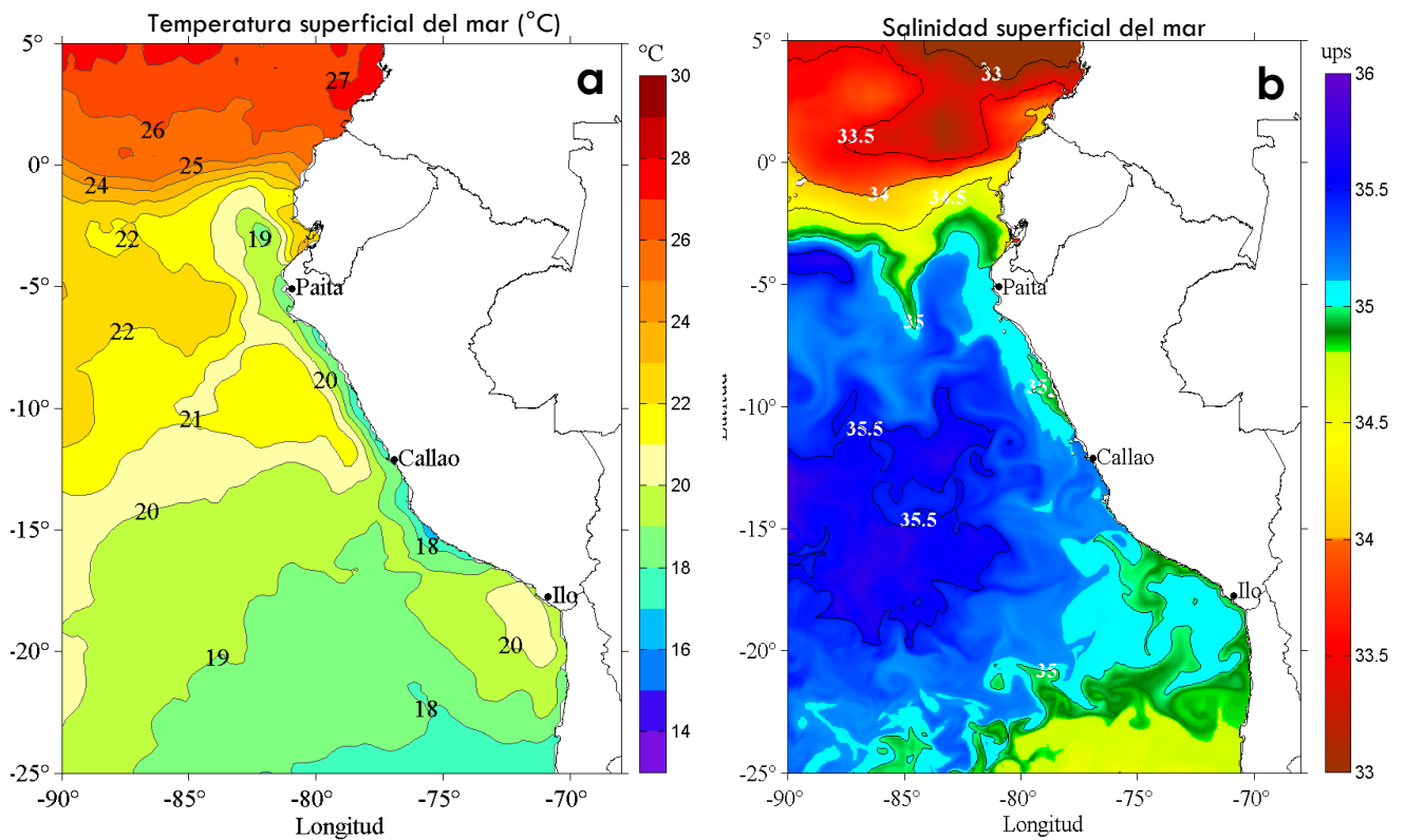
Figura 1. Distribución espacial promedio de: a) Temperatura Superficial del Mar (°C) y b) Salinidad Superficial del Mar, para la semana del 28 de octubre al 03 de noviembre de 2016 en el océano Pacífico tropical oriental. Datos: AVHRR v2 del Centro Nacional de Datos Climáticos de la Administración Nacional del Océano y la Atmósfera (NCDC/NOAA, según sus siglas en inglés) para (a) y del HYbrid Coordinate Ocean Model (HYCOM; Halliwell et al., 1998; 2000; Bleck, 2001) para (b). Las escalas de colores de la temperatura como de la salinidad superficial del mar se presentan a la derecha de cada gráfico. Procesamiento: LHFm/AFIOF/DGIOCC/IMARPE.
