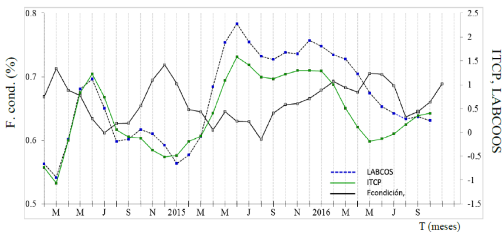
Figura 7. Series de tiempo del Índice LABCOS (línea punteada de color azul), del Índice Térmico Costero Peruano (ITCP, línea de color azul) y del Factor de Condición (% en color negro) desde febrero de 2014. La metodología para estimar estos índices se encuentran en Quispe y Vásquez (2015) para el LABCOS y Perea et al (2015) para el Factor de Condición. Procesamiento: IMARPE.
