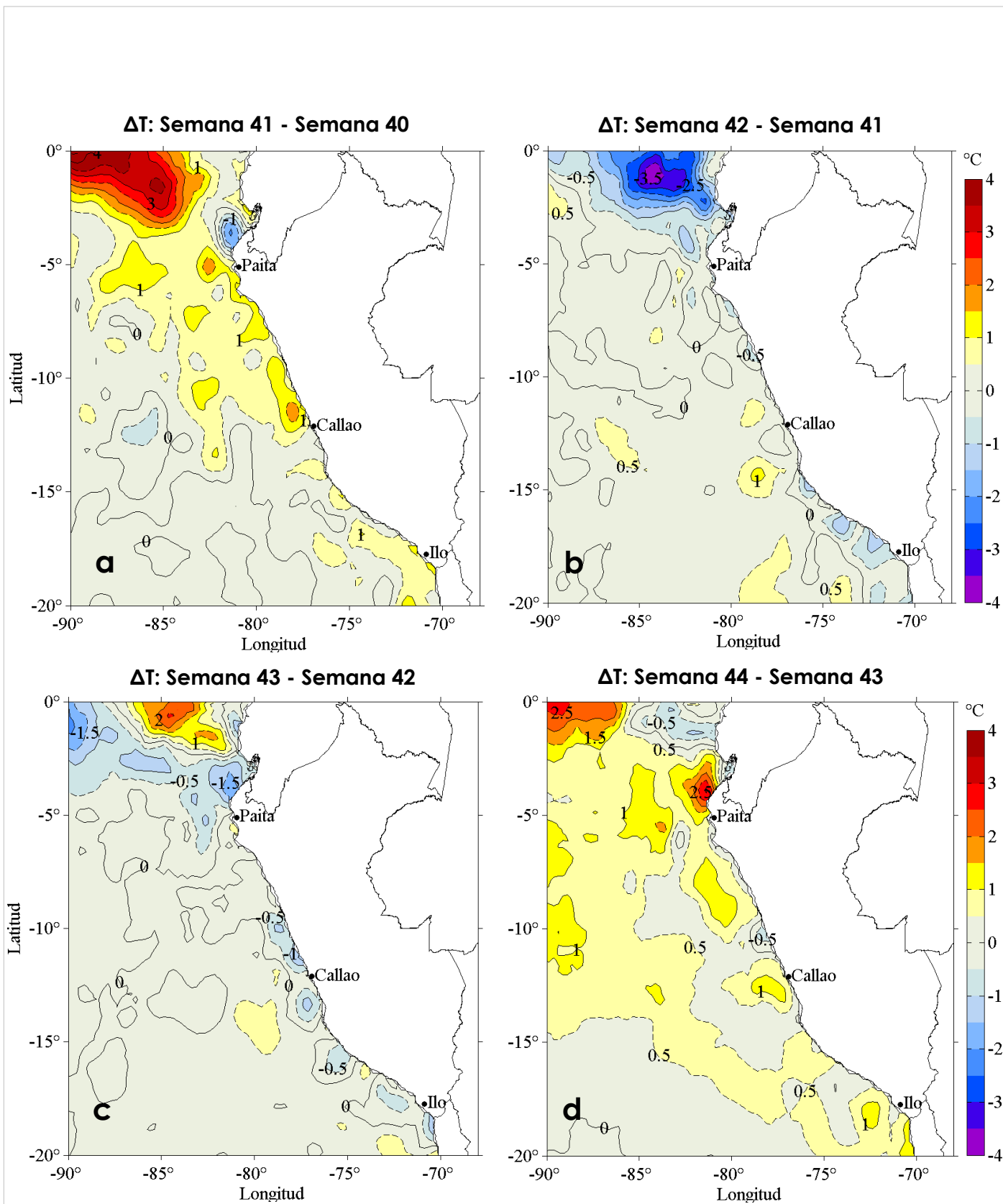
Figura 3. Variación semanal de la anomalía de la temperatura superficial del mar promedio (°C) en el océano Pacífico tropical oriental entre: a) la cuadragésimo primera (07 - 13 de octubre) y cuadragésima (30 de setiembre - 06 de octubre) semana, b) la cuadragésimo segunda (14 - 20 de octubre) y cuadragésimo primera (07 - 13 de octubre) semana, c) la cuadragésimo tercera (21 - 27 de octubre) y cuadragésimo segunda (14 - 20 de octubre) semana, y d) la cuadragésimo cuarta (28 de octubre - 03 de noviembre) y cuadragésimo tercera (21 - 27 de octubre) semana del presente año. Los mapas, que indican el grado de calentamiento o enfriamiento de una semana a otra, provienen del sensor AVHRR v2 del Centro Nacional de Datos Climáticos de la Administración Nacional del Océano y la Atmósfera (NCDC/NOAA, según sus siglas en inglés). Las anomalías térmicas se calcularon de acuerdo con la climatología para el período 1982-2011. La barra de colores de las anomalías térmicas se presenta a la derecha. Procesamiento: LHF/M/AFIOF/DGIOCC/IMARPE.
