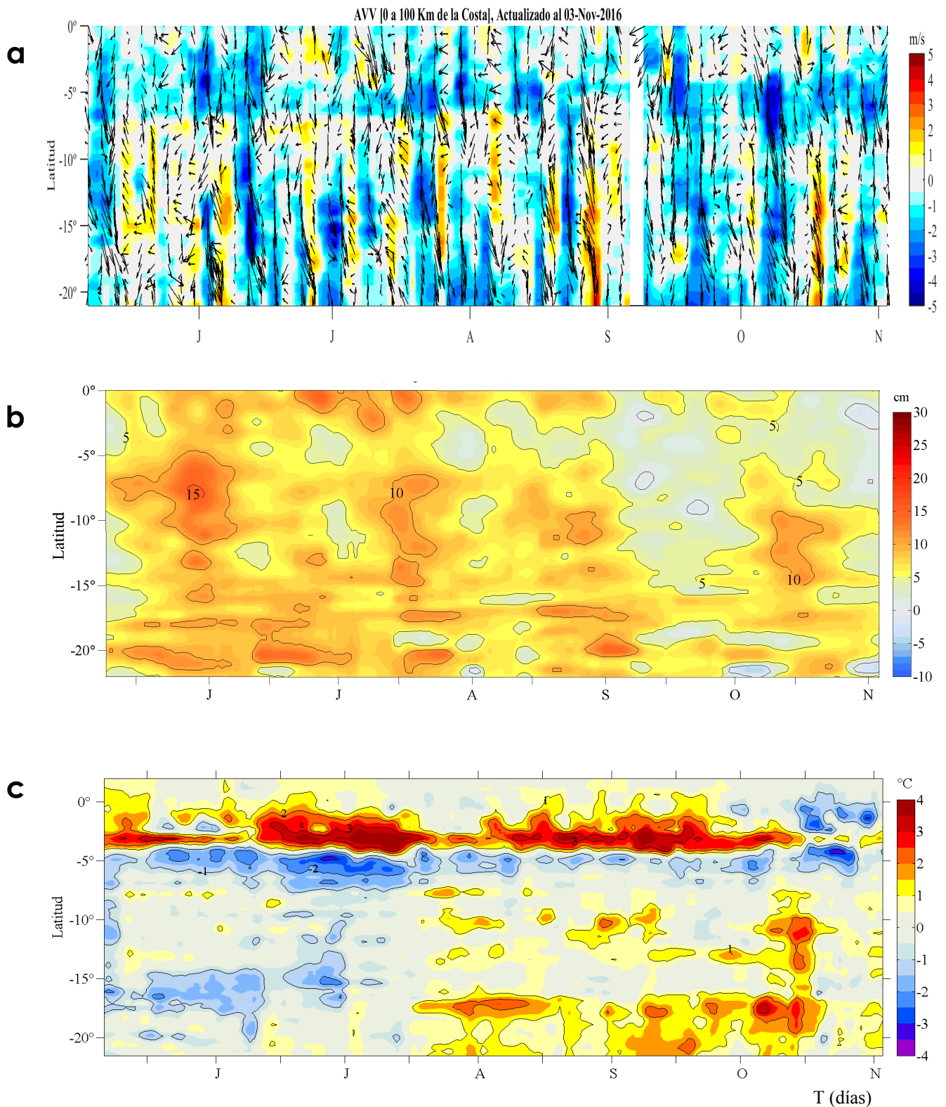
Figura 4. Evolución de las anomalías diarias de: a) velocidad del viento (m/s), b) nivel medio del mar (cm), y c) temperatura superficial del mar (°C) para el último semestre actualizado al 03 de noviembre de 2016. Datos: de IFREMER/CERSAT para (a), del Servicio de Monitoreo del Ambiente Marino Copernicus (CMEMS, según sus siglas en inglés) para (b), del satélite AVHRR v2 del Centro Nacional de Datos Climáticos de la Administración Nacional del Océano y la Atmósfera (NCDC/NOAA, según sus siglas en inglés) para (c). Las anomalías fueron calculadas para una franja de 100 km adyacente a la costa entre el ecuador y 21°S según los promedios climatológicos diarios de 2000-2014 para (a), de 1993-2013 para (b) y de 1982-2011 para (c). La barra de colores a la derecha muestra la escala de las anomalías en cada caso. Procesamiento: LHF/AFIOF/DGIOCC/IMARPE.
