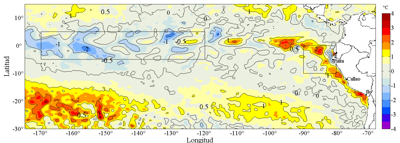
Figura 2. Anomalías promedio de la temperatura superficial del mar (°C) en el océano Pacífico tropical para la semana del 07 al 13 de octubre de 2016. Las regiones Niño 3.4 y Niño 1+2 en los sectores central y oriental del océano, respectivamente, están delimitadas con una línea de color gris. Datos: AVHRR Global Reyn_SmithOlv2R (Reynolds, et al., 2007) de CMB/EMC/NCEP de la Administración Nacional del Océano y la Atmósfera (NOAA, según sus siglas en inglés). Las anomalías se calcularon con respecto de la climatología para el período 1982-2011. Procesamiento: IMARPE.
