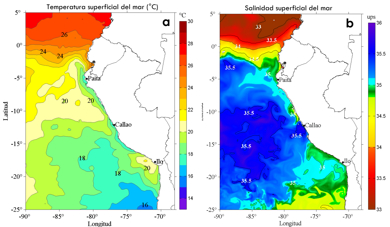
Figura 1. Distribución espacial promedio de: a) Temperatura Superficial del Mar (°C) y b) Salinidad Superficial del Mar, para la semana del 07 al 13 de octubre de 2016 en el océano Pacífico tropical oriental. Datos: AVHRR v2 del Centro Nacional de Datos Climáticos de la Administración Nacional del Océano y la Atmósfera (NCDC/NOAA, según sus siglas en inglés) para (a) y del Hybrid Coordinate Ocean Model (HYCOM; Halliwell et al., 1998; 2000; Bleck, 2001) para (b). Las escalas de colores de la temperatura como de la salinidad superficial del mar se presentan a la derecha de cada gráfico. Procesamiento: LHFH/AFIOF/DGIOCC/IMARPE.
