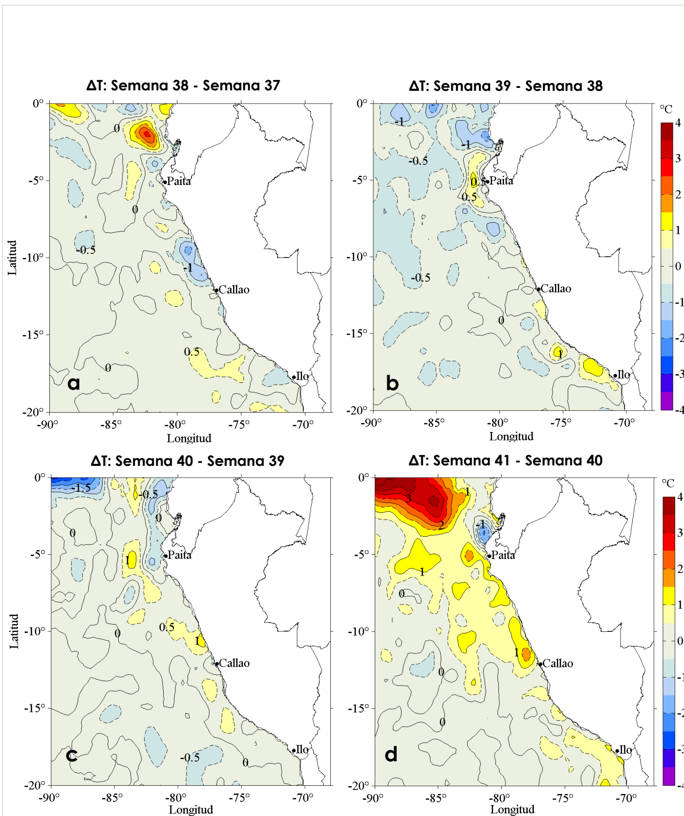
Figura 3. Variación semanal de la anomalía de la temperatura superficial del mar promedio (°C) en el océano Pacífico tropical oriental entre: a) la trigésimo octava (16 - 22 de setiembre) y trigésimo séptima (09 - 15 de setiembre) semana, b) la trigésimo novena (23 - 29 de setiembre) y trigésimo octava (16 - 22 de setiembre) semana, c) la cuadragésima (30 de setiembre - 06 de octubre) y trigésimo novena (23 - 29 de setiembre) semana, y d) la cuadragésimo primera (07 - 13 de octubre) y cuadragésima (30 de setiembre - 06 de octubre) semana del presente año. Los mapas, que indican el grado de calentamiento o enfriamiento de una semana a otra, provienen del sensor AVHRR v2 del Centro Nacional de Datos Climáticos de la Administración Nacional del Océano y la Atmósfera (NCDC/NOAA, según sus siglas en inglés). Las anomalías térmicas se calcularon de acuerdo con la climatología para el período 1982-2011. La barra de colores de las anomalías térmicas se presenta a la derecha. Procesamiento: LHF/AFIOF/DGIOCC/IMARPE.
