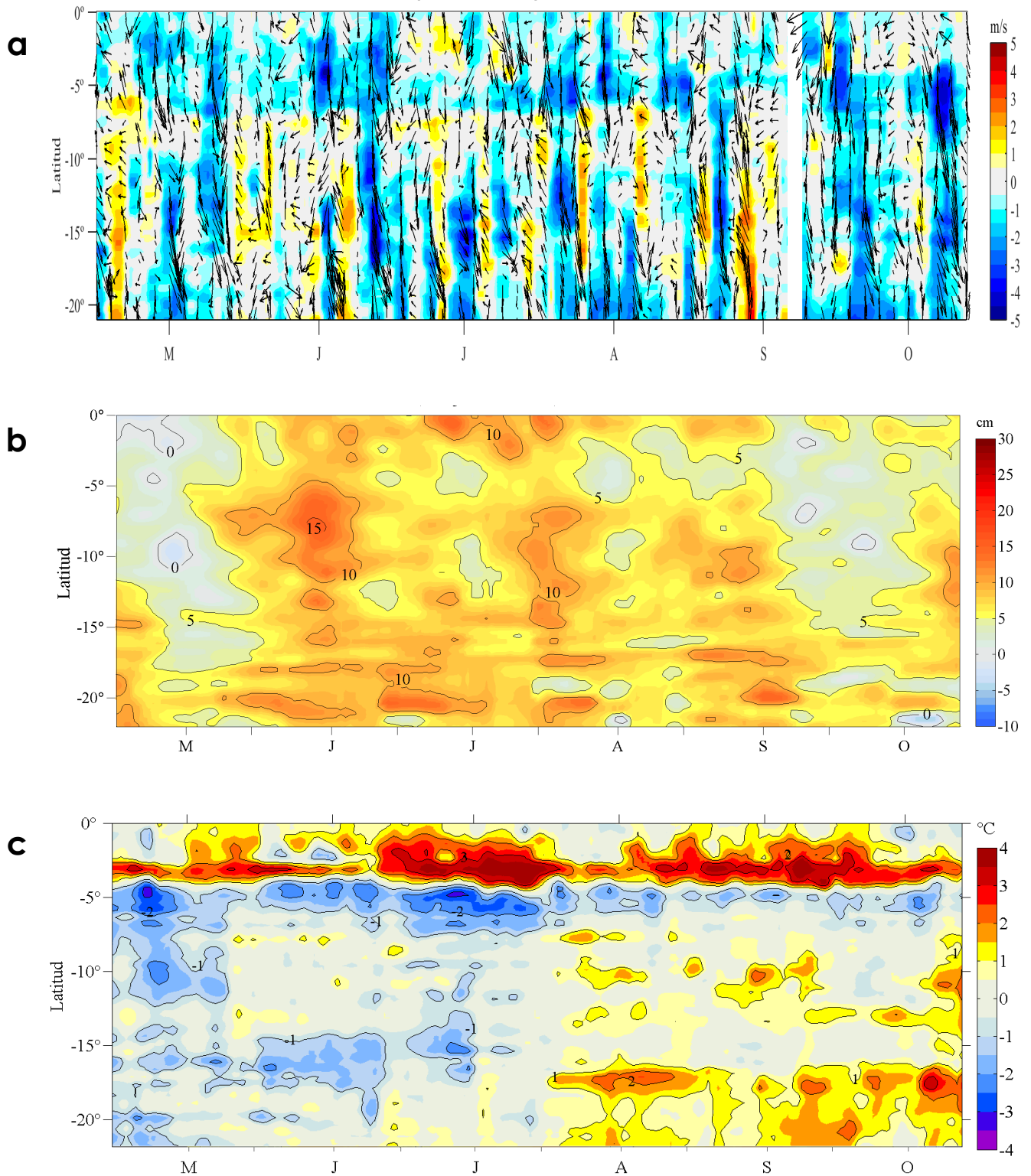
Figura 4. Evolución de las anomalías diarias de: a) velocidad del viento (m/s), b) nivel medio del mar (cm), c) temperatura superficial del mar (°C) para el último semestre actualizado al 13 de octubre de 2016. Datos: de IFREMER/CERSAT para (a), del Servicio de Monitoreo del Ambiente Marino Copernicus (CMEMS, según sus siglas en inglés) para (b) del satélite AVHRR v2 del Centro Nacional de Datos Climáticos de la Administración Nacional del Océano y la Atmósfera (NCDC/NOAA, según sus siglas en inglés) para (c). Las anomalías fueron calculadas para una franja de 100 km adyacente a la costa entre el ecuador y 21°S según los promedios climatológicos diarios de 2000-2014 para (a), de 1993-2013 para (b) y de 1982-2011 para (c). La barra de colores a la derecha muestra la escala de las anomalías en cada caso. Procesamiento: LHF/AFIOF/DGIOCC/IMARPE.
