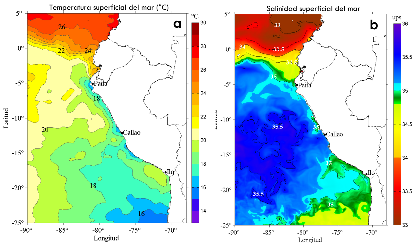
Figura 1. Distribución espacial promedio de: a) Temperatura Superficial del Mar (°C) y b) Salinidad Superficial del Mar, para la semana del 30 de setiembre al 06 de octubre de 2016 en el océano Pacífico tropical oriental. Datos: AVHRR v2 del Centro Nacional de Datos Climáticos de la Administración Nacional del Océano y la Atmósfera (NCDC/NOAA, según sus siglas en inglés) para (a) y del Hybrid Coordinate Ocean Model (HYCOM; Halliwell et al., 1998; 2000; Bleck, 2001) para (b). Las escalas de colores de la temperatura como de la salinidad superficial del mar se presentan a la derecha de cada gráfico. Procesamiento: LHFM/AFIOF/DGIOCC/IMARPE.
