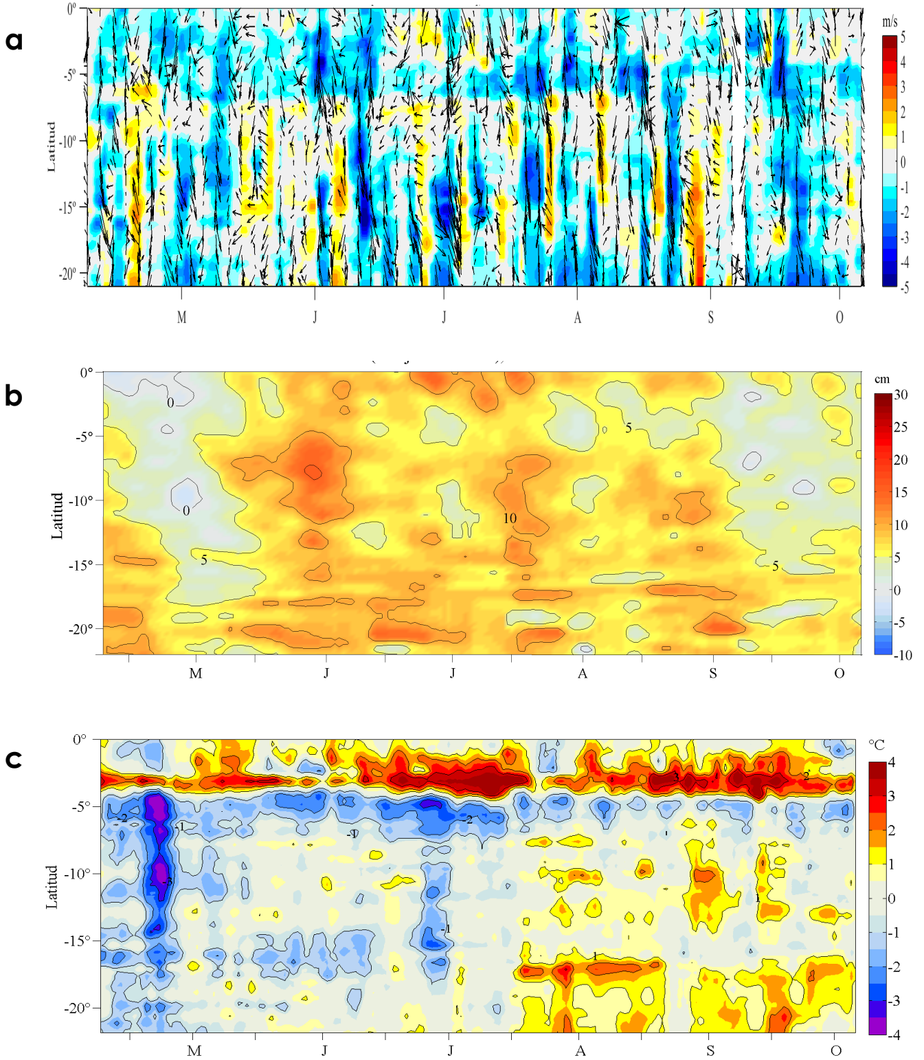
Figura 4. Evolución de las anomalías diarias de: a) velocidad del viento (m/s), b) nivel medio del mar (cm), c) temperatura superficial del mar (°C) para el último semestre actualizado al 06 de octubre de 2016. Datos: de IFREMER/CERSAT para (a), del Servicio de Monitoreo del Ambiente Marino Copernicus (CMEMS, según sus siglas en inglés) para (b) del satélite AVHRR v2 del Centro Nacional de Datos Climáticos de la Administración Nacional del Océano y la Atmósfera (NCDC/NOAA, según sus siglas en inglés) para (c). Las anomalías fueron calculadas para una franja de 100 km adyacente a la costa entre el ecuador y 21°S según los promedios climatológicos diarios de 2000-2014 para (a), de 1993-2013 para (b) y de 1982-2011 para (c). La barra de colores a la derecha muestra la escala de las anomalías en cada caso. Procesamiento: LHF/AFIOF/DGIOCC/IMARPE.
