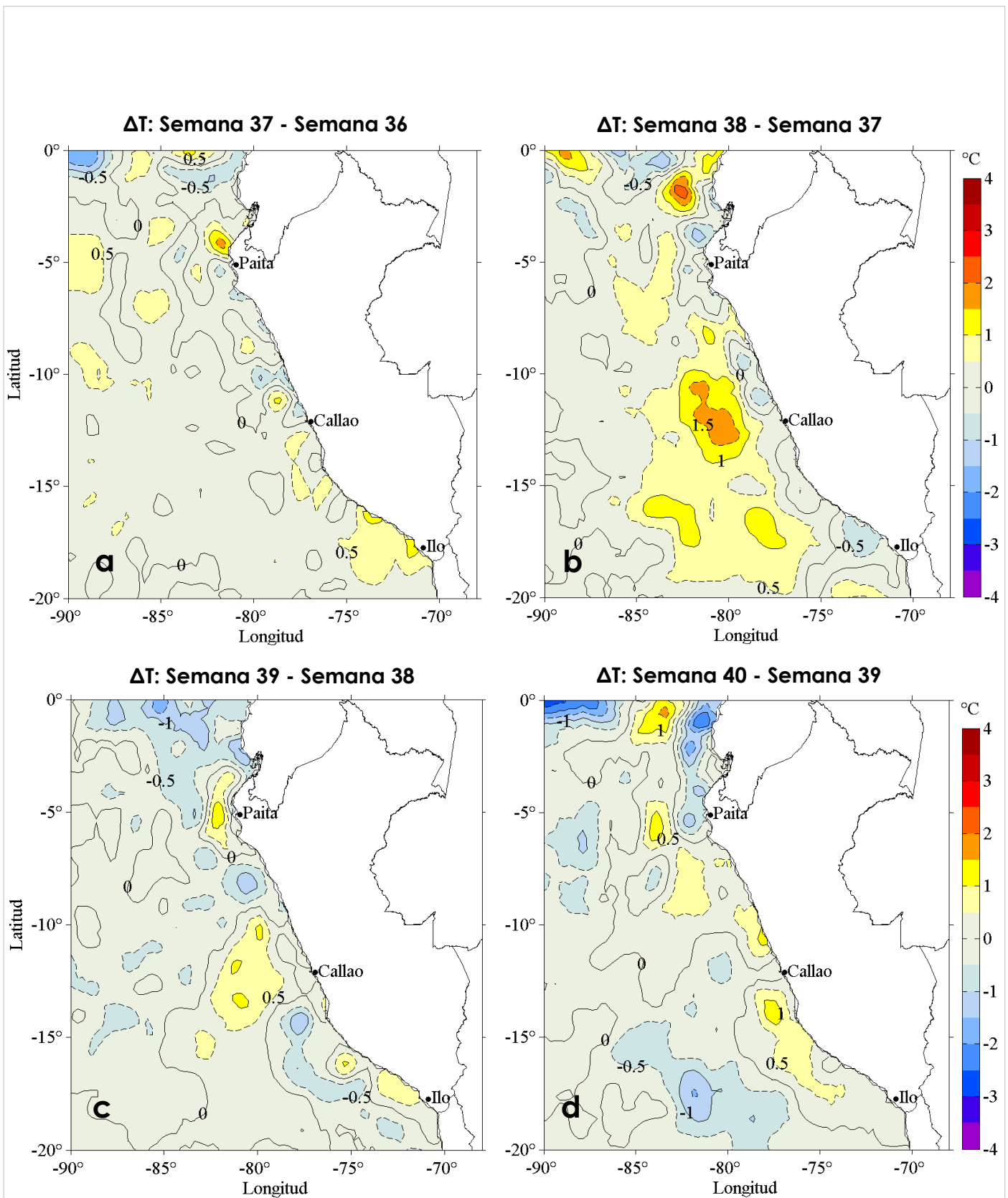
Figura 3. Variación semanal de la anomalía de la temperatura superficial del mar promedio (°C) en el océano Pacífico tropical oriental entre: a) la trigésimo séptima (09 - 15 de setiembre) y trigésimo sexta (02 - 08 de setiembre) semana, b) la trigésimo octava (16 - 22 de setiembre) y trigésimo séptima (09 - 15 de setiembre) semana, c) la trigésimo novena (23 - 29 de setiembre) y trigésimo octava (16 - 22 de setiembre) semana, y d) la cuadragésima (30 de setiembre - 06 de octubre) y trigésimo novena (23 - 29 de setiembre) semana del presente año. Los mapas, que indican el grado de calentamiento o enfriamiento de una semana a otra, provienen del sensor AVHRR v2 del Centro Nacional de Datos Climáticos de la Administración Nacional del Océano y la Atmósfera (NCDC/NOAA, según sus siglas en inglés). Las anomalías térmicas se calcularon de acuerdo con la climatología para el período 1982-2011. La barra de colores de las anomalías térmicas se presenta a la derecha. Procesamiento: LHF/AFIOF/DGIOCC/IMARPE.
