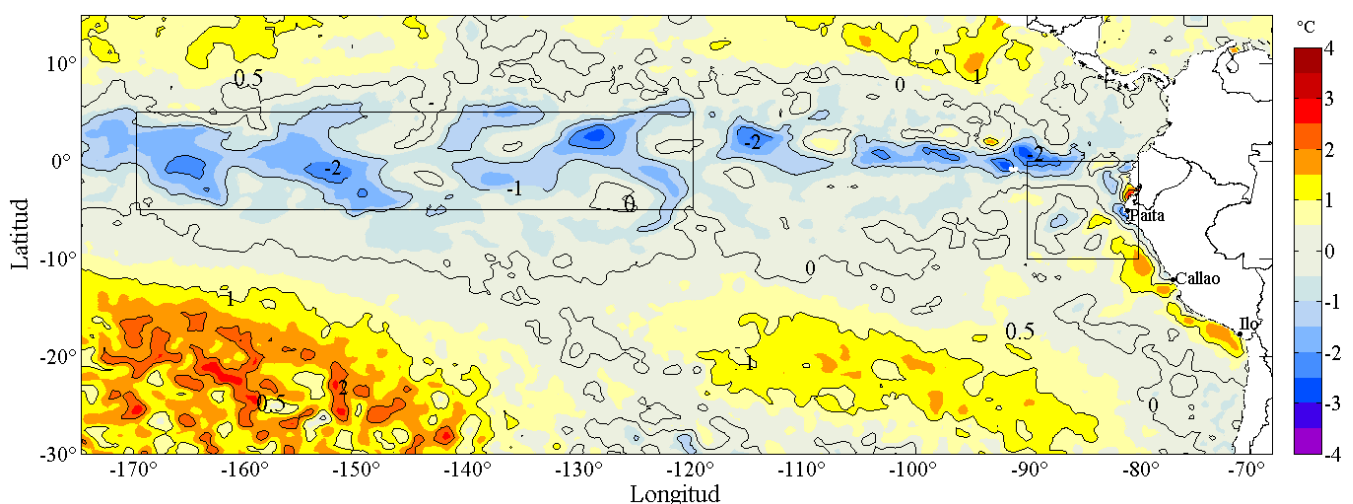
Figura 2. Anomalías promedio de la temperatura superficial del mar (°C) en el océano Pacífico tropical para la semana del 30 de setiembre al 06 de octubre de 2016. Las regiones Niño 3.4 y Niño 1+2 en los sectores central y oriental del océano, respectivamente, están delimitadas con una línea de color gris. Datos: AVHRR Global Reyn_SmithOIv2R (Reynolds, et. al., 2007) de CMB/EMC/NCEP de la Administración Nacional del Océano y la Atmósfera (NOAA, según sus siglas en inglés). Las anomalías se calcularon con respecto de la climatología para el período 1982-2011. Procesamiento: IMARPE.
