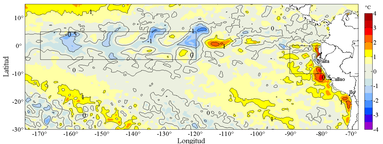
Figura 2. Anomalías promedio de la temperatura superficial del mar (°C) en el océano Pacífico tropical para la semana del 16 al 22 de setiembre de 2016. Las regiones Niño 3.4 y Niño 1+2 en los sectores central y oriental del océano, respectivamente, están delimitadas con una línea de color gris. Datos: AVHRR Global Reyn_SmithOlv2R (Reynolds, et al., 2007) de CMB/EMC/NCEP de la Administración Nacional del Océano y la Atmósfera (NOAA, según sus siglas en inglés). Las anomalías se calcularon con respecto de la climatología para el período 1982-2011. Procesamiento: IMARPE.
