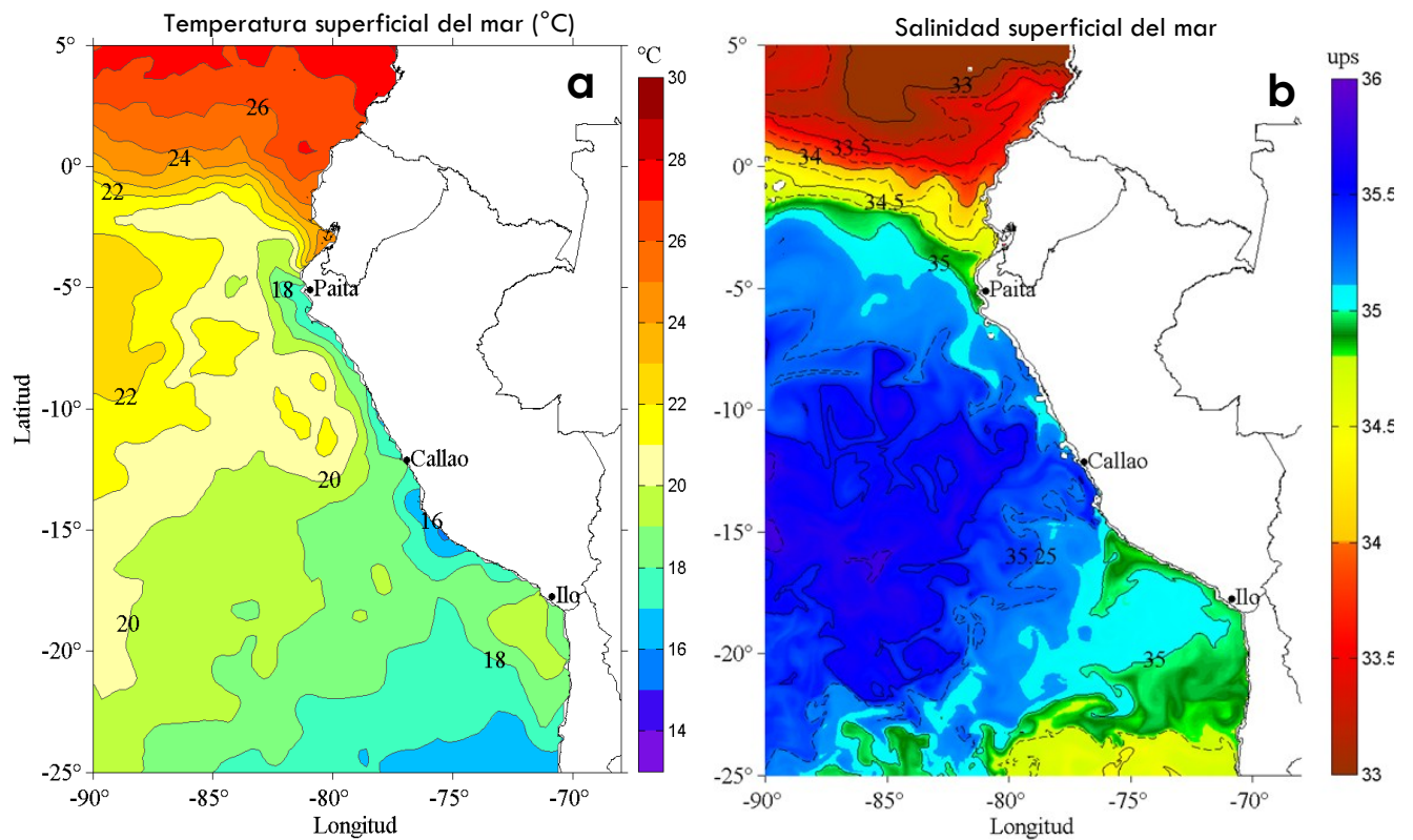
Figura 1. Distribución espacial promedio de: a) Temperatura Superficial del Mar (°C) y b) Salinidad Superficial del Mar, para la semana del 16 al 22 de setiembre de 2016 en el océano Pacífico tropical oriental. Datos: AVHRR v2 del Centro Nacional de Datos Climáticos de la Administración Nacional del Océano y la Atmósfera (NCDC/NOAA, según sus siglas en inglés) para (a) y del HYbrid Coordinate Ocean Model (HYCOM; Halliwell et al., 1998; 2000; Bleck, 2001) para (b). Las escalas de colores de la temperatura como de la salinidad superficial del mar se presentan a la derecha de cada gráfico. Procesamiento: LHFH/AFIOF/DGIOCC/IMARPE.
