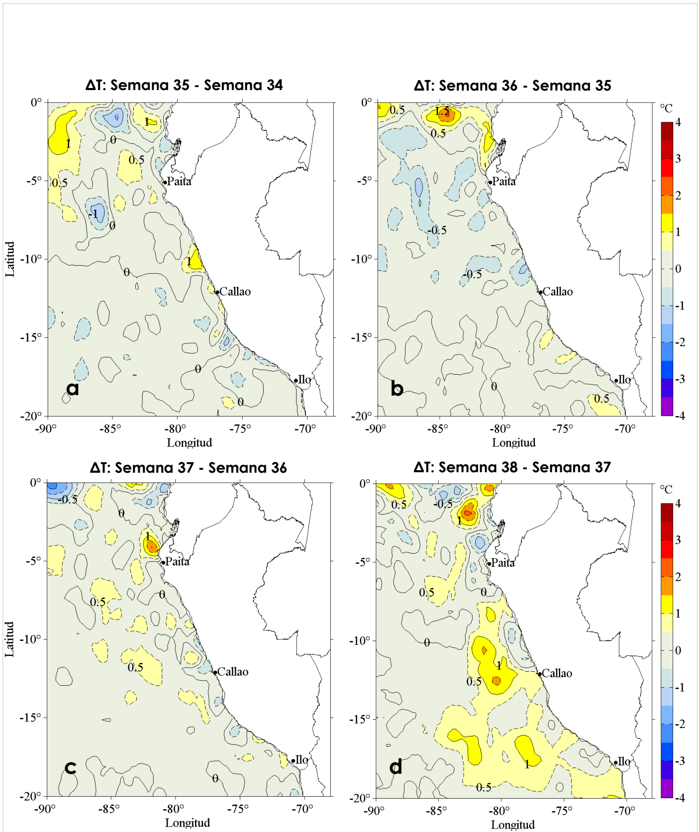
Figura 3. Variación semanal de la anomalía de la temperatura superficial del mar promedio (°C) en el océano Pacífico tropical oriental entre: a) la trigésimo quinta (26 de agosto - 01 de setiembre) y trigésimo cuarta (19 - 25 de agosto) semana, b) la trigésimo sexta (02 - 08 de setiembre) y trigésimo quinta (26 de agosto - 01 de setiembre) semana, c) la trigésimo séptima (9 - 15 de setiembre) y trigésimo sexta (02 - 08 de setiembre) semana, y d) la trigésimo octava (16 - 22 de setiembre) y trigésimo séptima (09 - 15 de setiembre) semana del presente año. Los mapas, que indican el grado de calentamiento o enfriamiento de una semana a otra, provienen del sensor AVHRR v2 del Centro Nacional de Datos Climáticos de la Administración Nacional del Océano y la Atmósfera (NCDC/NOAA, según sus siglas en inglés). Las anomalías térmicas se calcularon de acuerdo con la climatología para el período 1982-2011. La barra de colores de las anomalías térmicas se presenta a la derecha. Procesamiento: LHFM/AFIOF/DGIOCC/IMARPE.
