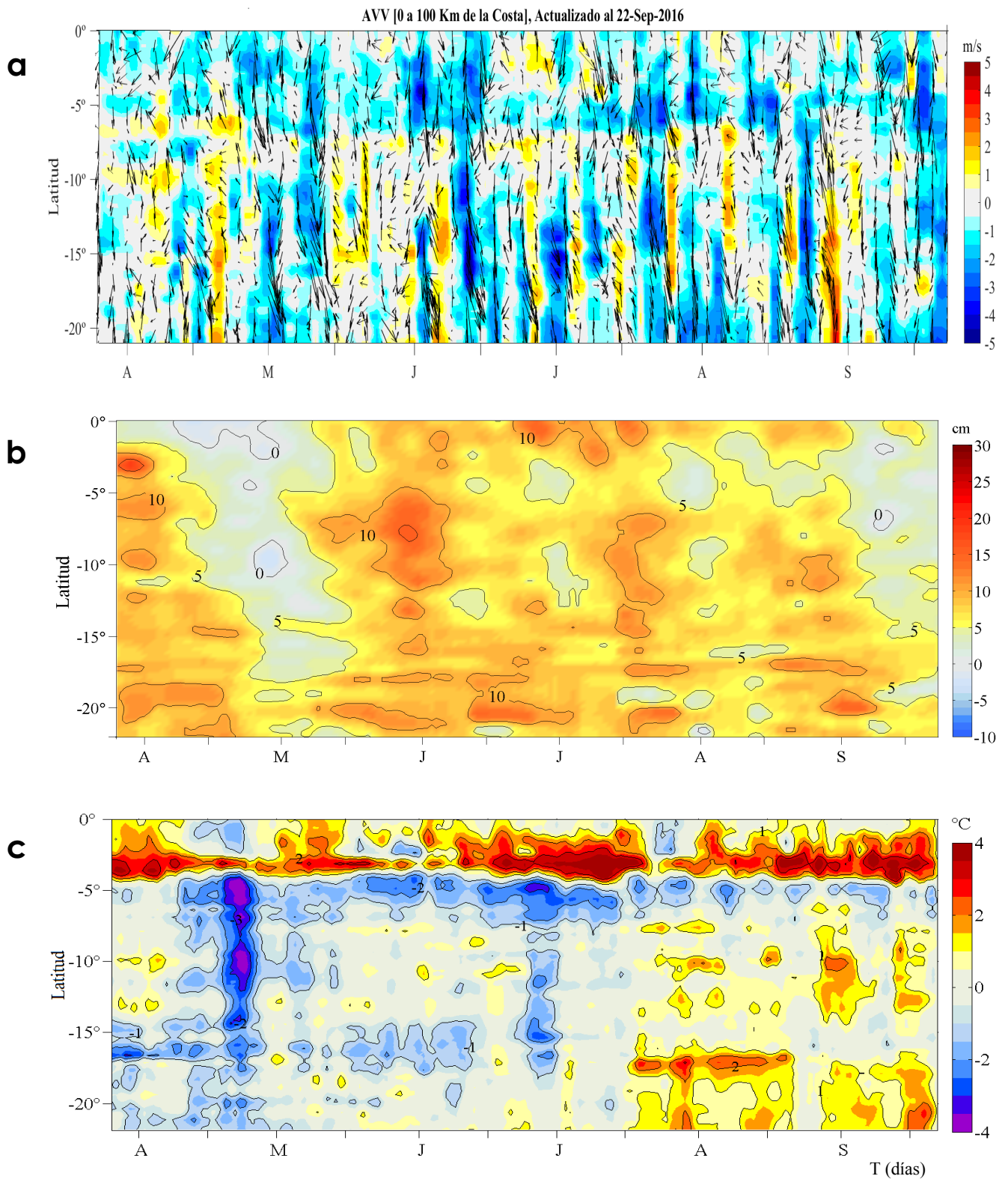
Figura 4. Evolución de las anomalías diarias de: a) velocidad del viento (m/s), b) nivel medio del mar (cm), c) temperatura superficial del mar (°C) para el último semestre actualizado al 22 de setiembre. Datos: de IFREMER/CERSAT para (a), del Servicio de Monitoreo del Ambiente Marino Copernicus (CMEMS, según sus siglas en inglés) para (b) del satélite AVHRR v2 del Centro Nacional de Datos Climáticos de la Administración Nacional del Océano y la Atmósfera (NCDC/NOAA, según sus siglas en inglés) para (c). Las anomalías fueron calculadas para una franja de 100 km adyacente a la costa entre el ecuador y 21°S según los promedios climatológicos diarios de 2000-2014 para (a), de 1993-2013 para (b) y de 1982-2011 para (c). La barra de colores a la derecha muestra la escala de las anomalías en cada caso. Procesamiento: LHF/AFIOF/DGIOCC/IMARPE.
