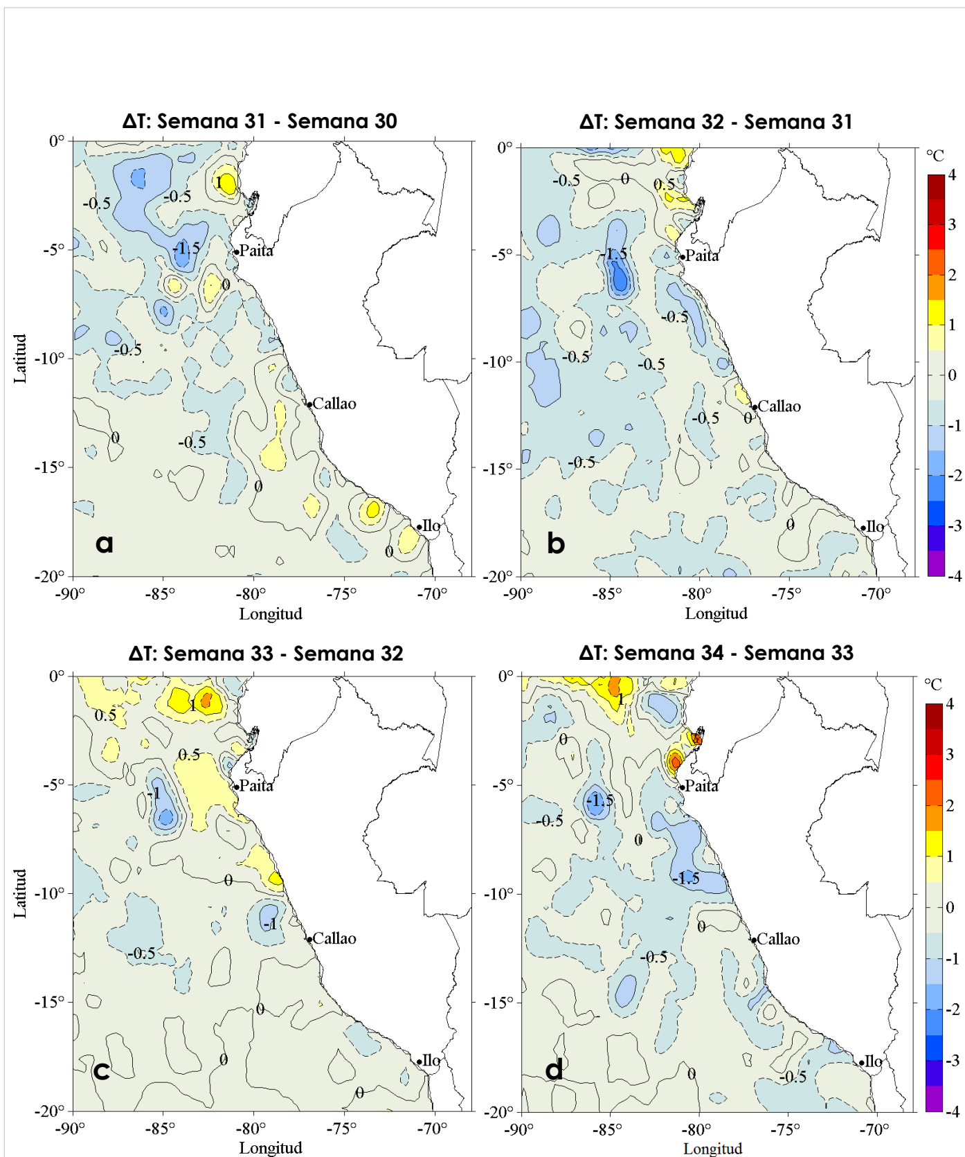
Figura 3. Variación semanal de la anomalía de la temperatura superficial del mar promedio (°C) en el océano Pacífico tropical oriental entre: a) la trigésimo primera (29 de julio - 04 de agosto) y trigésima (22 - 28 de julio) semana, b) la trigésimo segunda (05 - 11 de agosto) y trigésima primera (29 de julio - 04 de agosto) semana, c) la trigésimo tercera (12 - 18 de agosto) y trigésima segunda (05 - 11 de agosto) semana, y d) la trigésimo cuarta (19 - 25 de agosto) y trigésima tercera (12 - 18 de agosto) semana del presente año. Los mapas, que indican el grado de calentamiento o enfriamiento de una semana a otra, provienen del sensor AVHRR v2 del Centro Nacional de Datos Climáticos de la Administración Nacional del Océano y la Atmósfera (NCDC/NOAA, según sus siglas en inglés). Las anomalías térmicas se calcularon de acuerdo con la climatología para el período 1982-2011. La barra de colores de las anomalías térmicas se presenta a la derecha. Procesamiento: LHF/M/AFIOF/DGIOCC/IMARPE.
