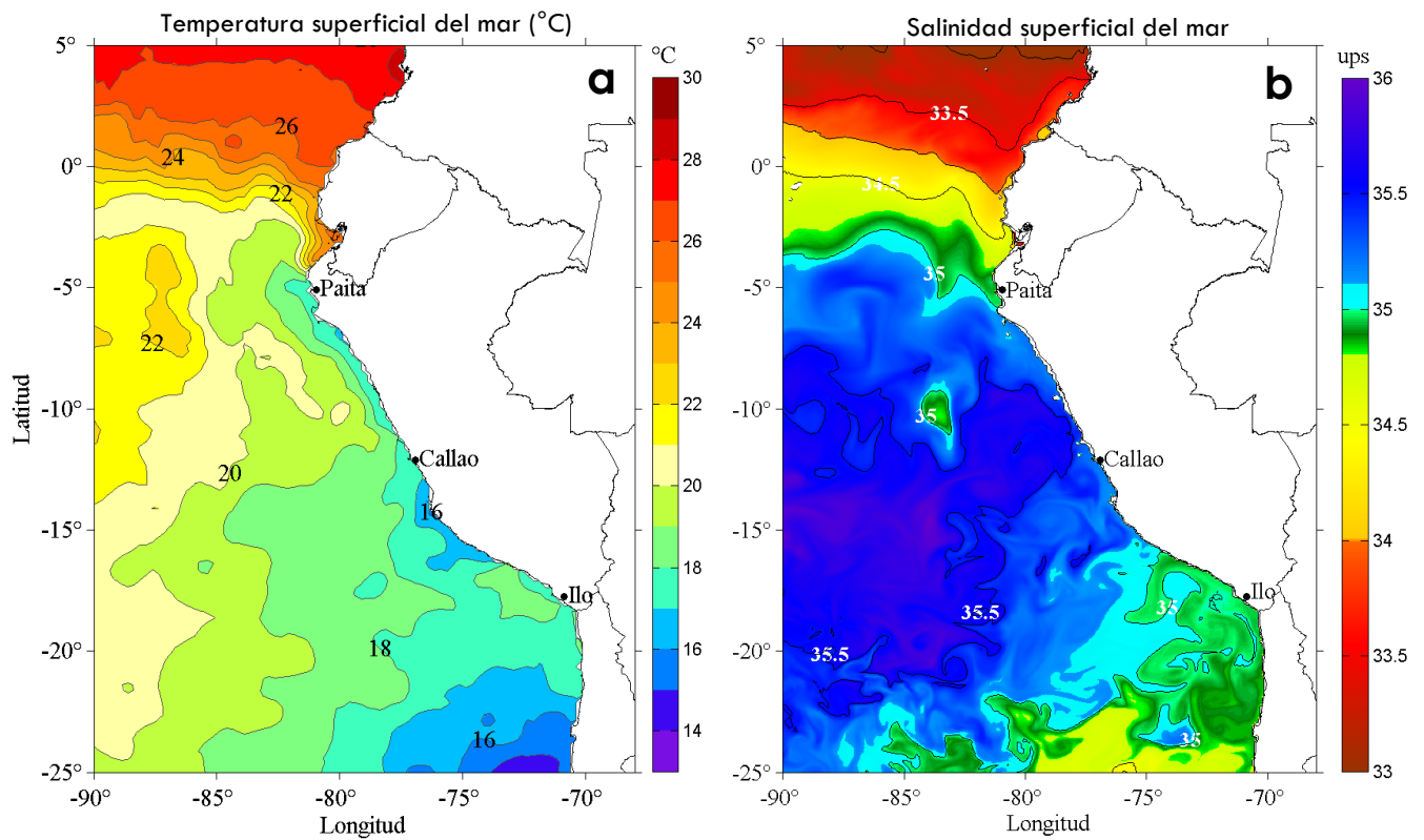
Figura 1. Distribución espacial promedio de: a) Temperatura Superficial del Mar (°C) y b) Salinidad Superficial del Mar, para la semana del 19 al 25 de agosto de 2016 en el océano Pacífico tropical oriental. Datos: AVHRR v2 del Centro Nacional de Datos Climáticos de la Administración Nacional del Océano y la Atmósfera (NCDC/NOAA, según sus siglas en inglés) para (a) y del Hybrid Coordinate Ocean Model (HYCOM; Halliwell et al., 1998; 2000; Bleck, 2001) para (b). Las escalas de colores de la temperatura como de la salinidad superficial del mar se presentan a la derecha de cada gráfico. Procesamiento: LHFM/AFIOF/DGIOCC/IMARPE.
