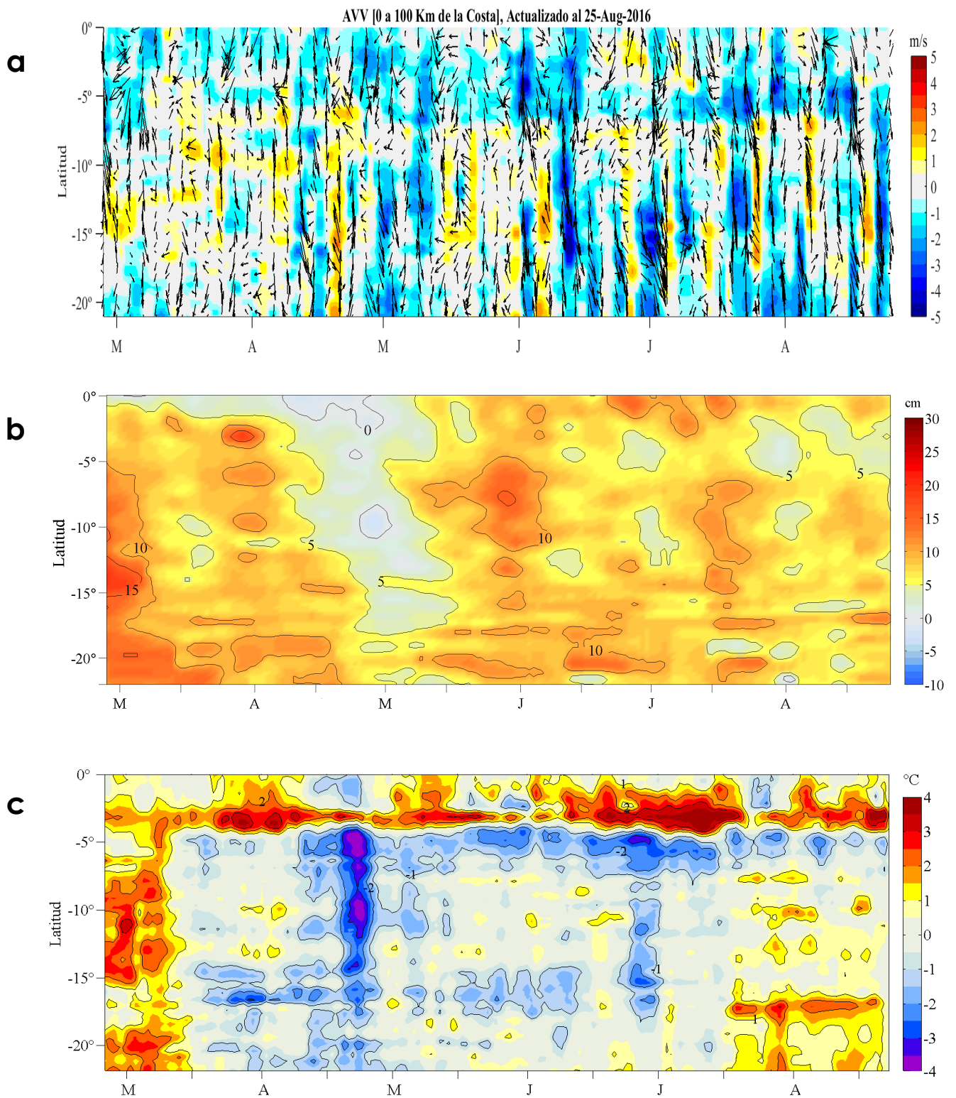
Figura 4. Evolución de las anomalías diarias de: a) velocidad del viento (m/s), b) nivel medio del mar (cm), c) temperatura superficial del mar (°C) para el último semestre actualizado al 25 de agosto de 2016. Datos: de IFREMER/CERSAT para (a), del Servicio de Monitoreo del Ambiente Marino Copernicus (CMEMS, según sus siglas en inglés) para (b) del satélite AVHRR v2 del Centro Nacional de Datos Climáticos de la Administración Nacional del Océano y la Atmósfera (NCDC/NOAA, según sus siglas en inglés) para (c). Las anomalías fueron calculadas para una franja de 100 km adyacente a la costa entre el ecuador y 21°S según los promedios climatológicos diarios de 2000-2014 para (a), de 1993-2013 para (b) y de 1982-2011 para (c). La barra de colores a la derecha muestra la escala de las anomalías en cada caso. Procesamiento: LHF/AFIOF/DGIOCC/IMARPE.
