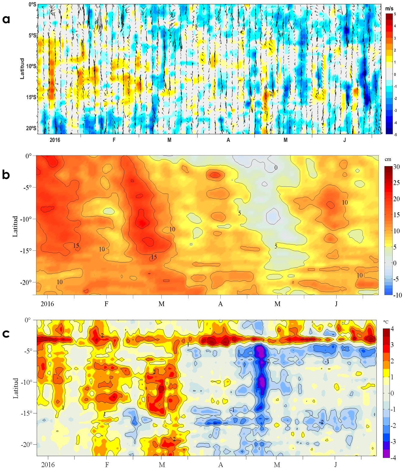
Figura 4. Evolución de las anomalías diarias de: a) velocidad del viento (m/s), b) nivel medio del mar (cm), c) temperatura superficial del mar (°C) para el último semestre actualizado al 23 de junio de 2016. Datos: de IFREMER/CERSAT para (a), del Servicio de Monitoreo del Ambiente Marino Copernicus (CMEMS, según sus siglas en inglés) para (b) del satélite AVHRR v2 del Centro Nacional de Datos Climáticos de la Administración Nacional del Océano y la Atmósfera (NCDC/NOAA, según sus siglas en inglés) para (c). Las anomalías fueron calculadas para una franja de 100 km adyacente a la costa entre el ecuador y 21°S según los promedios climatológicos diarios de 2000-2014 para (a), de 1993-2013 para (b) y de 1982-2011 para (c). La barra de colores a la derecha muestra la escala de las anomalías en cada caso. Procesamiento: LHF/AFIOF/DGIOCC/IMARPE.
