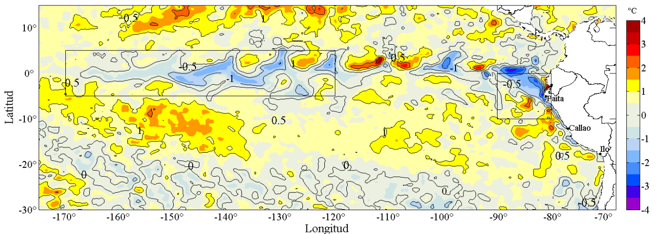
Figura 1. Anomalías promedio de la temperatura superficial del mar (°C) en el océano Pacífico tropical para la semana del 17 al 23 de junio de 2016. Las regiones Niño 3.4 y Niño 1+2 en los sectores central y oriental del océano, respectivamente, están delimitadas con una línea de color gris. Datos: AVHRR Global Reyn_SmithOiv2R (Reynolds, et. al., 2007) de CMB/EMC/NCEP de la Administración Nacional del Océano y la Atmósfera (NOAA, según sus siglas en inglés). Las anomalías se calcularon con respecto de la climatología para el período 1982-2011. Procesamiento: IMARPE.
