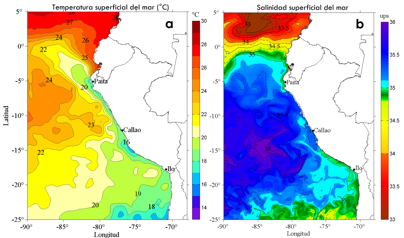
Figura 2. Distribución espacial promedio de: a) Temperatura Superficial del Mar (°C) y b) Salinidad Superficial del Mar, para la semana del 17 al 23 de junio de 2016 en el océano Pacífico tropical oriental. Datos: AVHRR v2 del Centro Nacional de Datos Climáticos de la Administración Nacional del Océano y la Atmósfera (NCDC/NOAA, según sus siglas en inglés) para (a) y del HYbrid Coordinate Ocean Model (HYCOM; Halliwell et al., 1998; 2000; Bleck, 2001) para (b). Las escalas de colores de la temperatura como de la salinidad superficial del mar se presentan a la derecha de cada gráfico. Procesamiento: LHFH/AFIOF/DGIOCC/IMARPE.
