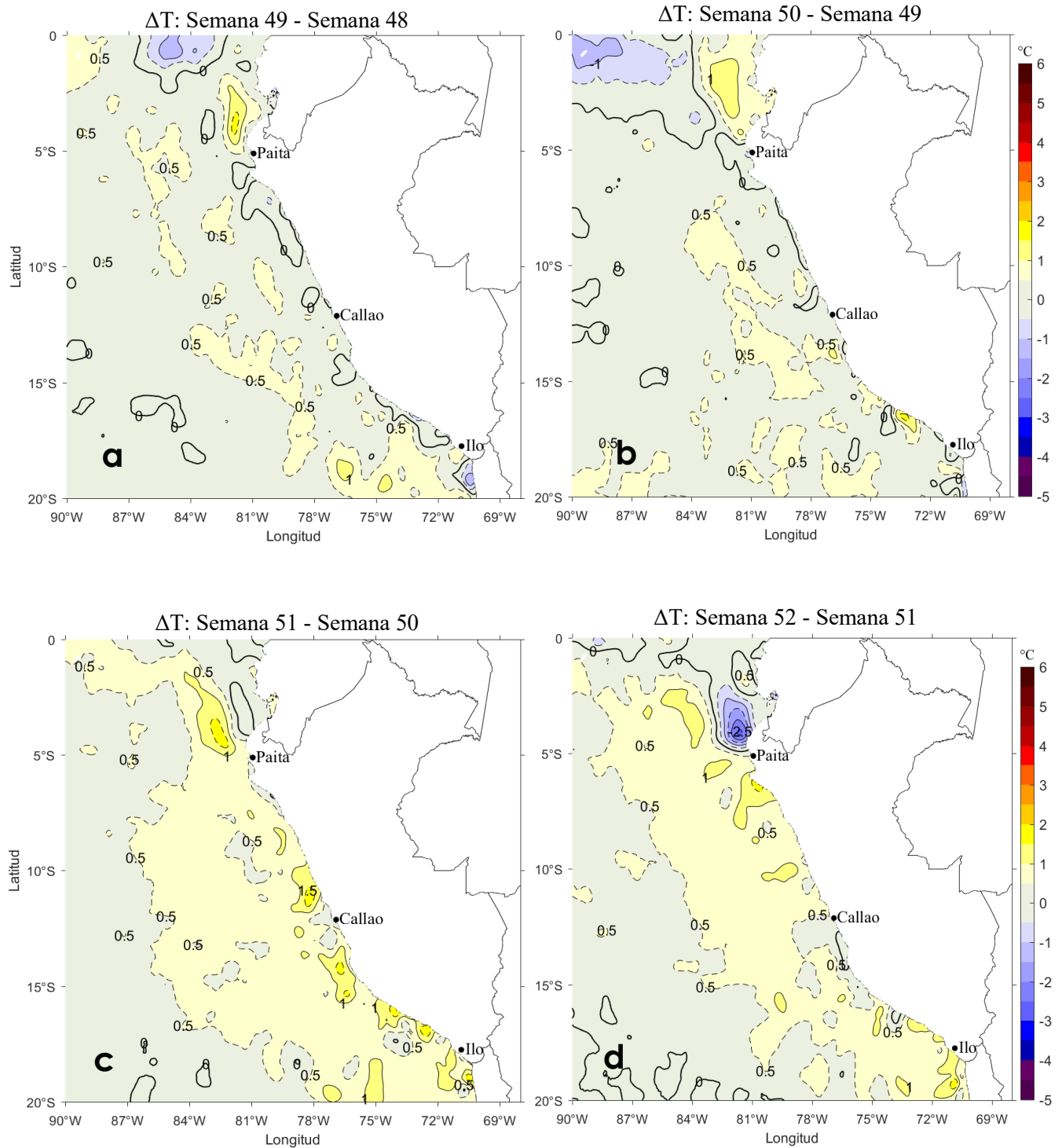
Figura 3. Variación semanal de la temperatura superficial del mar promedio ( ^{\circ}\text{C} ) en el océano Pacífico tropical oriental entre: a) cuadragésimo novena (03-09 de diciembre) y cuadragésimo octava (26 de noviembre-02 de diciembre) semana, b) quincuagésima (10-16 de diciembre) y cuadragésimo novena (03-09 de diciembre) semana, c) quincuagésima primera (17-23 de diciembre) y quincuagésima (10-16 de diciembre) semana, y d) quincuagésima segunda (24-30 de diciembre) y quincuagésima primera (17-23 de diciembre) semana del presente año.
