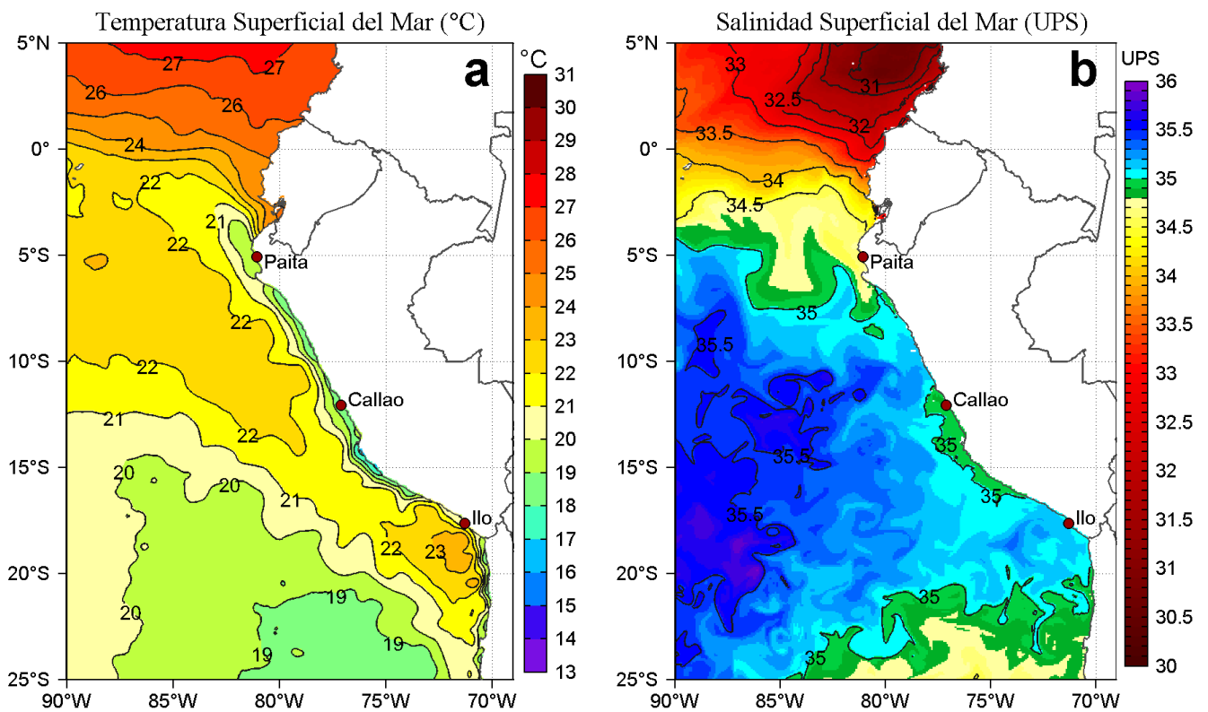
Figura 1. Distribución espacial promedio de: a) Temperatura Superficial del Mar (°C) y b) Salinidad Superficial del Mar, para la semana del 24 al 30 de diciembre de 2017 en el océano Pacífico tropical oriental. Datos: OSTIA-UKMO-L4-GLOB-v2.0 (UK Met Office, 2012; Donlon et al, 2012) disponible en https://podaac.jpl.nasa.gov/dataset/OSTIA-UKMO-L4-GLOB-v2.0 ) para (a) y del Hybrid Coordinate Ocean Model (HYCOM; Halliwell et al., 1998; 2000; Bleck, 2001) para (b). Las escalas de colores de la temperatura como de la salinidad superficial del mar se presentan a la derecha de cada gráfico. Procesamiento: LHF/AFIOF/DGIOCC/IMARPE.
