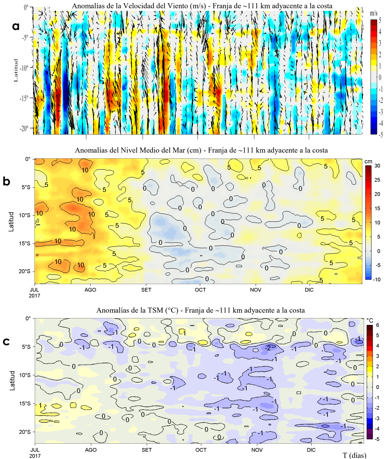
Figura 4. Evolución de las anomalías diarias de: a) velocidad del viento (m/s), b) nivel medio del mar (cm), c) temperatura superficial del mar (°C) para el último semestre actualizado al 30 de diciembre de 2017. Datos: de IFREMER/CERSAT para (a), del Servicio de Monitoreo del Ambiente Marino Copernicus (CMEMS, según sus siglas en inglés) para (b), de OSTIA-UKMO-L4-GLOB-v2.0 para (c). Las anomalías fueron calculadas para una franja de 111 km adyacente a la costa entre el ecuador y 22°S según los promedios climatológicos diarios de 2000-2014 para (a), de 1993-2013 para (b) y de 2007-2016 para (c). La barra de colores a la derecha muestra la escala de las anomalías en cada caso. Procesamiento: LHFm/AFIOF/DGIOCC/IMARPE.
