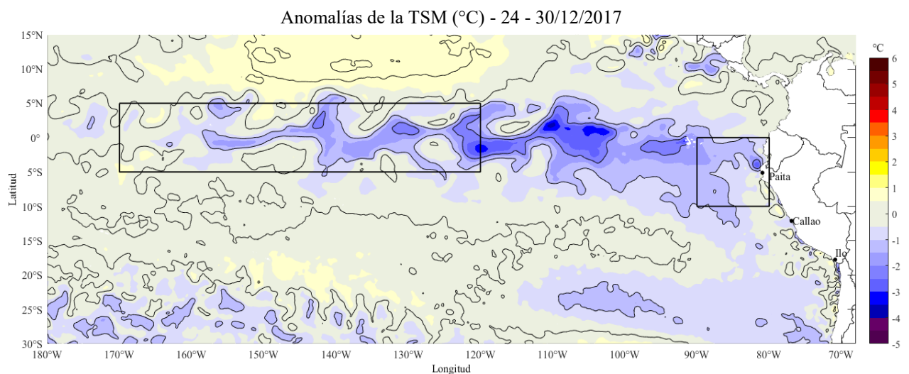
Figura 2. Anomalías promedio de la temperatura superficial del mar (°C) en el océano Pacífico tropical para la semana del 24 al 30 de diciembre de 2017. Las regiones Niño 3.4 y Niño 1+2 en los sectores central y oriental del océano, respectivamente, están delimitadas con una línea de color gris. Datos: OSTIA-UKMO-L4-GLOB-v2.0 (UK Met Office, 2012; Donlon et al, 2012) disponible en https://podaac.jpl.nasa.gov/dataset/OSTIA-UKMO-L4-GLOB-v2.0 ). Las anomalías se calcularon con respecto de la climatología para el período 2007-2016. Procesamiento: IMARPE.
