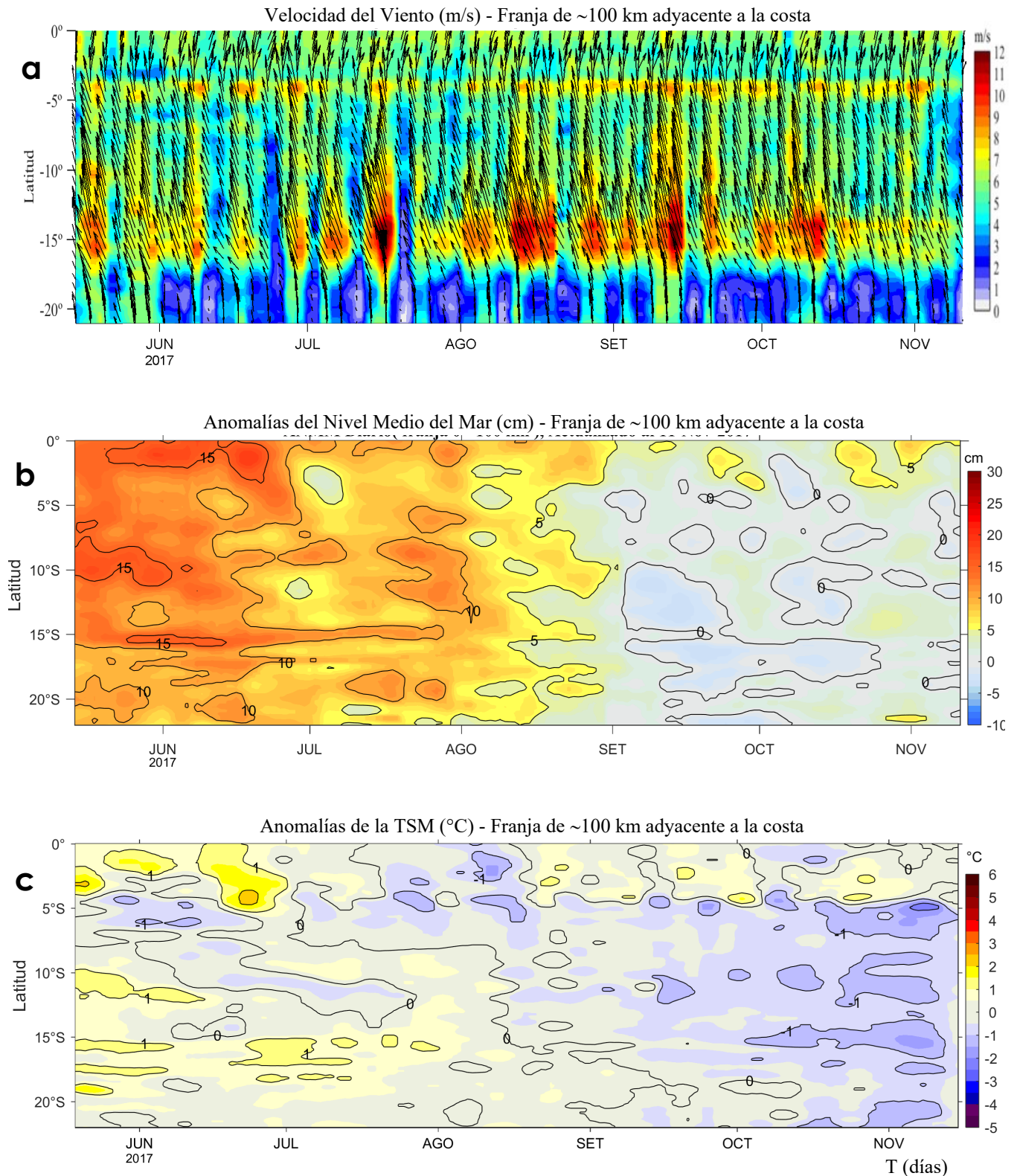
Figura 4. Evolución de: a) Velocidad del viento (m/s), b) de la anomalía del nivel medio del mar (cm), c) de la anomalía de la temperatura superficial del mar (°C) para el último semestre actualizado al 11 de noviembre de 2017. Datos: de IFREMER/CERSAT para (a), del Servicio de Monitoreo del Ambiente Marino Copernicus (CMEMS en inglés) para (b), de OSTIA-UKMO-L4-GLOB-v2.0 para (c). Las anomalías fueron calculadas para una franja de 100 km adyacente a la costa entre el ecuador y 22°S según los promedios climatológicos diarios de 2000-2014 para (a), de 1993-2013 para (b) y de 2007-2016 para (c). La barra de colores a la derecha muestra la escala de las anomalías en cada caso. Procesamiento: LHF/AFIOF/DGIOCC/IMARPE.
