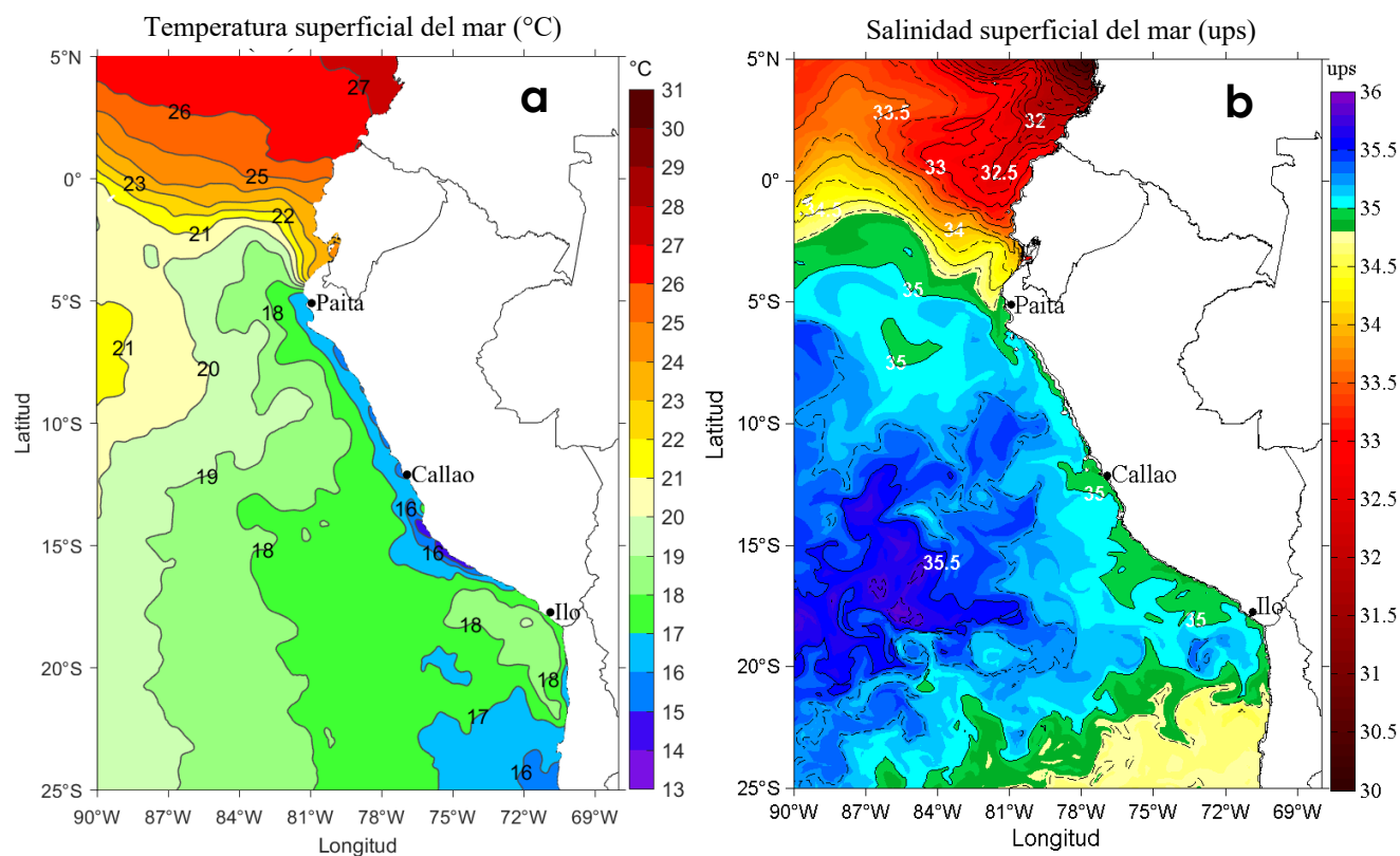
Figura 1. Distribución espacial promedio de: a) Temperatura Superficial del Mar (°C) para la semana del 05 al 11 de noviembre de 2017 y b) Salinidad Superficial del Mar (UPS) para la semana del 29 de octubre al 04 de noviembre en el océano Pacífico tropical oriental. Datos: OSTIA-UKMO-L4-GLOB-v2.0 (UK Met Office, 2012; Donlon et al, 2012) disponible en https://podaac.jpl.nasa.gov/dataset/OSTIA-UKMO-L4-GLOB-v2.0 para (a) y del Hybrid Coordinate Ocean Model (HYCOM; Halliwell et al., 1998; 2000; Bleck, 2001) para (b). Las escalas de colores de la temperatura como de la salinidad superficial del mar se presentan a la derecha de cada gráfico. Procesamiento: LHFM/AFIOF/DGIOCC/IMARPE.
