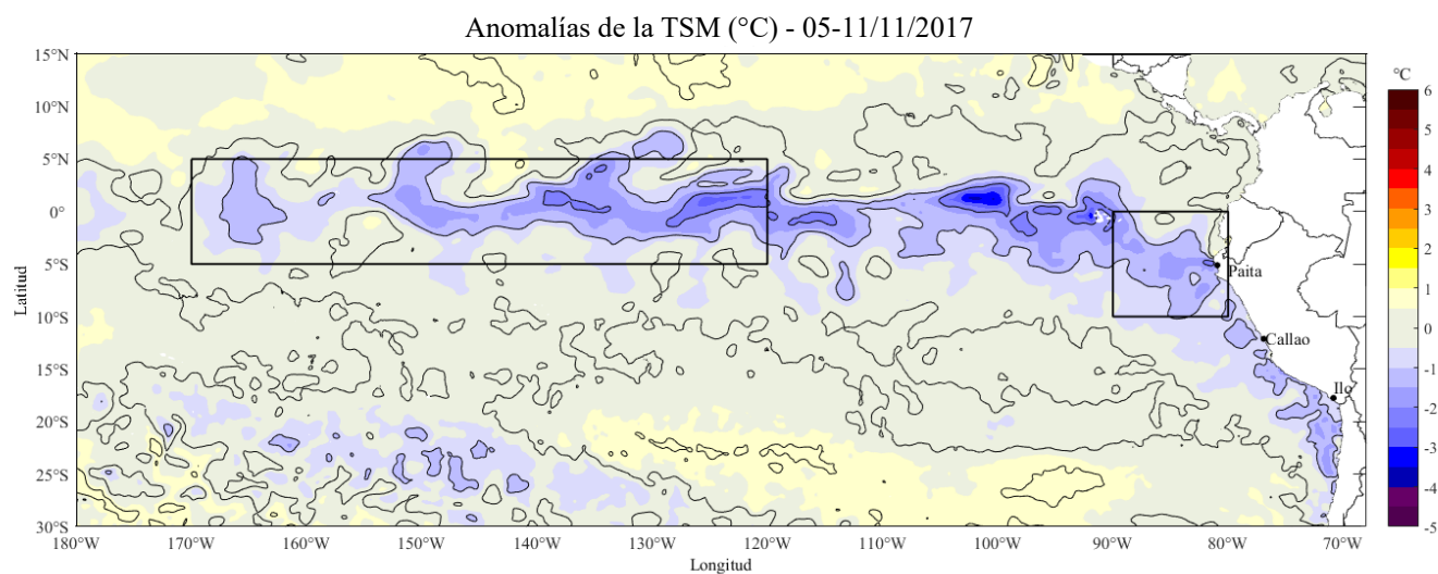
Figura 2. Anomalías promedio de la temperatura superficial del mar (°C) en el océano Pacífico tropical para la semana del 05 al 11 de noviembre de 2017. Las regiones Niño 3.4 y Niño 1+2 en los sectores central y oriental del océano, respectivamente, están delimitadas con una línea de color gris. Datos: OSTIA-UKMO-L4-GLOB-v2.0 (UK Met Office, 2012; Donlon et al, 2012) disponible en https://podaac.jpl.nasa.gov/dataset/OSTIA-UKMO-L4-GLOB-v2.0 ). Las anomalías se calcularon con respecto de la climatología para el período 2007-2016. Procesamiento: IMARPE.
