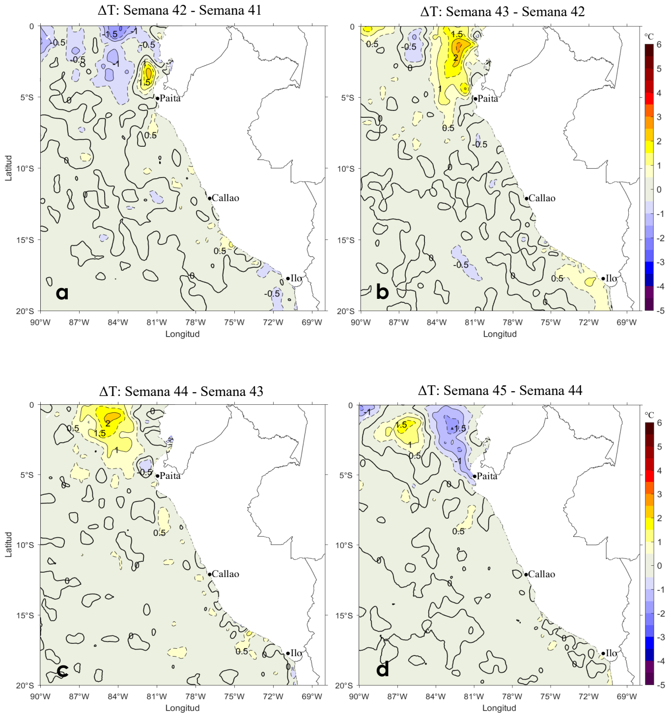
Figura 3. Variación semanal de la temperatura superficial del mar promedio ( ^{\circ}\text{C} ) en el océano Pacífico tropical oriental entre: a) cuadragésimo segunda (15-21 de octubre) y cuadragésimo primera (08-14 de octubre) semana, b) cuadragésimo tercera (22-28 de octubre) y cuadragésimo segunda (15-21 de octubre) semana, c) cuadragésimo cuarta (29 de octubre-04 de noviembre) y cuadragésimo tercera (22-28 de octubre) semana, y d) cuadragésimo quinta (05 -11 de noviembre) y cuadragésimo cuarta (29 de octubre-04 de noviembre) semana del presente año.
