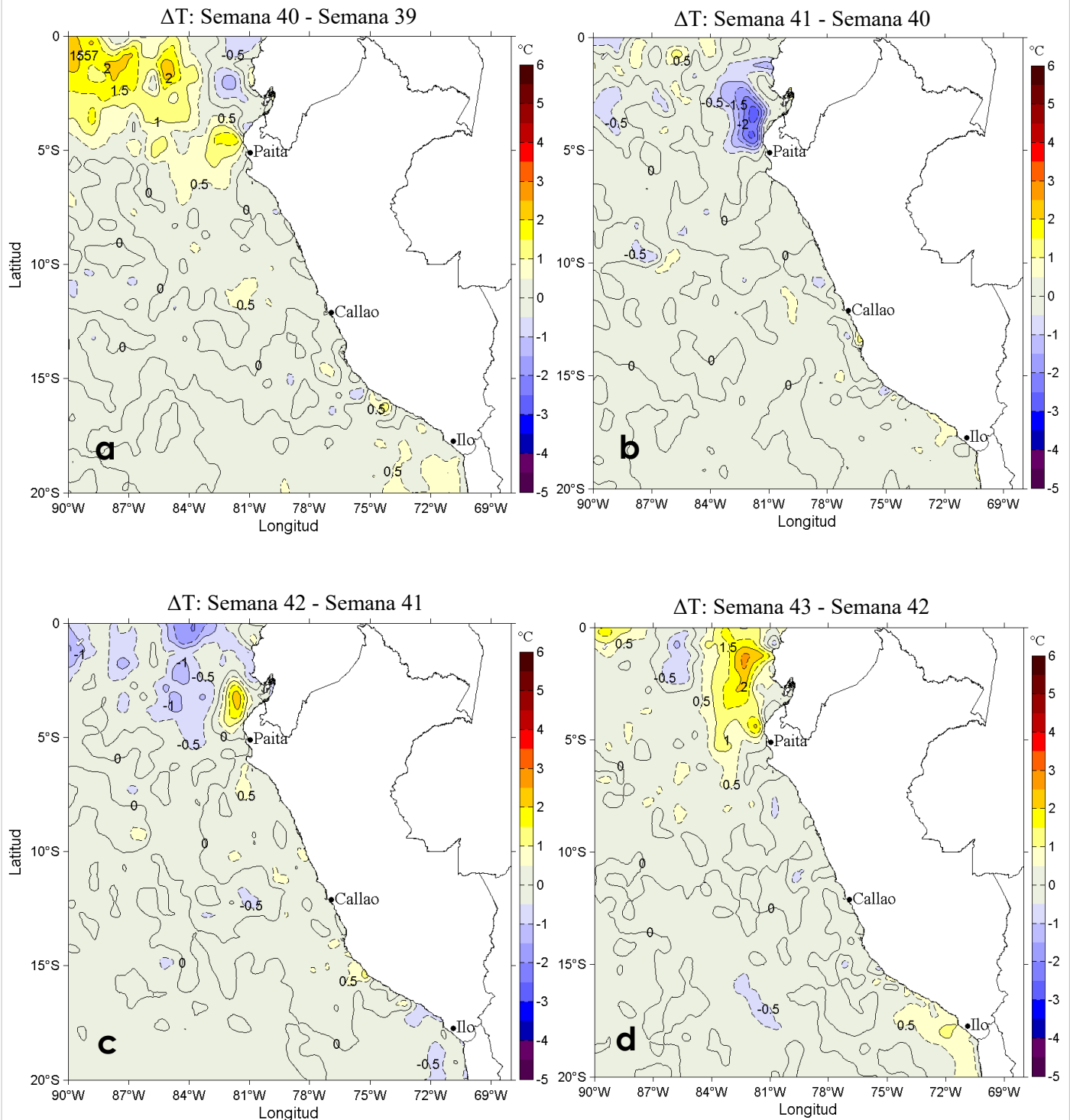
Figura 3. Variación semanal de la temperatura superficial del mar ( ^{\circ}\text{C} ) en el océano Pacífico tropical oriental entre: a) cuadragésima (01-07 de octubre) y trigésimo novena (24-30 de setiembre) semana, b) cuadragésimo primera (08-14 de octubre) y cuadragésima (01-07 de octubre) semana, c) cuadragésimo segunda (15-21 de octubre) y cuadragésimo primera (08-14 de octubre) semana, y d) cuadragésimo segunda (22-28 de octubre) y cuadragésimo primera (15-21 de octubre) semana del presente año.
