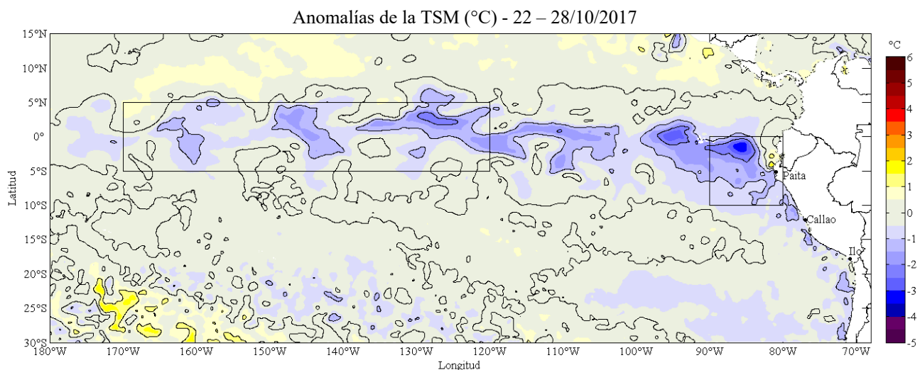
Figura 2. Anomalías promedio de la temperatura superficial del mar (°C) en el océano Pacífico tropical para la semana del 22 al 28 de octubre de 2017. Las regiones Niño 3.4 y Niño 1+2 en los sectores central y oriental del océano, respectivamente, están delimitadas con una línea de color gris. Datos: OSTIA-UKMO-L4-GLOB-v2.0 (UK Met Office, 2012; Donlon et al, 2012) disponible en https://podaac.jpl.nasa.gov/dataset/OSTIA-UKMO-L4-GLOB-v2.0 ). Las anomalías se calcularon con respecto de la climatología para el período 2007-2016. Procesamiento: IMARPE.
