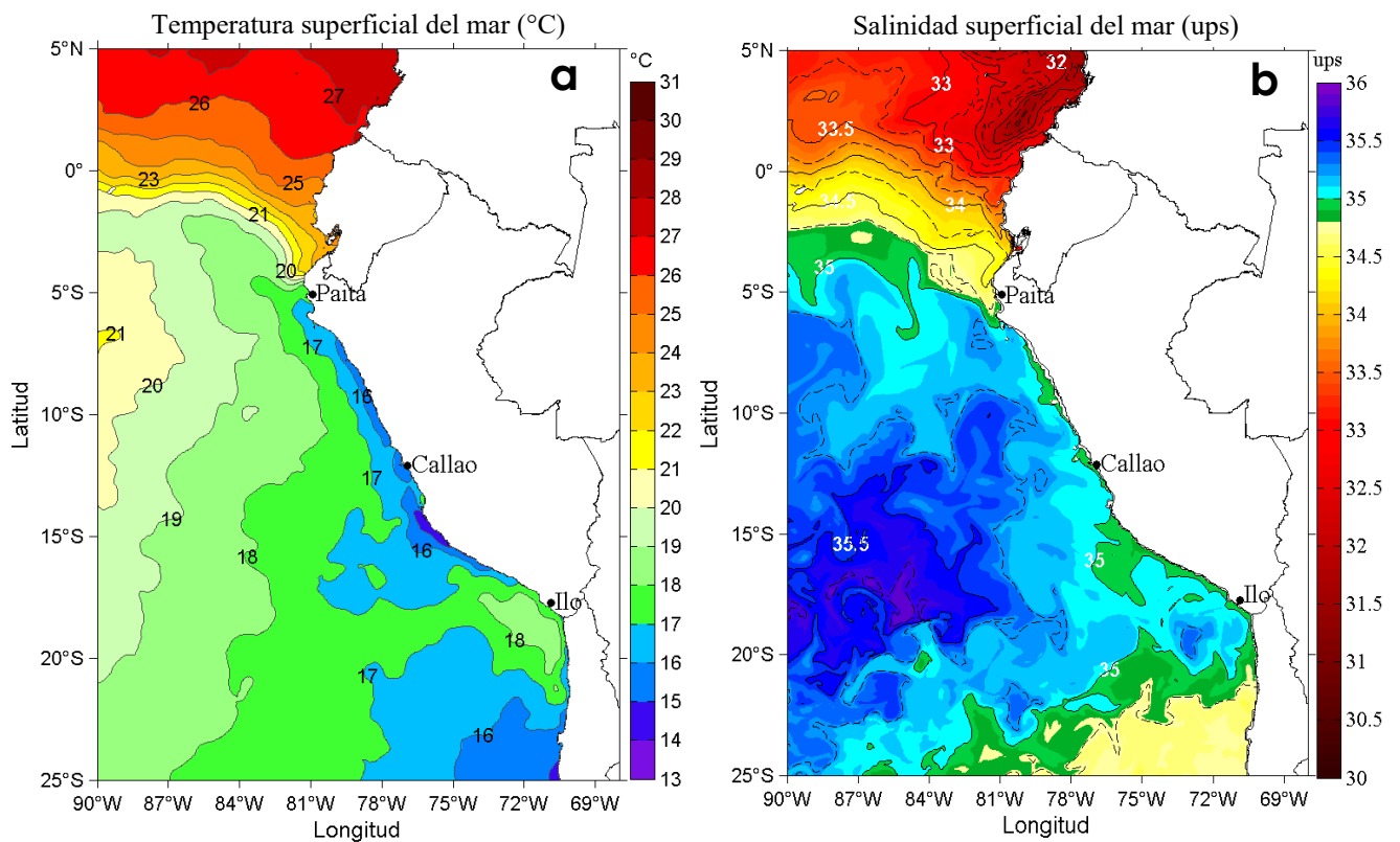
Figura 1. Distribución espacial promedio de: a) Temperatura Superficial del Mar (°C) y b) Salinidad Superficial del Mar (ups), para la semana del 22 al 28 de octubre de 2017 en el océano Pacífico tropical oriental. Datos: OSTIA-UKMO-L4-GLOB-v2.0 (UK Met Office, 2012; Donlon et al, 2012) disponible en https://podaac.jpl.nasa.gov/dataset/OSTIA-UKMO-L4-GLOB-v2.0 ) para (a) y del Hybrid Coordinate Ocean Model (HYCOM; Halliwell et al., 1998; 2000; Bleck, 2001) para (b). Las escalas de colores de la temperatura como de la salinidad superficial del mar se presentan a la derecha de cada gráfico. Procesamiento: LHFM/AFIOF/DGIOCC/IMARPE.
