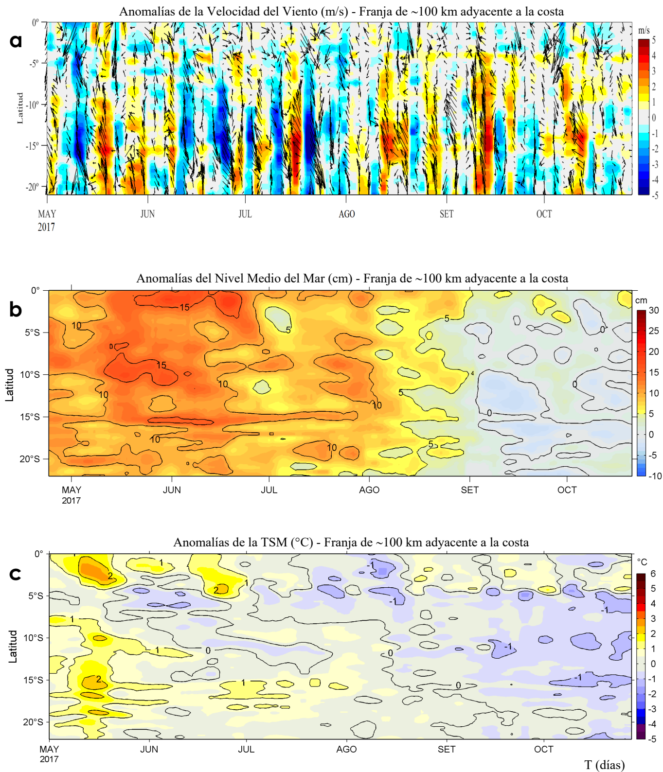
Figura 4. Evolución de las anomalías diarias de: a) velocidad del viento (m/s), b) nivel medio del mar (cm), c) temperatura superficial del mar (°C) para el último semestre actualizado al 28 de octubre de 2017. Datos: de IFREMER/CERSAT para (a), del Servicio de Monitoreo del Ambiente Marino Copernicus (CMEMS, según sus siglas en inglés) para (b), de OSTIA-UKMO-L4-GLOB-v2.0 para (c). Las anomalías fueron calculadas para una franja de 100 km adyacente a la costa entre el ecuador y 22°S según los promedios climatológicos diarios de 2000-2014 para (a), de 1993-2013 para (b) y de 2007-2016 para (c). La barra de colores a la derecha muestra la escala de las anomalías en cada caso. Procesamiento: LHF/AFIOF/DGIOCC/IMARPE.
