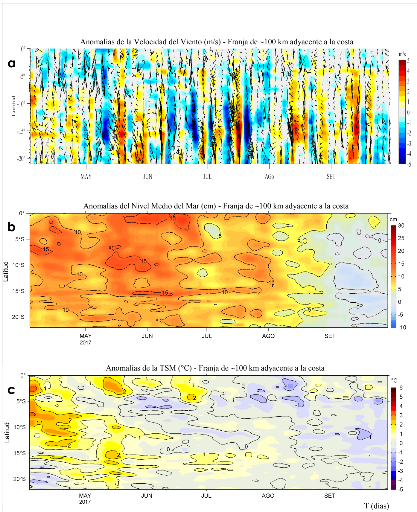
Figura 4. Evolución de las anomalías diarias de: a) velocidad del viento (m/s), b) nivel medio del mar (cm), c) temperatura superficial del mar (°C) para el último semestre actualizado al 30 de setiembre de 2017. Datos: de IFREMER/CERSAT para (a), del Servicio de Monitoreo del Ambiente Marino Copernicus (CMEMS, según sus siglas en inglés) para (b), de OSTIA-UKMO-L4-GLOB-v2.0 para (c). Las anomalías fueron calculadas para una franja de 100 km adyacente a la costa entre el ecuador y 22°S según los promedios climatológicos diarios de 2000-2014 para (a), de 1993-2013 para (b) y de 2007-2016 para (c). La barra de colores a la derecha muestra la escala de las anomalías en cada caso. Procesamiento: LHFH/AFIOF/DGIOCC/IMARPE.
