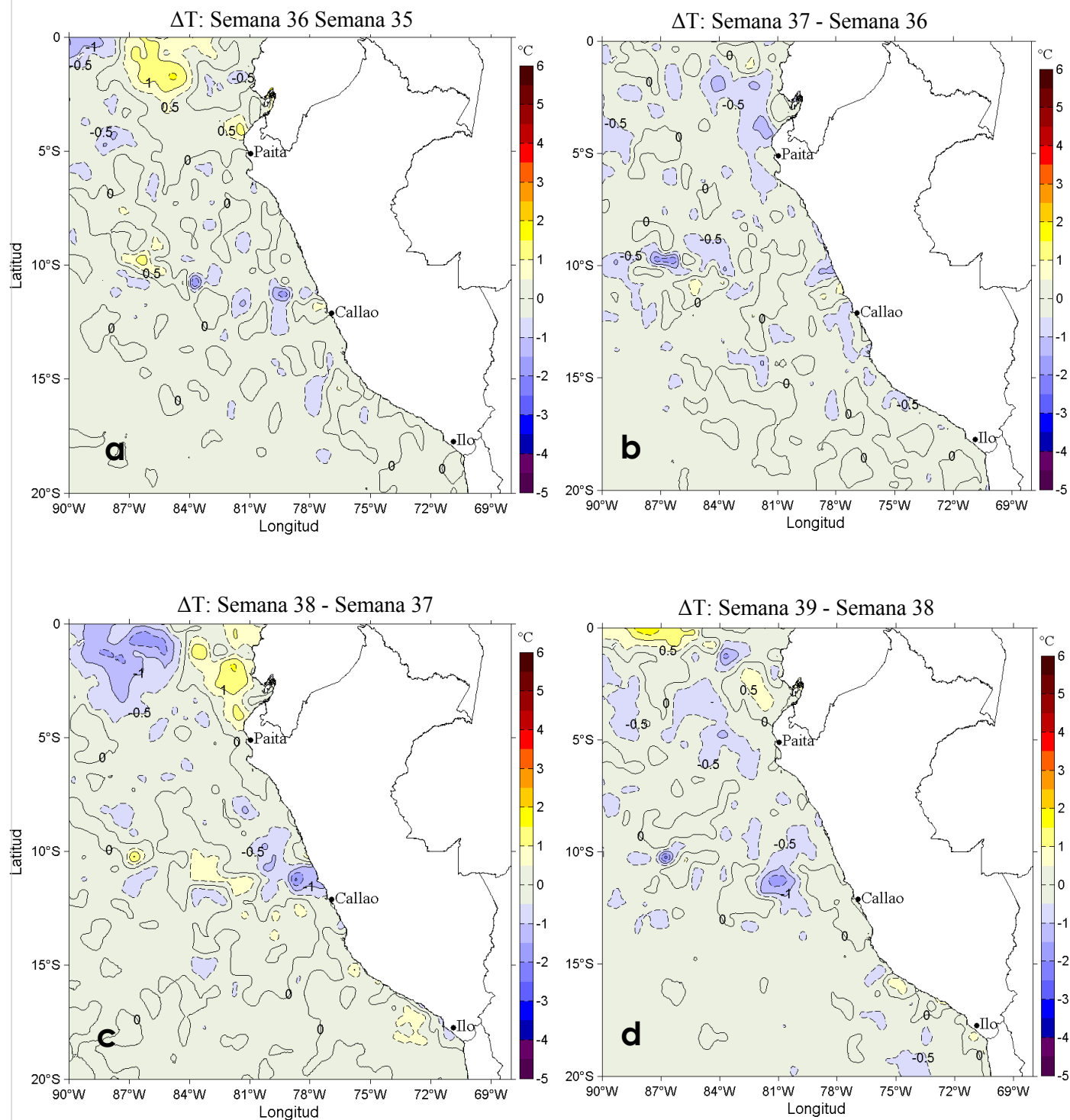
Figura 3. Variación semanal de la temperatura superficial del mar promedio ( ^{\circ}\text{C} ) en el océano Pacífico tropical oriental entre: a) trigésimo sexta (03-09 de setiembre) y trigésimo cuarta (27 de agosto-02 de setiembre) semana, b) séptima (10-16 de setiembre) y trigésimo sexta (03-09 de setiembre) semana, c) trigésimo octava (17-23 de setiembre) y trigésimo séptima (10-16 de setiembre) semana, y d) trigésimo novena (24-30 de setiembre) y trigésimo octava (17-23 de setiembre) semana del presente año.
