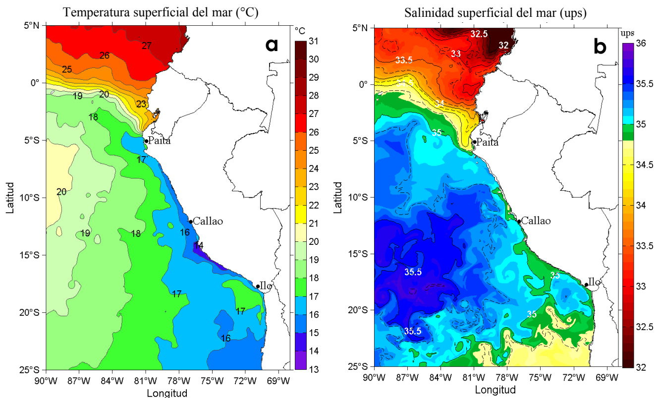
Figura 1. Distribución espacial promedio de: a) Temperatura Superficial del Mar (°C) y b) Salinidad Superficial del Mar, para la semana del 24 al 30 de setiembre de 2017 en el océano Pacífico tropical oriental. Datos: OSTIA-UKMO-L4-GLOB-v2.0 (UK Met Office, 2012; Donlon et al, 2012) disponible en https://podaac.jpl.nasa.gov/dataset/OSTIA-UKMO-L4-GLOB-v2.0 para (a) y del Hybrid Coordinate Ocean Model (HYCOM; Halliwell et al., 1998; 2000; Bleck, 2001) para (b). Las escalas de colores de la temperatura como de la salinidad superficial del mar se presentan a la derecha de cada gráfico. Procesamiento: LHF/AFIOF/DGIOCC/IMARPE.
