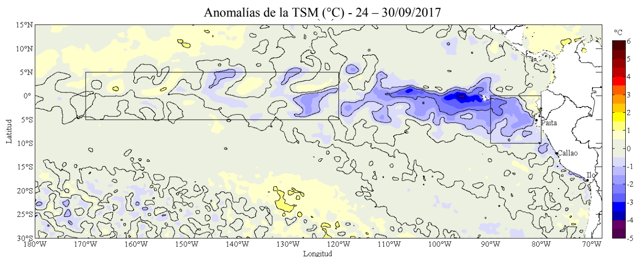
Figura 2. Anomalías promedio de la temperatura superficial del mar (°C) en el océano Pacífico tropical para la semana del 24 al 30 de setiembre de 2017. Las regiones Niño 3.4 y Niño 1+2 en los sectores central y oriental del océano, respectivamente, están delimitadas con una línea de color gris. Datos: OSTIA-UKMO-L4-GLOB-v2.0 (UK Met Office, 2012; Donlon et al, 2012) disponible en https://podaac.jpl.nasa.gov/dataset/OSTIA-UKMO-L4-GLOB-v2.0 . Las anomalías se calcularon con respecto de la climatología para el período 2007-2016. Procesamiento: IMARPE.
