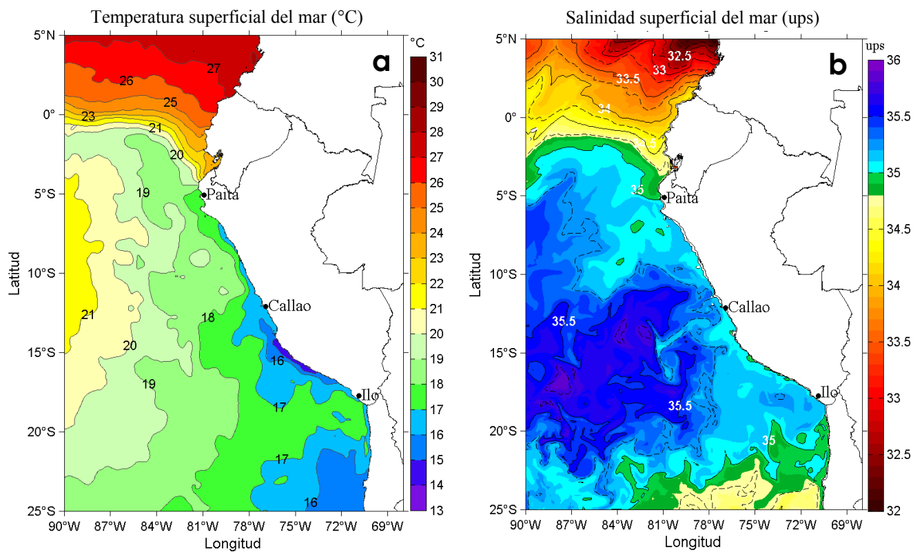
Figura 1. Distribución espacial promedio de: a) Temperatura Superficial del Mar (°C) y b) Salinidad Superficial del Mar, para la semana del 20 al 26 de agosto de 2017 en el océano Pacífico tropical oriental. Datos: OSTIA-UKMO-L4-GLOB-v2.0 (UK Met Office, 2012; Donlon et al, 2012) disponible en https://podaac.jpl.nasa.gov/dataset/OSTIA-UKMO-L4-GLOB-v2.0 para (a) y del Hybrid Coordinate Ocean Model (HYCOM; Halliwell et al., 1998; 2000; Bleck, 2001) para (b). Las escalas de colores de la temperatura como de la salinidad superficial del mar se presentan a la derecha de cada gráfico. Procesamiento: LHF/AFIOF/DGIOCC/IMARPE.
