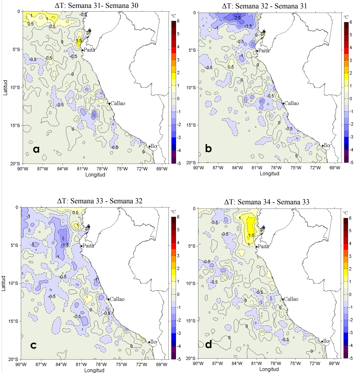
Figura 3. Variación semanal de la temperatura superficial del mar promedio ( ^{\circ}\text{C} ) en el océano Pacífico tropical oriental entre: a) trigésimo primera (30 de julio-05 de agosto) y trigésima (23-29 de julio) semana, b) trigésimo segunda (06-12 de agosto) y trigésimo primera (30 de julio-05 de agosto) semana, c) trigésimo tercera (13-19 de agosto) y trigésimo segunda (06-12 de agosto) semana, y d) trigésimo cuarta (20-26 de agosto) y trigésimo tercera (13-19 de agosto) semana del presente año. Los mapas, que indican el grado de calentamiento o enfriamiento de una semana a otra, provienen de OSTIA-UKMO-L4-GLOB-v2.0 (UK Met Office, 2012; Donlon et al, 2012). Las anomalías térmicas se calcularon de acuerdo con la climatología para el período 2007-2016. La barra de colores de las anomalías térmicas se presenta a la derecha. Procesamiento: LHF/M/AFIOF/DGIOCC/IMARPE.
