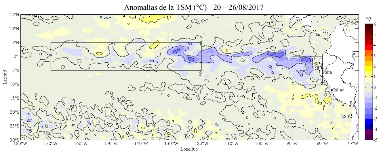
Figura 2. Anomalías promedio de la temperatura superficial del mar (°C) en el océano Pacífico tropical para la semana del 20 al 26 de agosto de 2017. Las regiones Niño 3.4 y Niño 1+2 en los sectores central y oriental del océano, respectivamente, están delimitadas con una línea de color gris. Datos: OSTIA-UKMO-L4-GLOB-v2.0 (UK Met Office, 2012; Donlon et al, 2012) disponible en https://podaac.jpl.nasa.gov/dataset/OSTIA-UKMO-L4-GLOB-v2.0 . Las anomalías se calcularon con respecto de la climatología para el período 2007-2016. Procesamiento: IMARPE.
