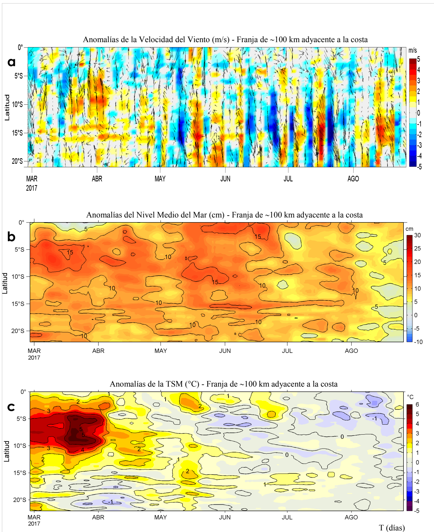
Figura 4. Evolución de las anomalías diarias de: a) velocidad del viento (m/s), b) nivel medio del mar (cm), c) temperatura superficial del mar (°C) para el último semestre actualizado al 26 de agosto de 2017. Datos: de IFREMER/CERSAT para (a), del Servicio de Monitoreo del Ambiente Marino Copernicus (CMEMS, según sus siglas en inglés) para (b), de OSTIA-UKMO-L4-GLOB-v2.0 para (c). Las anomalías fueron calculadas para una franja de 100 km adyacente a la costa entre el ecuador y 22°S según los promedios climatológicos diarios de 2000-2014 para (a), de 1993-2013 para (b) y de 2007-2016 para (c). La barra de colores a la derecha muestra la escala de las anomalías en cada caso. Procesamiento: LHF/AFIOF/DGIOCC/MARPE.
