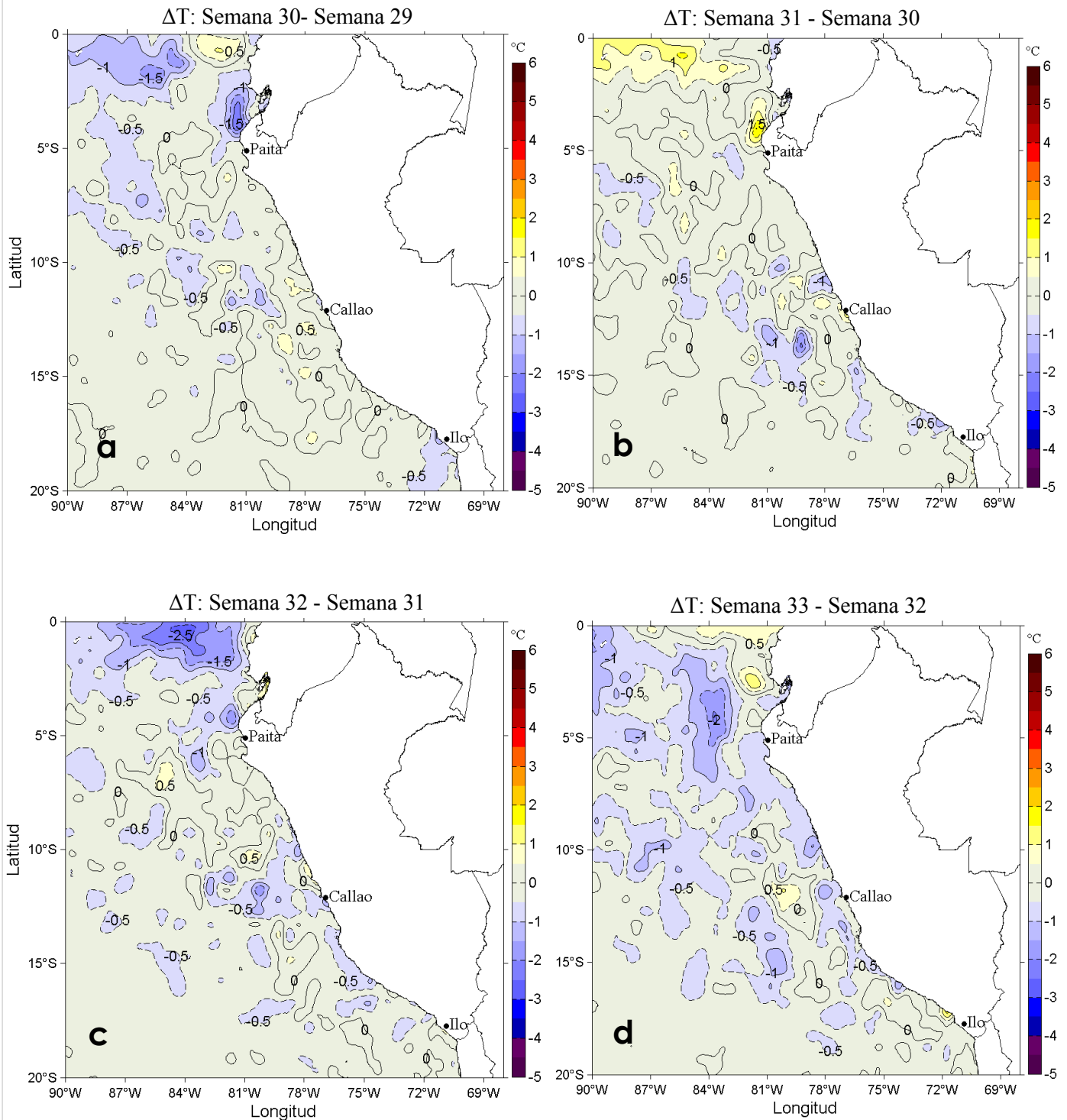
Figura 3. Variación semanal de la temperatura superficial del mar promedio ( ^{\circ}\text{C} ) en el océano Pacífico tropical oriental entre: a) trigésima (23-29 de julio) y vigésimo novena (16-22 de julio) semana, b) trigésimo primera (30 de julio-05 de agosto) y trigésima (23-29 de julio) semana, c) trigésimo segunda (06-12 de agosto) y trigésimo primera (30 de julio-05 de agosto) semana, y d) trigésimo tercera (13-19 de agosto) y trigésimo segunda (06-12 de agosto) semana del presente año. Los mapas, que indican el grado de calentamiento o enfriamiento de una semana a otra, provienen de OSTIA-UKMO-L4-GLOB-v2.0 (UK Met Office, 2012; Donlon et al, 2012). Las anomalías térmicas se calcularon de acuerdo con la climatología para el período 2007-2016. La barra de colores de las anomalías térmicas se presenta a la derecha. Procesamiento: LHF/AFIOF/DGIOCC/IMARPE.
