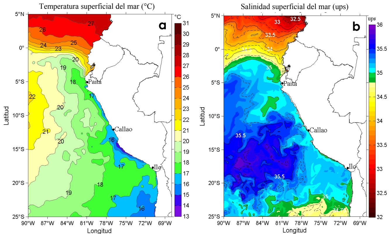
Figura 1. Distribución espacial promedio de: a) Temperatura Superficial del Mar (°C) y b) Salinidad Superficial del Mar, para la semana del 13 al 19 de agosto de 2017 en el océano Pacífico tropical oriental. Datos: OSTIA-UKMO-L4-GLOB-v2.0 (UK Met Office, 2012; Donlon et al, 2012) disponible en https://podaac.jpl.nasa.gov/dataset/OSTIA-UKMO-L4-GLOB-v2.0 para (a) y del Hybrid Coordinate Ocean Model (HYCOM; Halliwell et al., 1998; 2000; Bleck, 2001) para (b). Las escalas de colores de la temperatura como de la salinidad superficial del mar se presentan a la derecha de cada gráfico. Procesamiento: LHF/AFIOF/DGIOCC/IMARPE.
