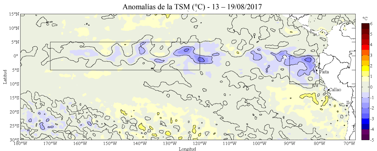
Figura 2. Anomalías promedio de la temperatura superficial del mar (°C) en el océano Pacífico tropical para la semana del 13 al 19 de agosto de 2017. Las regiones Niño 3.4 y Niño 1+2 en los sectores central y oriental del océano, respectivamente, están delimitadas con una línea de color gris. Datos: OSTIA-UKMO-L4-GLOB-v2.0 (UK Met Office, 2012; Donlon et al, 2012) disponible en https://podaac.jpl.nasa.gov/dataset/OSTIA-UKMO-L4-GLOB-v2.0 ). Las anomalías se calcularon con respecto de la climatología para el período 2007-2016. Procesamiento: IMARPE.
