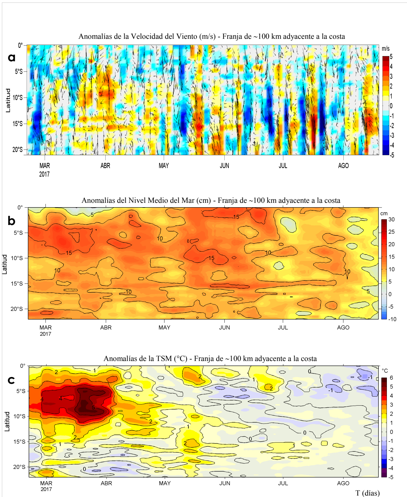
Figura 4. Evolución de las anomalías diarias de: a) velocidad del viento (m/s), b) nivel medio del mar (cm), c) temperatura superficial del mar (°C) para el último semestre actualizado al 19 de agosto de 2017. Datos: de IFREMER/CERSAT para (a), del Servicio de Monitoreo del Ambiente Marino Copernicus (CMEMS, según sus siglas en inglés) para (b), de OSTIA-UKMO-L4-GLOB-v2.0 para (c). Las anomalías fueron calculadas para una franja de 100 km adyacente a la costa entre el ecuador y 22°S según los promedios climatológicos diarios de 2000-2014 para (a), de 1993-2013 para (b) y de 2007-2016 para (c). La barra de colores a la derecha muestra la escala de las anomalías en cada caso. Procesamiento: LHF/AFIOF/DGIOCC/IMARPE.
