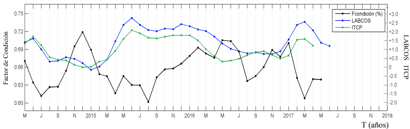
Figura 7. Series de tiempo mensual del Índice LABCOS (línea punteada de color azul), del Índice Térmico Costero Peruano (ITCP, línea de color verde) y el Factor de Condición (%) (línea de color negro) desde mayo de 2014. La metodología para estimar estos índices se encuentran en Quispe y Vásquez (2015), Quispe et al (2016), Takahashi, et al. (2014) y Perea et al (2015), respectivamente. Procesamiento: IMARPE.
