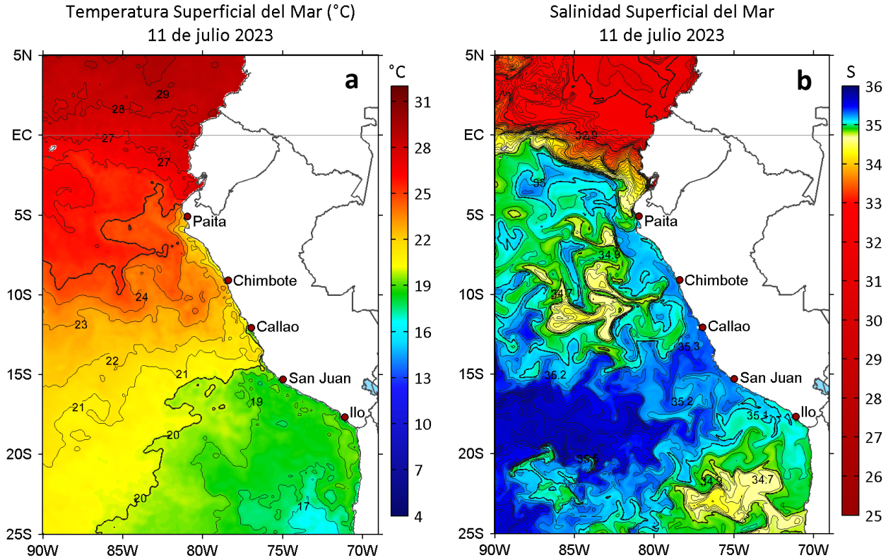
Figura 2. a) Temperatura superficial del mar (°C) y b) Salinidad superficial del mar para el 11 de julio de 2023. Datos: OSTIA-UKMO-L4-GLOB-v2.0 (UK Met Office, 2012; Donlon et al, 2012) y del GLOBAL_ANALYSISFORECAST_PHY_001_024 (Lellouche, J. M. et al, 2013), respectivamente.
