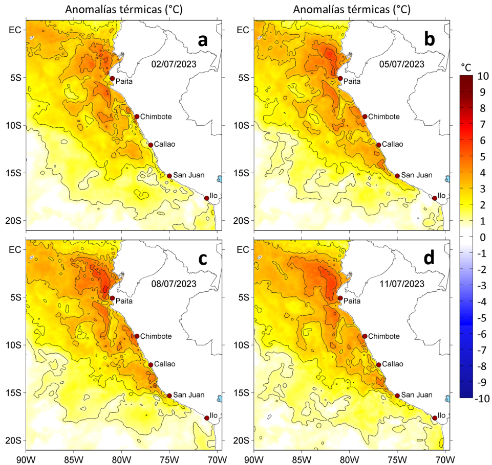
Figura 3. Anomalías de la temperatura superficial del mar (°C) para el a) 02, b) 05, c) 08 y d) 11 de julio de 2023. Las anomalías se calcularon respecto de la climatología para el periodo 2007-2016. Datos: OSTIA-UKMO-L4-GLOB-v2.0 (UK Met Office, 2012; Donlon et al, 2012).
