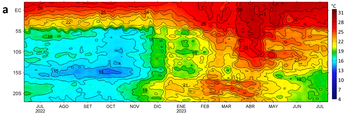
Anomalías de la Temperatura Superficial del mar (°C), franja costera de 60 m.n. 10 de junio 2022 - 11 de julio 2023
