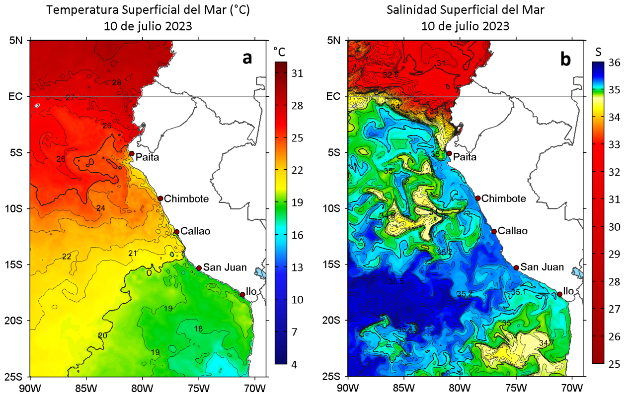
Figura 2. a) Temperatura superficial del mar ( ^{\circ}\text{C} ) y b) Salinidad superficial del mar para el 10 de julio de 2023. Datos: OSTIA-UKMO-L4-GLOB-v2.0 (UK Met Office, 2012; Donlon et al, 2012) y del GLOBAL_ANALYSISFORECAST_PHY_001_024 (Lellouche, J. M. et al, 2013), respectivamente.
