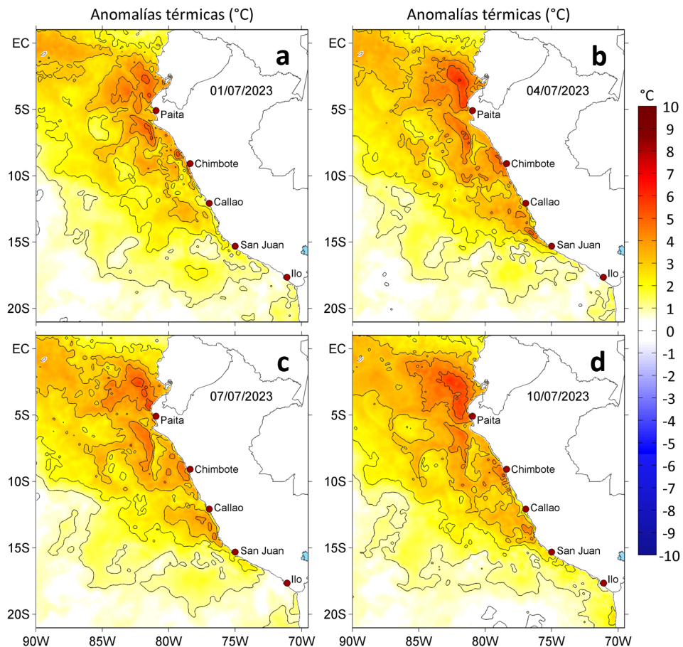
Figura 3. Anomalías de la temperatura superficial del mar ( ^{\circ}\text{C} ) para el a) 01, b) 04, c) 07 y d) 10 de julio de 2023. Las anomalías se calcularon respecto de la climatología para el periodo 2007-2016. Datos: OSTIA-UKMO-L4-GLOB-v2.0 (UK Met Office, 2012; Donlon et al, 2012).
