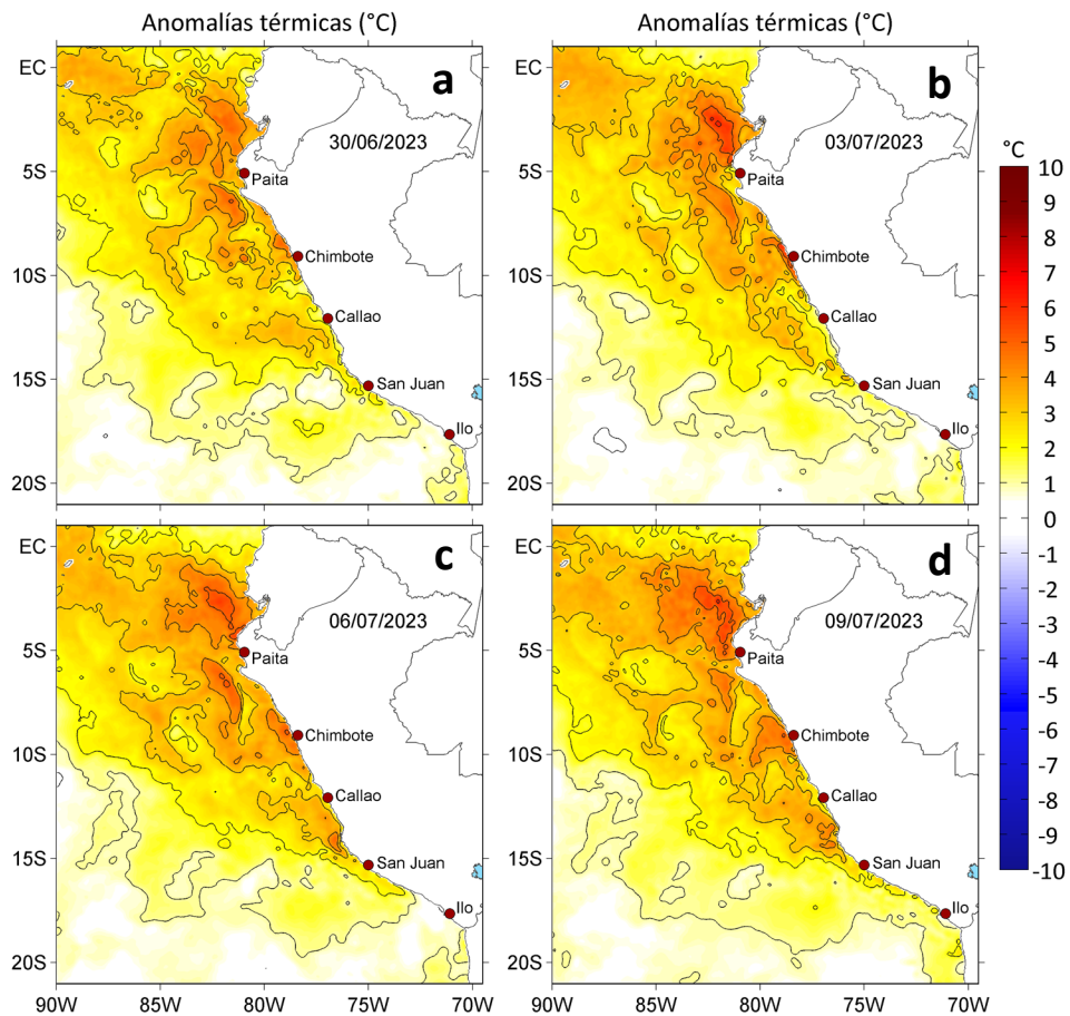
Figura 3. Anomalías de la temperatura superficial del mar ( ^{\circ}\text{C} ) para: a) 30 de junio, b) 03, c) 06 y d) 09 de julio de 2023. Las anomalías se calcularon respecto de la climatología para el periodo 2007-2016. Datos: OSTIA-UKMO-L4-GLOB-v2.0 (UK Met Office, 2012; Donlon et al, 2012).
