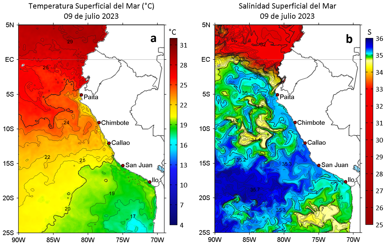
Figura 2. a) Temperatura superficial del mar ( ^{\circ}\text{C} ) y b) Salinidad superficial del mar para el 09 de julio de 2023. Datos: OSTIA-UKMO-L4-GLOB-v2.0 (UK Met Office, 2012; Donlon et al, 2012) y del GLOBAL_ANALYSISFORECAST_PHY_001_024 (Lellouche, J. M. et al, 2013), respectivamente.
