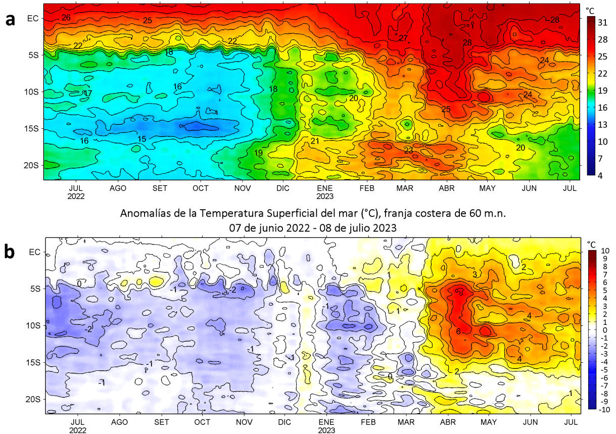
Figura 4. Variación promedio diaria de a) temperatura superficial del mar (°C) y b) anomalías térmicas (°C) para una franja de 60 m.n. adyacente al litoral peruano para los últimos trece meses. Datos: OSTIA-UKMO-L4-GLOB-v2.0 (UK Met. Office, 2012; Donlon et al, 2012) disponible en https://podaac.jpl.nasa.gov/dataset/OSTIA-UKMO-L4-GLOB-v2.0 . Las anomalías se calcularon con respecto al periodo 2007-2016.
