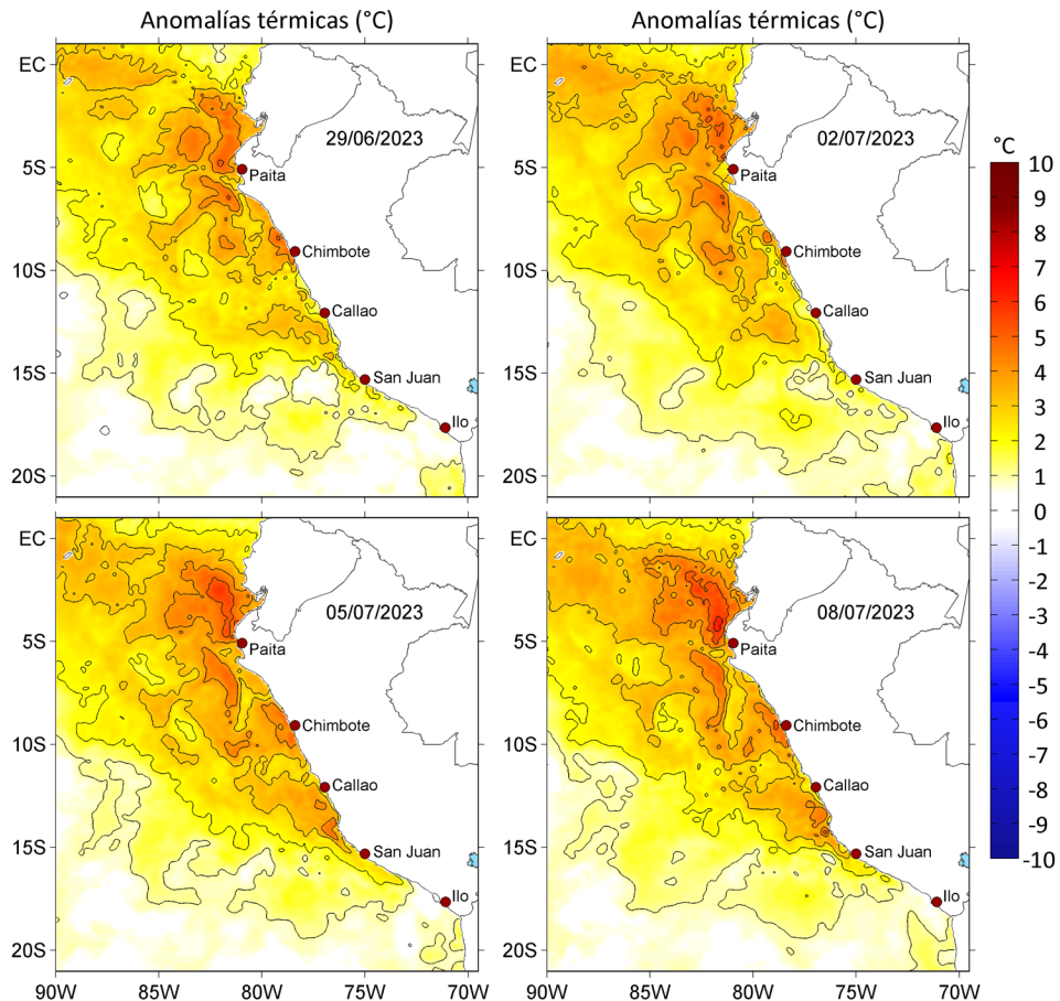
Figura 3. Anomalías de la temperatura superficial del mar ( ^{\circ}\text{C} ) para el a) 29 de junio, b) 02, c) 05 y d) 08 de julio de 2023. Las anomalías se calcularon respecto de la climatología para el periodo 2007-2016. Datos: OSTIA-UKMO-L4-GLOB-v2.0 (UK Met Office, 2012; Donlon et al, 2012).
