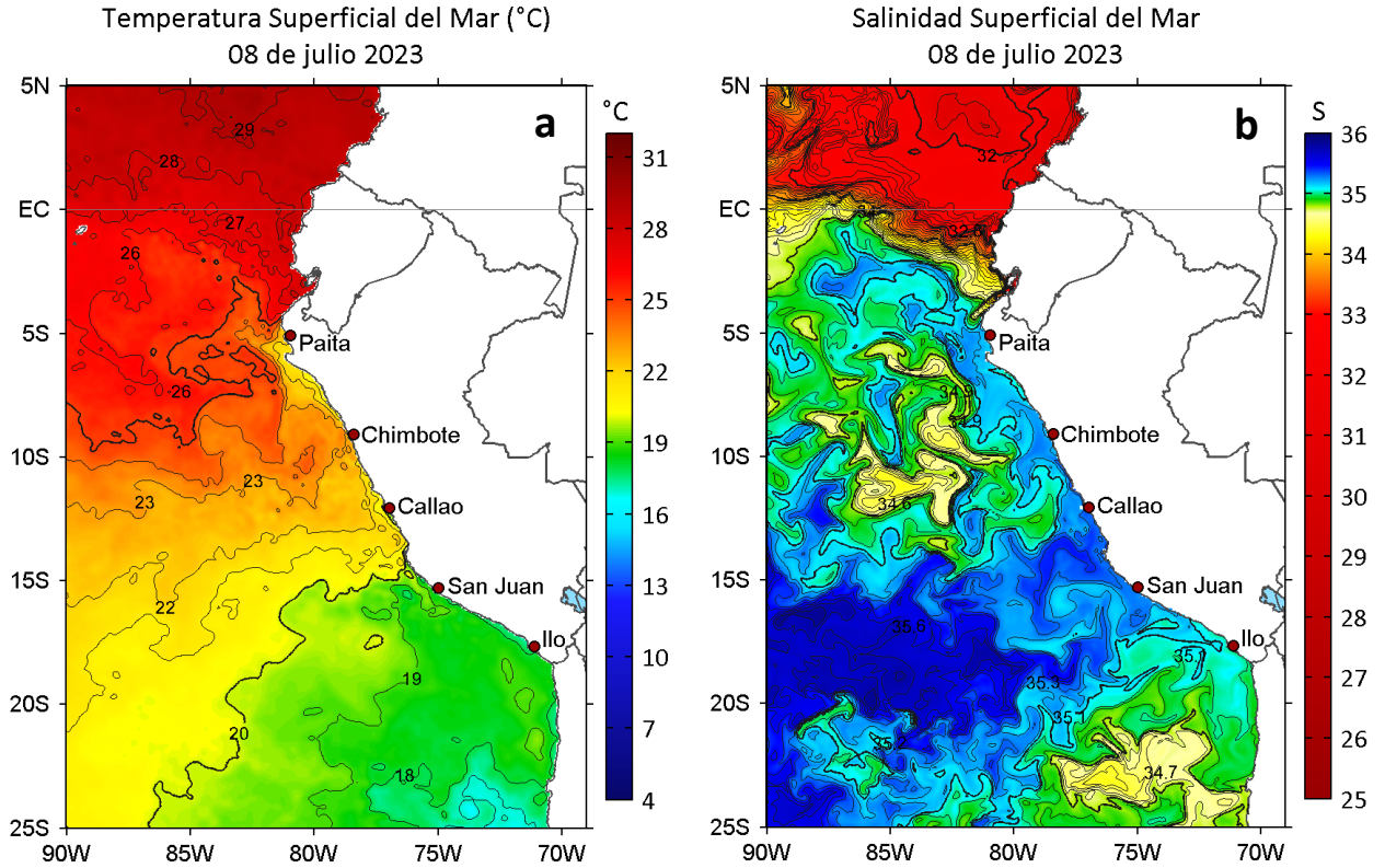
Figura 2. a) Temperatura superficial del mar ( ^{\circ}\text{C} ) y b) Salinidad superficial del mar para el 08 de julio de 2023. Datos: OSTIA-UKMO-L4-GLOB-v2.0 (UK Met Office, 2012; Donlon et al, 2012) y del GLOBAL_ANALYSISFORECAST_PHY_001_024 (Lellouche, J. M. et al, 2013), respectivamente.
