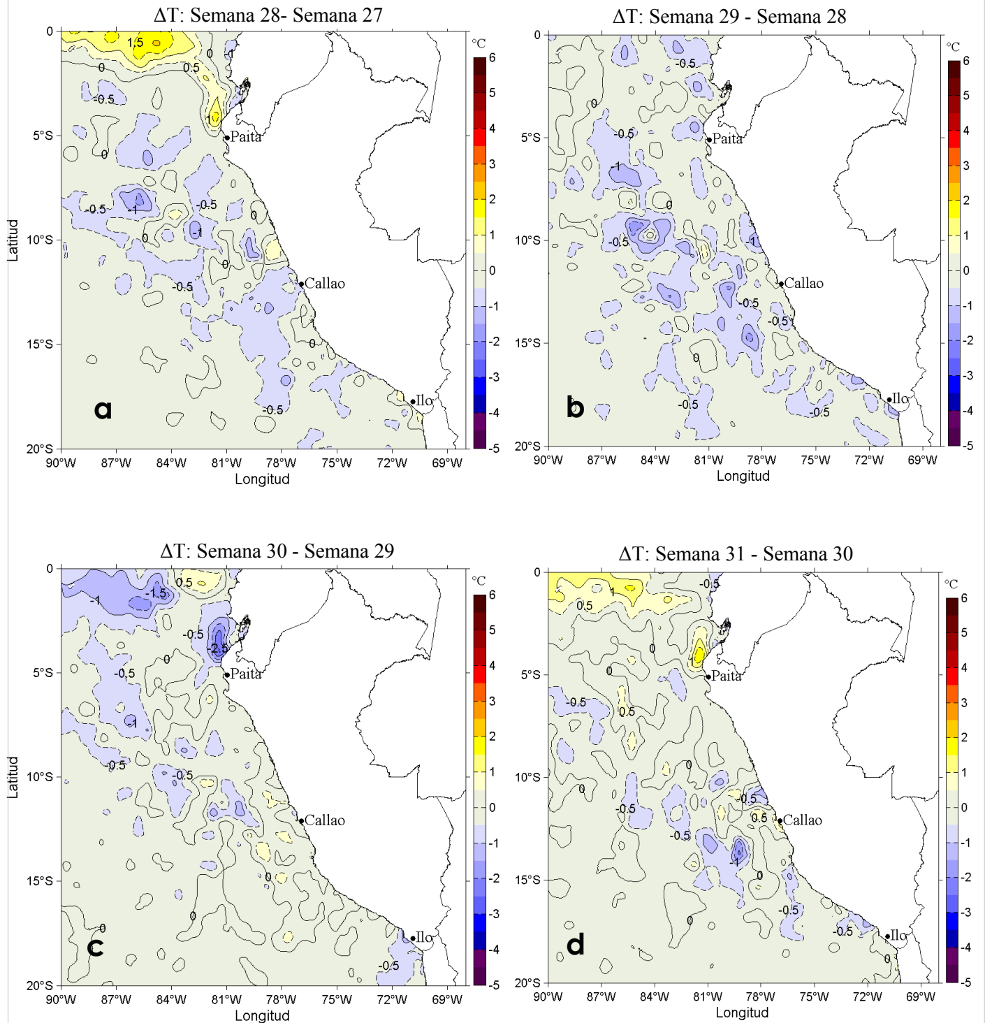
Figura 3. Variación semanal de la temperatura superficial del mar promedio ( ^{\circ}\text{C} ) en el océano Pacífico tropical oriental entre la: a) vigésimo octava (09-15 de julio) y vigésimo séptima (02-08 de julio) semana, b) vigésimo novena (16-22 de julio) y vigésimo octava (09-15 de julio) semana, c) trigésima (23-29 de julio) y vigésimo novena (16-22 de julio) semanas, y d) trigésimo primera (30 de julio-05 de agosto) y trigésima (23-29 de julio) semana del presente año.
