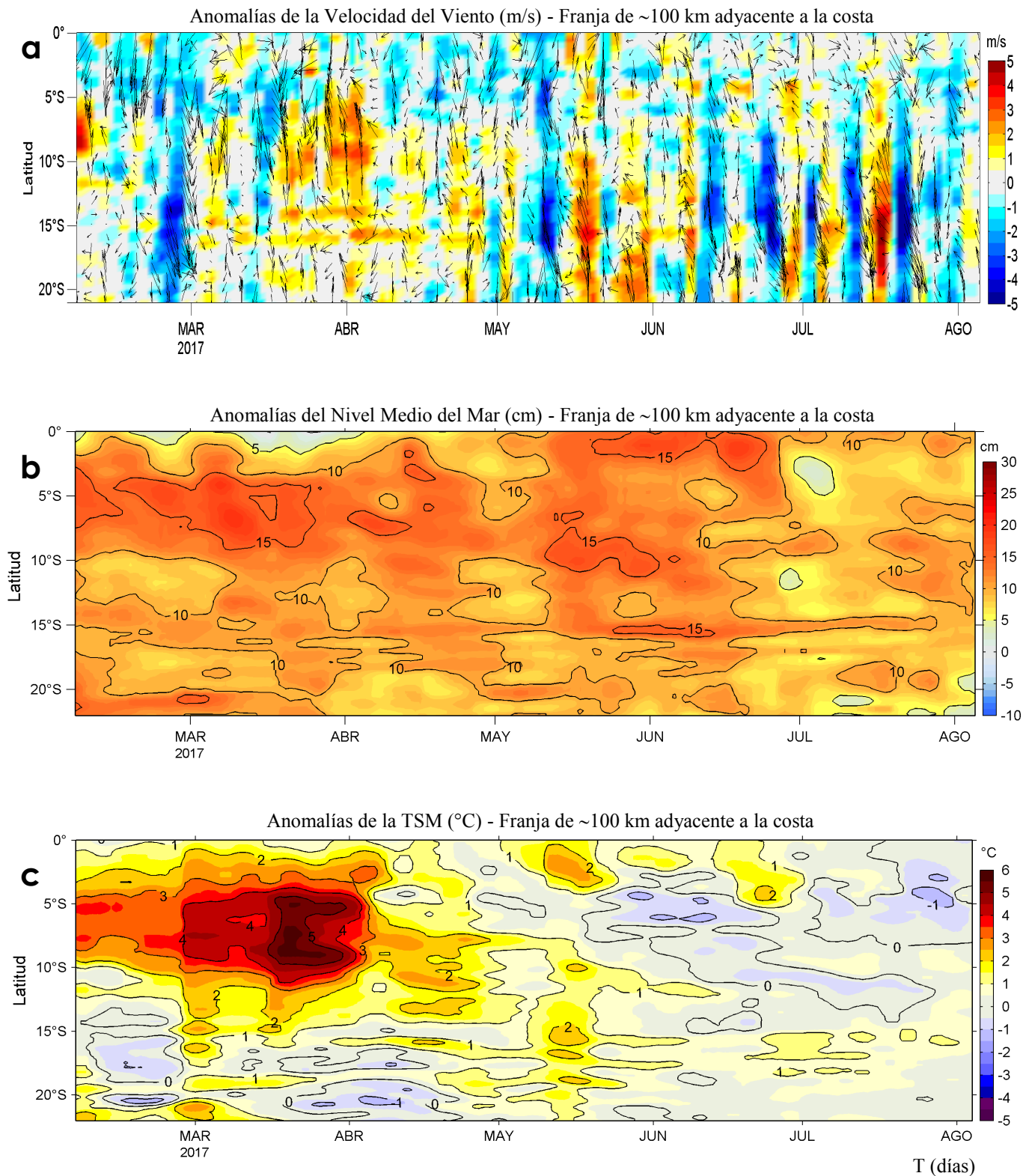
Figura 4. Evolución de las anomalías diarias de: a) velocidad del viento (m/s), b) nivel medio del mar (cm), c) temperatura superficial del mar (°C) para el último semestre actualizado al 05 de agosto de 2017. Datos: de IFREMER/CERSAT para (a), del Servicio de Monitoreo del Ambiente Marino Copernicus (CMEMS, según sus siglas en inglés) para (b), de OSTIA-UKMO-L4-GLOB-v2.0 para (c). Las anomalías fueron calculadas para una franja de 100 km adyacente a la costa entre el ecuador y 22°S según los promedios climatológicos diarios de 2000-2014 para (a), de 1993-2013 para (b) y de 2007-2016 para (c). La barra de colores a la derecha muestra la escala de las anomalías en cada caso. Procesamiento: LHF/AFIOF/DGIOCC/MARPE.
