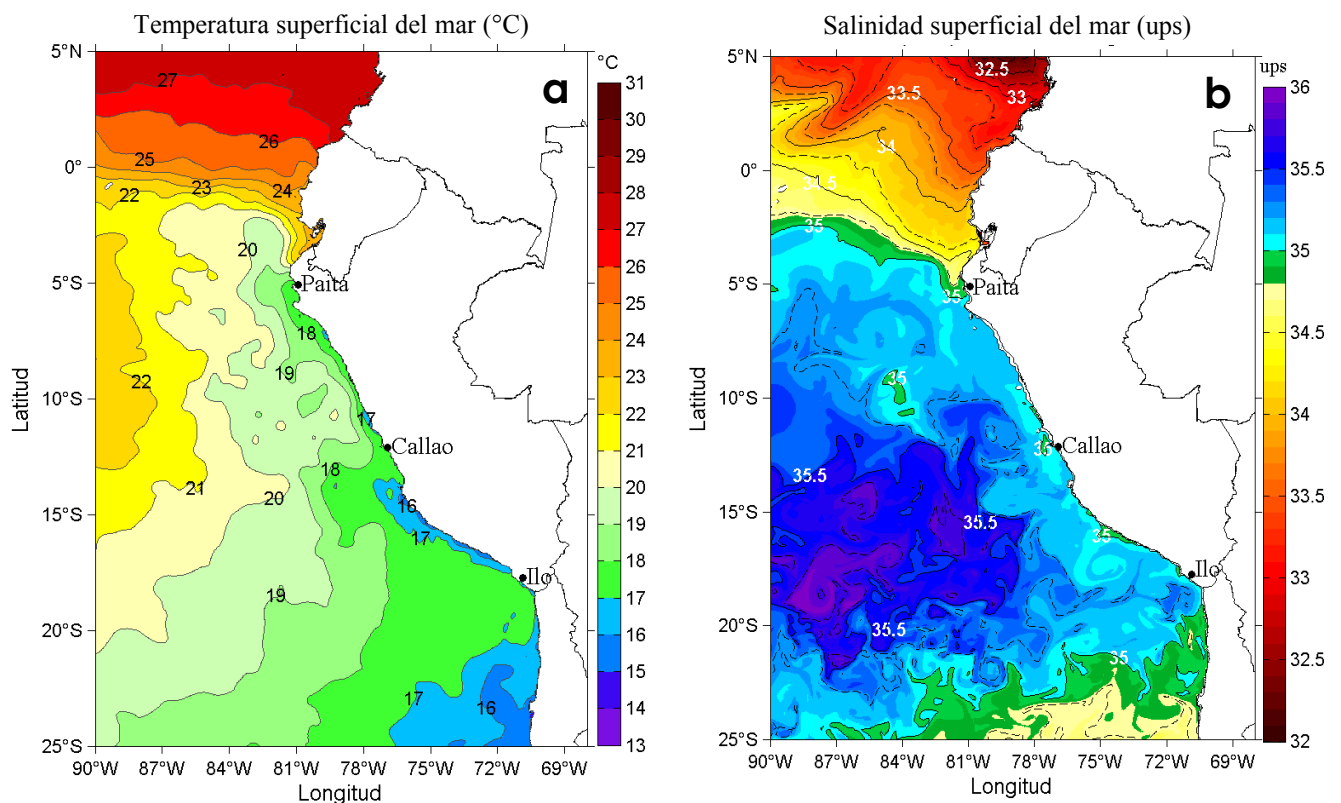
Figura 1. Distribución espacial promedio de: a) Temperatura Superficial del Mar (°C) y b) Salinidad Superficial del Mar, para la semana del 30 de julio al 05 de agosto de 2017 en el océano Pacífico tropical oriental. Datos: OSTIA-UKMO-L4-GLOB-v2.0 (UK Met Office, 2012; Donlon et al, 2012) disponible en https://podaac.jpl.nasa.gov/dataset/OSTIA-UKMO-L4-GLOB-v2.0 ) para (a) y del Hybrid Coordinate Ocean Model (HYCOM; Halliwell et al., 1998; 2000; Bleck, 2001) para (b). Las escalas de colores de la temperatura como de la salinidad superficial del mar se presentan a la derecha de cada gráfico. Procesamiento: LHF/AFIOF/DGIOCC/IMARPE.
