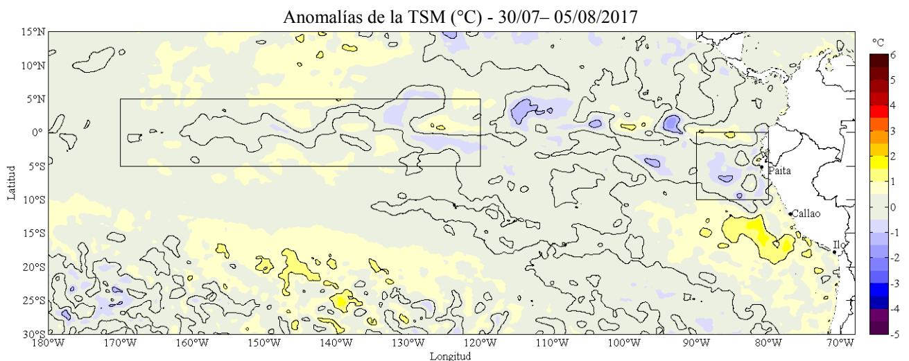
Figura 2. Anomalías promedio de la temperatura superficial del mar (°C) en el océano Pacífico tropical para la semana del 30 de julio al 05 de agosto de 2017. Las regiones Niño 3.4 y Niño 1+2 en los sectores central y oriental del océano, respectivamente, están delimitadas con una línea de color gris. Datos: OSTIA-UKMO-L4-GLOB-v2.0 (UK Met Office, 2012; Donlon et al, 2012) disponible en https://podaac.jpl.nasa.gov/dataset/OSTIA-UKMO-L4-GLOB-v2.0 ). Las anomalías se calcularon con respecto de la climatología para el período 2007-2016. Procesamiento: IMARPE.
