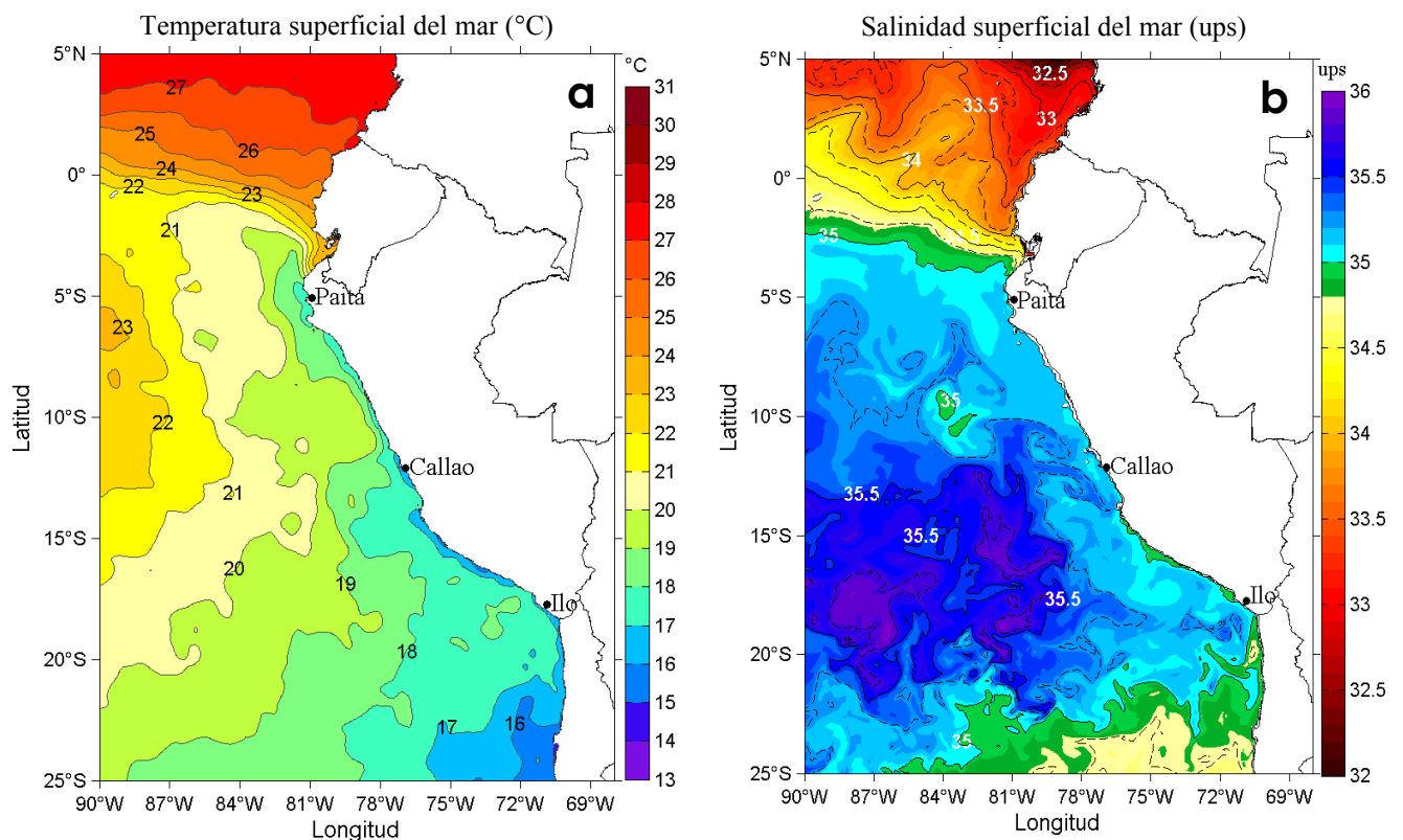
Figura 1. Distribución espacial promedio de: a) Temperatura Superficial del Mar (°C) y b) Salinidad Superficial del Mar, para la semana del 23 al 29 de julio de en el océano Pacífico tropical oriental. Datos: OSTIA-UKMO-L4-GLOB-v2.0 (UK Met Office, 2012; Donlon et al, 2012) disponible en https://podaac.jpl.nasa.gov/dataset/OSTIA-UKMO-L4-GLOB-v2.0 para (a) y del Hybrid Coordinate Ocean Model (HYCOM; Halliwell et al., 1998; 2000; Bleck, 2001) para (b). Las escalas de colores de la temperatura como de la salinidad superficial del mar se presentan a la derecha de cada gráfico. Procesamiento: LHFM/AFIOF/DGIOCC/IMARPE.
