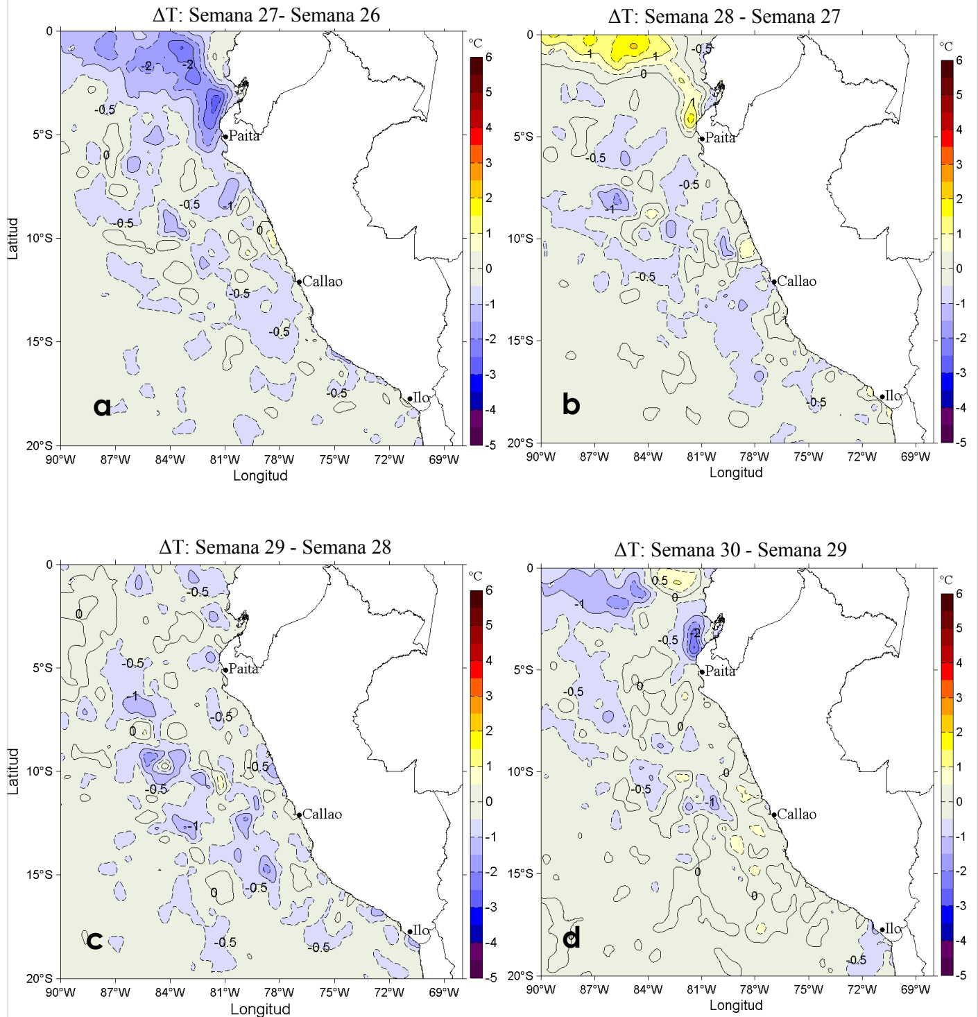
Figura 3. Variación semanal de la temperatura superficial del mar promedio ( ^{\circ}\text{C} ) en el océano Pacífico tropical oriental entre: a) vigésimo séptima (02-08 de julio) y vigésima sexta (25 de junio-01 de julio) semana, b) vigésimo octava (09-15 de julio) y vigésima séptima (02-08 de julio) semana, c) vigésimo novena (16-22 de julio) y vigésimo octava (09-15 de julio) semana, y d) trigésima (23-29 de julio) y vigésimo novena (16-22 de julio) semana del presente año.
