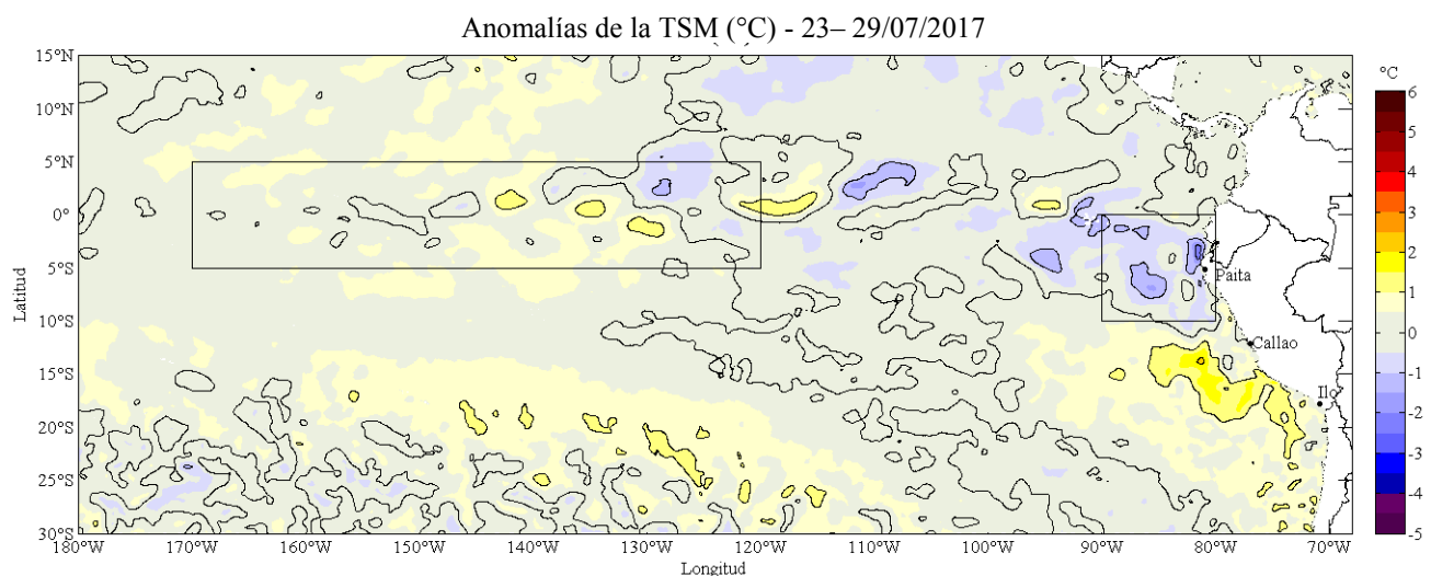
Figura 2. Anomalías promedio de la temperatura superficial del mar (°C) en el océano Pacífico tropical para la semana del 23 al 29 de julio de 2017. Las regiones Niño 3.4 y Niño 1+2 en los sectores central y oriental del océano, respectivamente, están delimitadas con una línea de color gris. Datos: OSTIA-UKMO-L4-GLOB-v2.0 (UK Met Office, 2012; Donlon et al, 2012) disponible en https://podaac.jpl.nasa.gov/dataset/OSTIA-UKMO-L4-GLOB-v2.0 . Las anomalías se calcularon con respecto de la climatología para el período 2007-2016. Procesamiento: IMARPE.
