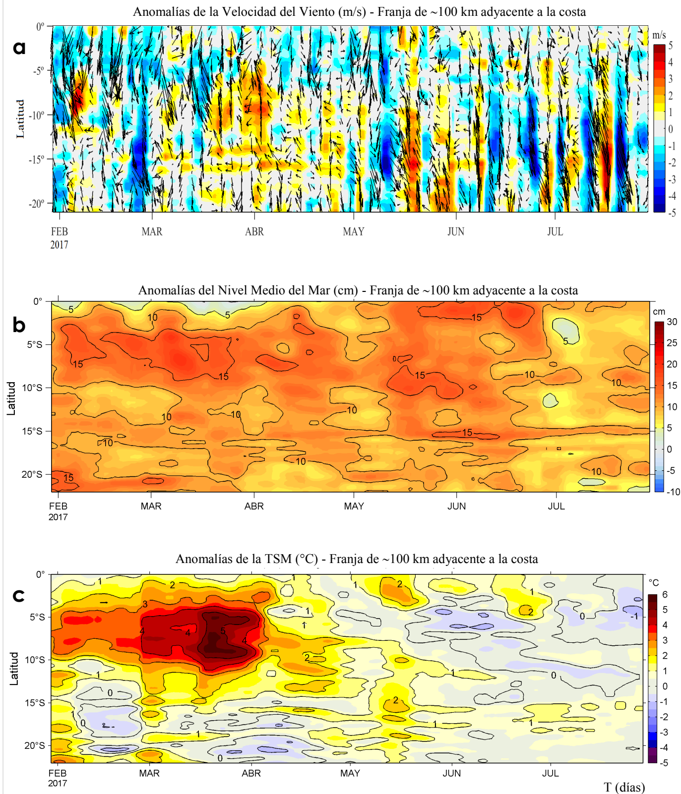
Figura 4. Evolución de las anomalías diarias de: a) velocidad del viento (m/s), b) nivel medio del mar (cm), c) temperatura superficial del mar (°C) para el último semestre actualizado al 29 de julio de 2017. Datos: de IFREMER/CERSAT para (a), del Servicio de Monitoreo del Ambiente Marino Copernicus (CMEMS, según sus siglas en inglés) para (b), de OSTIA-UKMO-L4-GLOB-v2.0 para (c). Las anomalías fueron calculadas para una franja de 100 km adyacente a la costa entre el ecuador y 22°S según los promedios climatológicos diarios de 2000-2014 para (a), de 1993-2013 para (b) y de 2007-2016 para (c). La barra de colores a la derecha muestra la escala de las anomalías en cada caso. Procesamiento: LHF/AFIOF/DGIOCC/MARPE.
