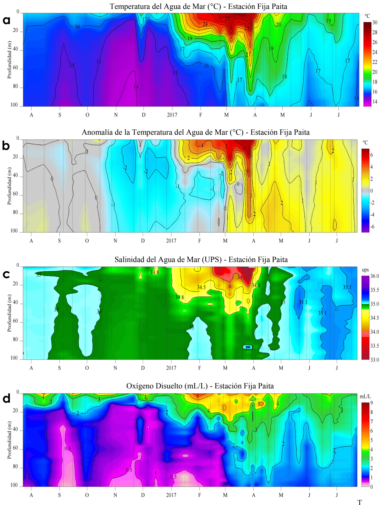
Figura 5. Evolución de: a) Temperatura del agua de mar (°C), b) Anomalías térmicas (°C), c) Salinidad del agua de mar, d) Contenido de Oxígeno disuelto (mL/L) para la estación fija Paita, localizada a 7 mn de esta localidad, de abril de 2016 al 23 de julio de 2017. Las anomalías de la temperatura del agua (°C), salinidad y de oxígeno disuelto (mL/L) se calcularon en base al promedio climatológico de 1981-2010 de acuerdo a Anculle, et al (2015). Los puntos en la columna de agua indican los días en que se realizó la estación fija Paita. Datos: Monterrey Bay Aquarium Research Institute (MBARI) para el periodo de 1982 a mayo de 2013, así como de IMARPE para el periodo de 2013 al 15 de junio de 2016. Procesamiento: LHF/M/ AFIOF/DGIOCC/IMARPE.
