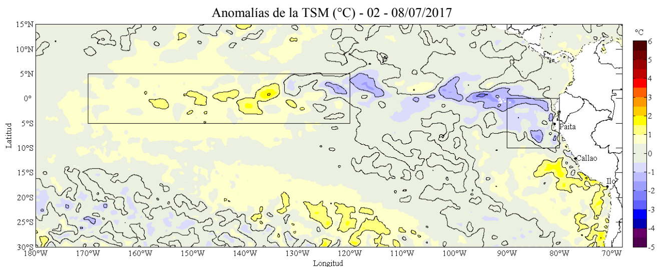
Figura 2. Anomalías promedio de la temperatura superficial del mar (°C) en el océano Pacífico tropical para la semana del 02 al 08 de julio de 2017. Las regiones Niño 3.4 y Niño 1+2 en los sectores central y oriental del océano, respectivamente, están delimitadas con una línea de color gris. Datos: OSTIA-UKMO-L4-GLOB-v2.0 (UK Met Office, 2012; Donlon et al, 2012) disponible en https://podaac.jpl.nasa.gov/dataset/OSTIA-UKMO-L4-GLOB-v2.0 . Las anomalías se calcularon con respecto de la climatología para el período 2007-2016. Procesamiento: IMARPE.
