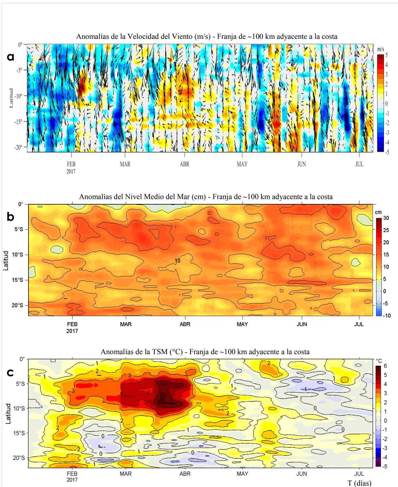
Figura 4. Evolución de las anomalías diarias de: a) velocidad del viento (m/s), b) nivel medio del mar (cm), c) temperatura superficial del mar (°C) para el último semestre actualizado al 08 de julio de 2017. Datos: de IFREMER/CERSAT para (a), del Servicio de Monitoreo del Ambiente Marino Copernicus (CMEMS, según sus siglas en inglés) para (b), de OSTIA-UKMO-L4-GLOB-v2.0 para (c). Las anomalías fueron calculadas para una franja de 100 km adyacente a la costa entre el ecuador y 22°S según los promedios climatológicos diarios de 2000-2014 para (a), de 1993-2013 para (b) y de 2007-2016 para (c). La barra de colores a la derecha muestra la escala de las anomalías en cada caso. Procesamiento: LHF/AFIOF/DGIOCC/IMARPE.
