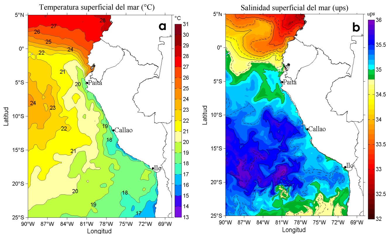
Figura 1. Distribución espacial promedio de: a) Temperatura Superficial del Mar (°C) y b) Salinidad Superficial del Mar, para la semana del 02 al 08 de julio de en el océano Pacífico tropical oriental. Datos: OSTIA-UKMO-L4-GLOB-v2.0 (UK Met Office, 2012; Donlon et al, 2012) disponible en https://podaac.jpl.nasa.gov/dataset/OSTIA-UKMO-L4-GLOB-v2.0 para (a) y del Hybrid Coordinate Ocean Model (HYCOM; Halliwell et al., 1998; 2000; Bleck, 2001) para (b). Las escalas de colores de la temperatura como de la salinidad superficial del mar se presentan a la derecha de cada gráfico. Procesamiento: LHFM/AFIOF/DGIOCC/IMARPE.
