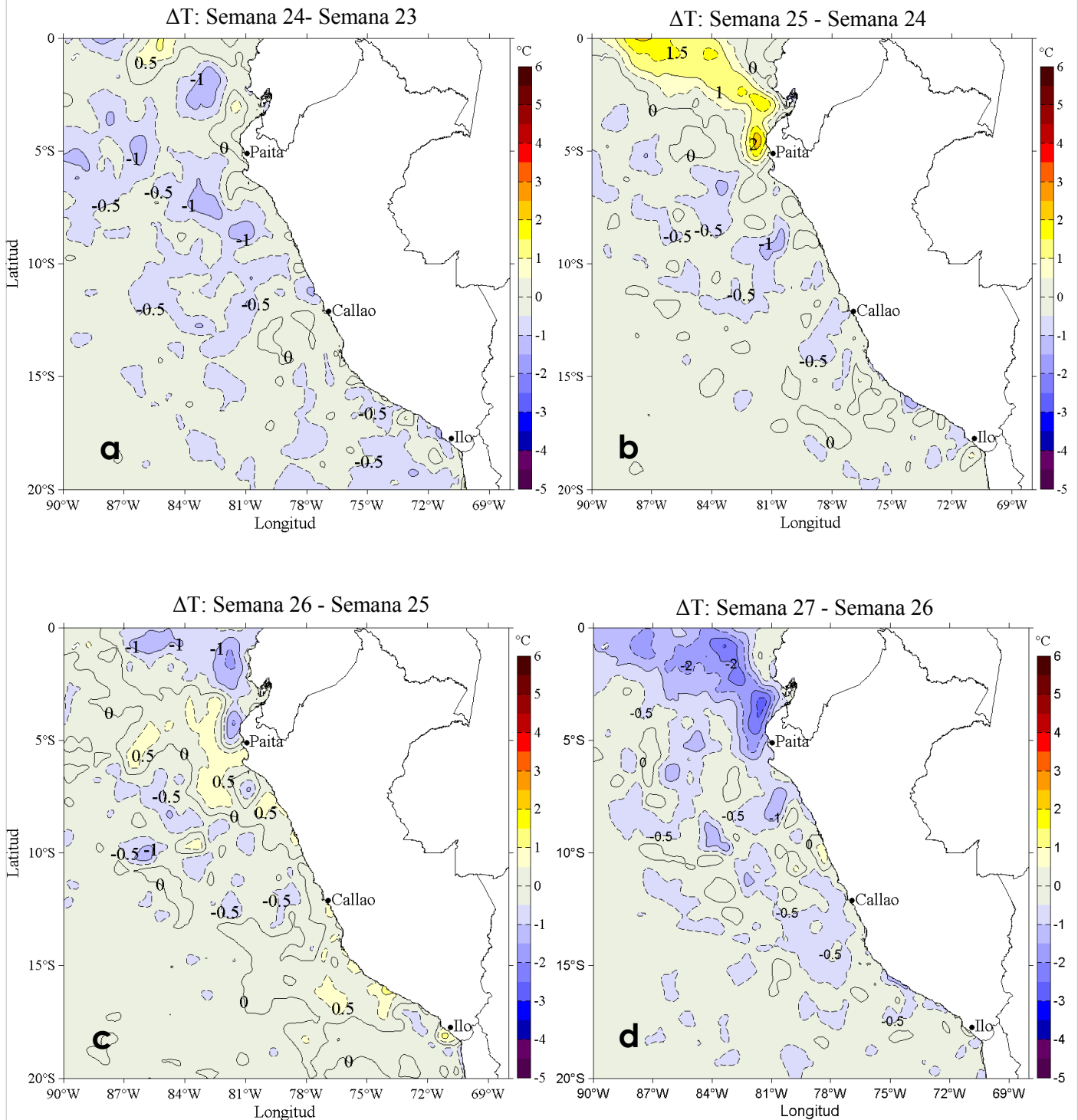
Figura 3. Variación semanal de la temperatura superficial del mar promedio ( ^{\circ}\text{C} ) en el océano Pacífico tropical oriental entre: a) vigésima cuarta (11-17 de junio) y vigésima tercera (04-10 de junio) semana, b) vigésima quinta (18-24 de junio) y vigésima cuarta (11-17 de junio) semana, c) vigésima sexta (25 de junio-01 de julio) y vigésima quinta (18-24 de junio) semana, y d) vigésimo séptima (02-08 de julio) y vigésima sexta (25 de junio-01 de julio) semana del presente año.
