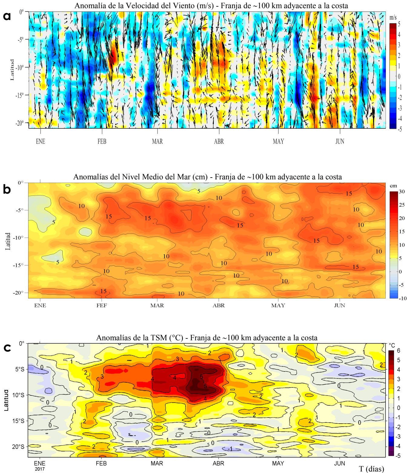
Figura 4. Evolución de las anomalías diarias de: a) velocidad del viento (m/s), b) nivel medio del mar (cm), c) temperatura superficial del mar (°C) para el último semestre actualizado al 24 de junio de 2017. Datos: de IFREMER/CERSAT para (a), del Servicio de Monitoreo del Ambiente Marino Copernicus (CMEMS, según sus siglas en inglés) para (b), de OSTIA-UKMO-L4-GLOB-v2.0 para (c). Las anomalías fueron calculadas para una franja de 100 km adyacente a la costa entre el ecuador y 22°S según los promedios climatológicos diarios de 2000-2014 para (a), de 1993-2013 para (b) y de 2007-2016 para (c). La barra de colores a la derecha muestra la escala de las anomalías en cada caso. Procesamiento: LHF/AFIOF/DGIOCC/IMARPE.
