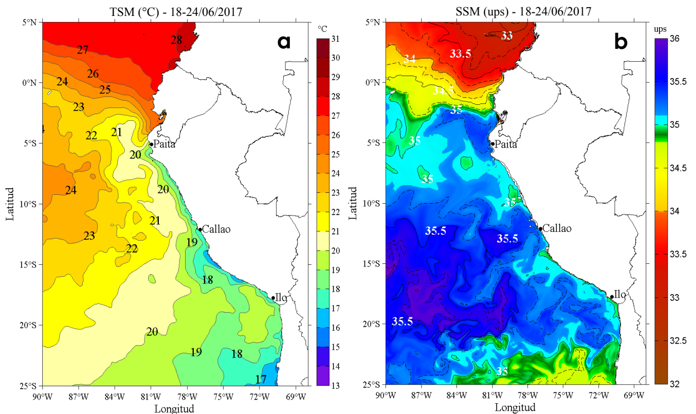
Figura 1. Distribución espacial promedio de: a) Temperatura Superficial del Mar (°C) y b) Salinidad Superficial del Mar (ups) para la semana del 18 al 24 de junio de 2017 en el océano Pacífico tropical oriental. Datos: OSTIA-UKMO-L4-GLOB-v2.0 (UK Met Office, 2012; Donlon et al, 2012) disponible en https://podaac.jpl.nasa.gov/dataset/OSTIA-UKMO-L4-GLOB-v2.0 para (a) y del Hybrid Coordinate Ocean Model (HYCOM; Halliwell et al., 1998; 2000; Bleck, 2001) para (b). Las escalas de colores de la temperatura como de la salinidad superficial del mar se presentan a la derecha de cada gráfico. Procesamiento: LHFM/AFIOF/DGIOCC/IMARPE.
