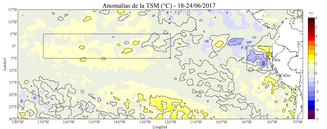
Figura 2. Anomalías promedio de la temperatura superficial del mar (°C) en el océano Pacífico tropical para la semana del 18 al 24 de junio de 2017. Las regiones Niño 3.4 y Niño 1+2 en los sectores central y oriental del océano, respectivamente, están delimitadas con una línea de color gris. Datos: OSTIA-UKMO-L4-GLOB-v2.0 (UK Met Office, 2012; Donlon et al, 2012) disponible en https://podaac.jpl.nasa.gov/dataset/OSTIA-UKMO-L4-GLOB-v2.0 . Las anomalías se calcularon con respecto de la climatología para el período 2007-2016. Procesamiento: IMARPE.
