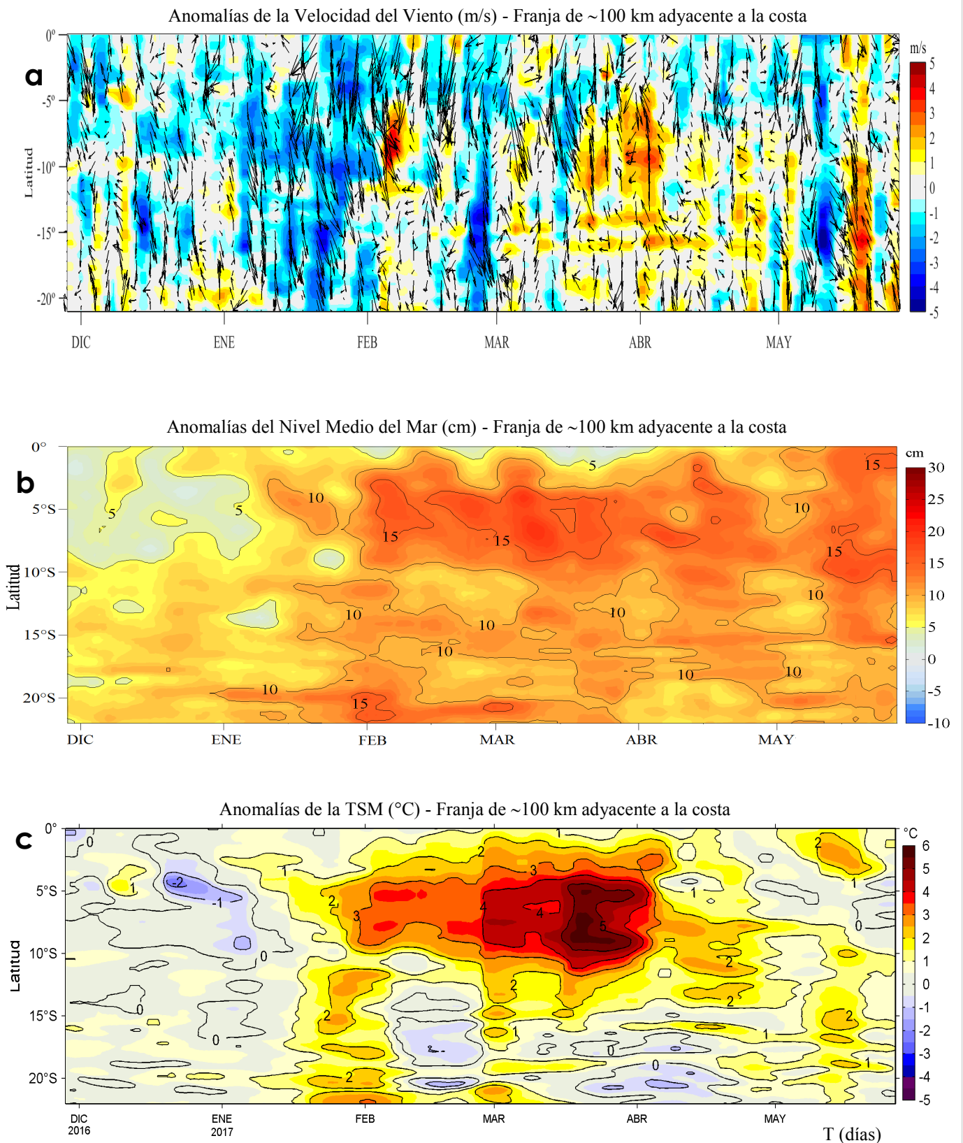
Figura 4. Evolución de las anomalías diarias de: a) velocidad del viento (m/s), b) nivel medio del mar (cm), c) temperatura superficial del mar (°C) para el último semestre actualizado al 27 de mayo de 2017. Datos: de IFREMER/CERSAT para (a), del Servicio de Monitoreo del Ambiente Marino Copernicus (CMEMS, según sus siglas en inglés) para (b), de OSTIA-UKMO-L4-GLOB-v2.0 para (c). Las anomalías fueron calculadas para una franja de 100 km adyacente a la costa entre el ecuador y 22°S según los promedios climatológicos diarios de 2000-2014 para (a), de 1993-2013 para (b) y de 2007-2016 para (c). La barra de colores a la derecha muestra la escala de las anomalías en cada caso. Procesamiento: LHF/AFIOF/DGIOCC/IMARPE.
