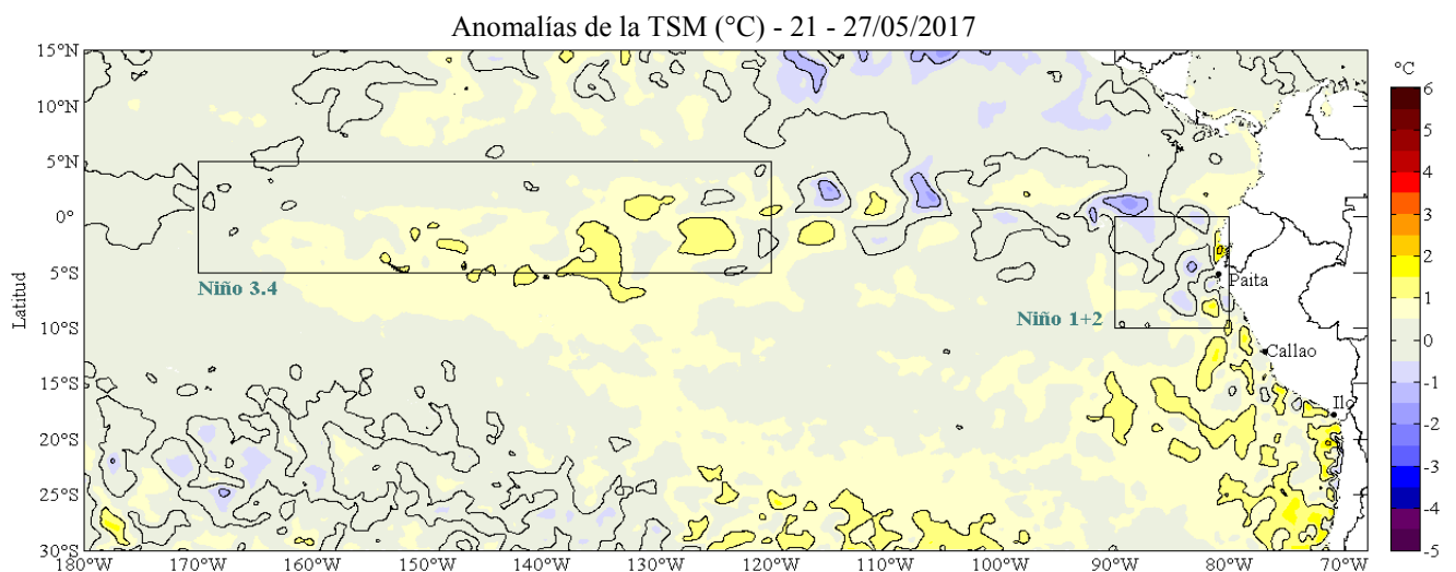
Figura 2. Anomalías promedio de la temperatura superficial del mar ( ^{\circ}\text{C} ) en el océano Pacífico tropical para la semana del 21 al 27 de mayo de 2017. Las regiones Niño 3.4 y Niño 1+2 en los sectores central y oriental del océano, respectivamente, están delimitadas con una línea de color gris. Datos: OSTIA-UKMO-L4-GLOB-v2.0 (UK Met Office, 2012; Donlon et al, 2012) disponible en https://podaac.jpl.nasa.gov/dataset/OSTIA-UKMO-L4-GLOB-v2.0 . Las anomalías se calcularon con respecto de la climatología para el período 2007-2016. Procesamiento: IMARPE.
