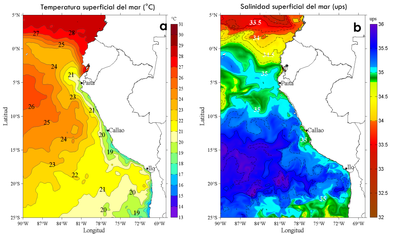
Figura 1. Distribución espacial promedio de: a) Temperatura Superficial del Mar ( ^{\circ}\text{C} ) y b) Salinidad Superficial del Mar, para la semana del 21 al 27 de mayo de 2017 en el océano Pacífico tropical oriental. Datos: OSTIA-UKMO-L4-GLOB-v2.0 (UK Met Office, 2012; Donlon et al, 2012) disponible en https://podaac.jpl.nasa.gov/dataset/OSTIA-UKMO-L4-GLOB-v2.0 para (a) y del Hybrid Coordinate Ocean Model (HYCOM; Halliwell et al., 1998; 2000; Bleck, 2001) para (b). Las escalas de colores de la temperatura como de la salinidad superficial del mar se presentan a la derecha de cada gráfico. Procesamiento: LHF/AFIOF/DGIOCC/IMARPE.
