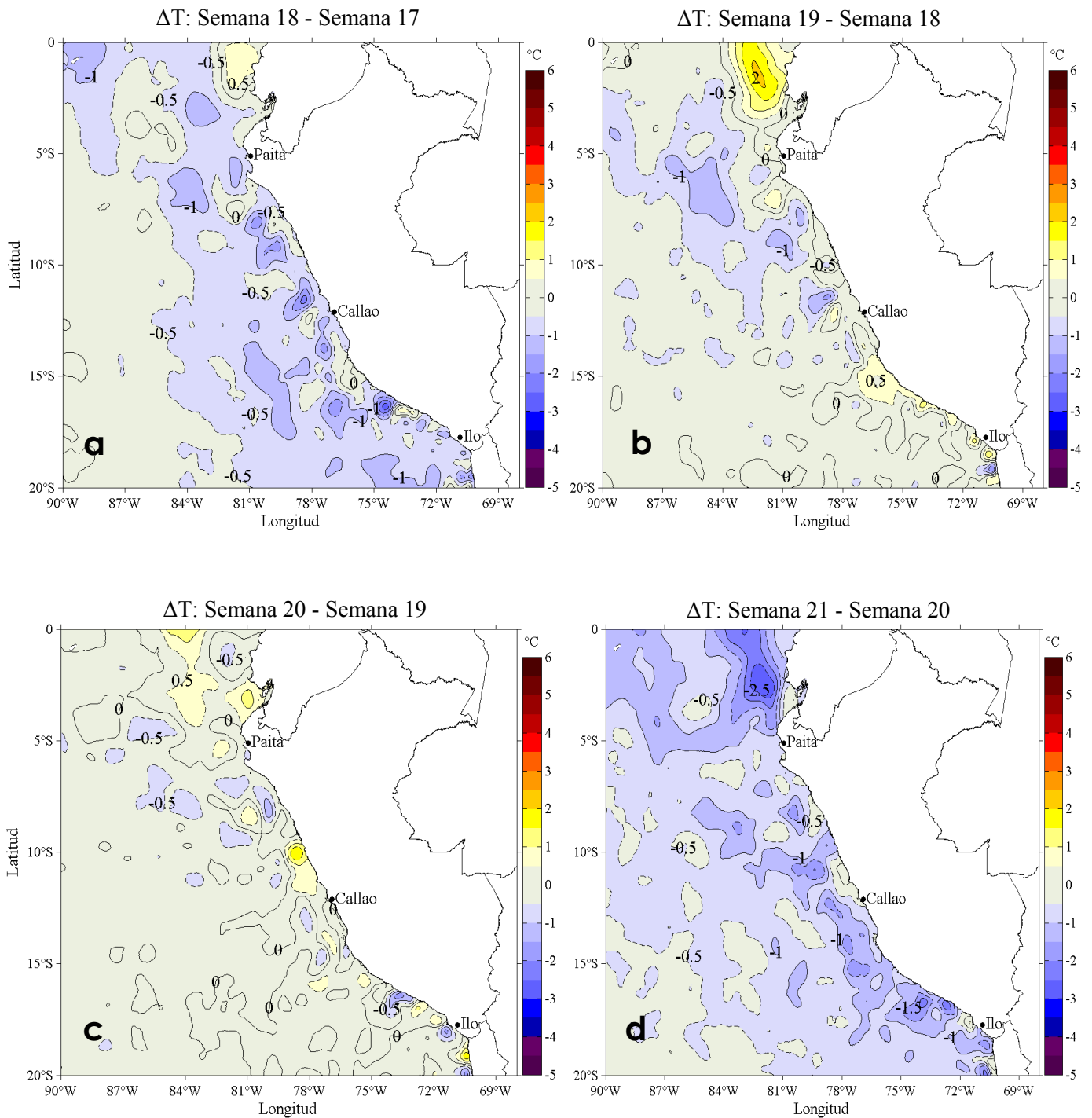
Figura 3. Variación semanal de la temperatura superficial del mar promedio ( ^{\circ}\text{C} ) en el océano Pacífico tropical oriental entre: a) décimo octava (30 de abril-06 de mayo) y décimo séptima (23-29 de abril) semana, b) décimo novena (07-13 de mayo) y décimo octava (30 de abril-06 de mayo) semana, c) vigésima (14-20 de mayo) y décimo novena (07-13 de mayo) semana, y d) vigésima primera (21-27 de mayo) y vigésima (14-20 de mayo) semana del presente año.
