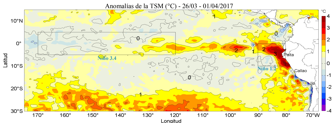
Figura 2. Anomalías promedio de la temperatura superficial del mar (°C) en el océano Pacífico tropical para la semana del 26 de marzo al 01 de abril de 2017. Las regiones Niño 3.4 y Niño 1+2 en los sectores central y oriental del océano, respectivamente, están delimitadas con una línea de color gris. Datos: AVHRR Global Reyn_SmithOiv2R (Reynolds, et. al., 2007) de CMB/EMC/NCEP de la Administración Nacional del Océano y la Atmósfera (NOAA, en inglés). Las anomalías se calcularon con respecto de la climatología para el período 1982-2011. Procesamiento: IMARPE.
