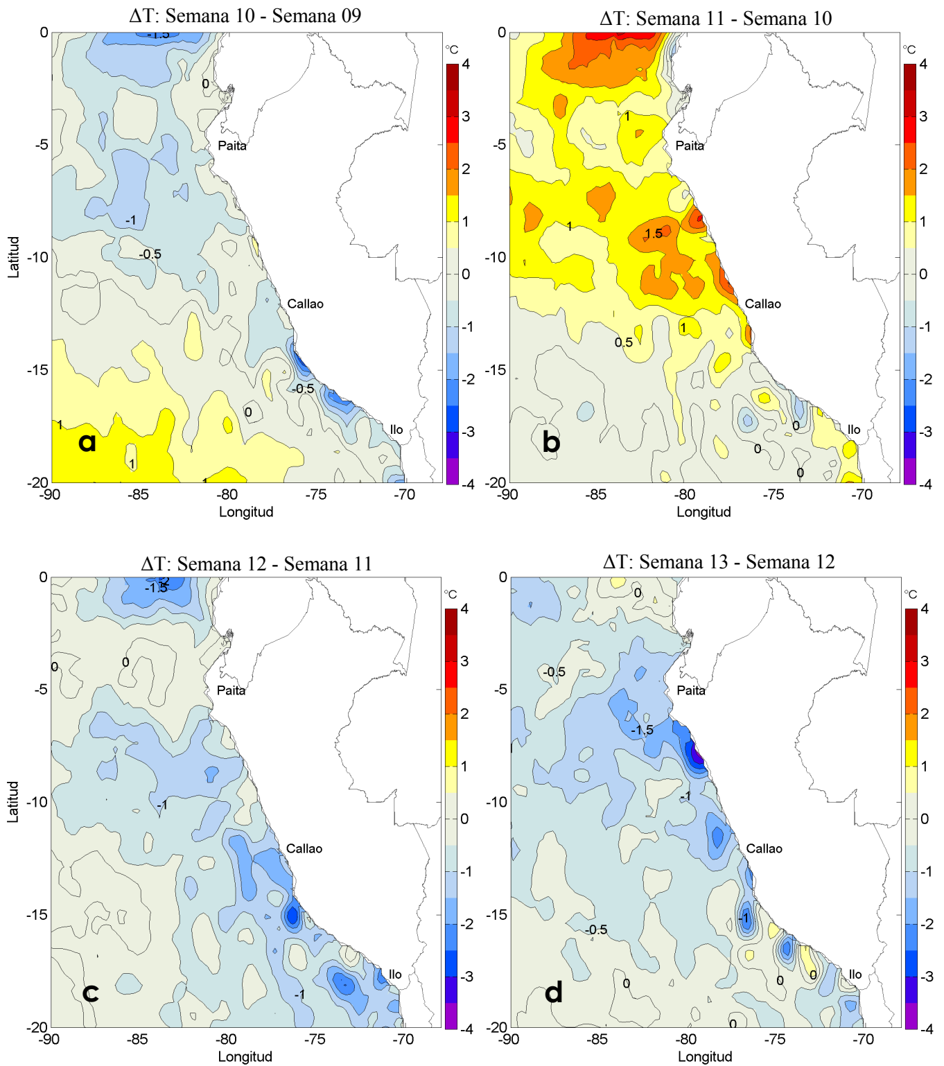
Figura 3. Variación de la anomalía promedio semanal de la temperatura superficial del mar ( ^{\circ}\text{C} ) en el océano Pacífico tropical oriental entre: a) la décima (05-11 de marzo) y novena (26 de febrero - 04 de marzo) semana, b) undécima (12-18 de marzo) y décima (05-11 de marzo) semana, c) la duodécima (19-25 de marzo) y undécima (12-18 de marzo) semana, d) décimo tercera (26 de marzo - 01 de abril) y duodécima (19-25 de marzo) semana del presente año.
