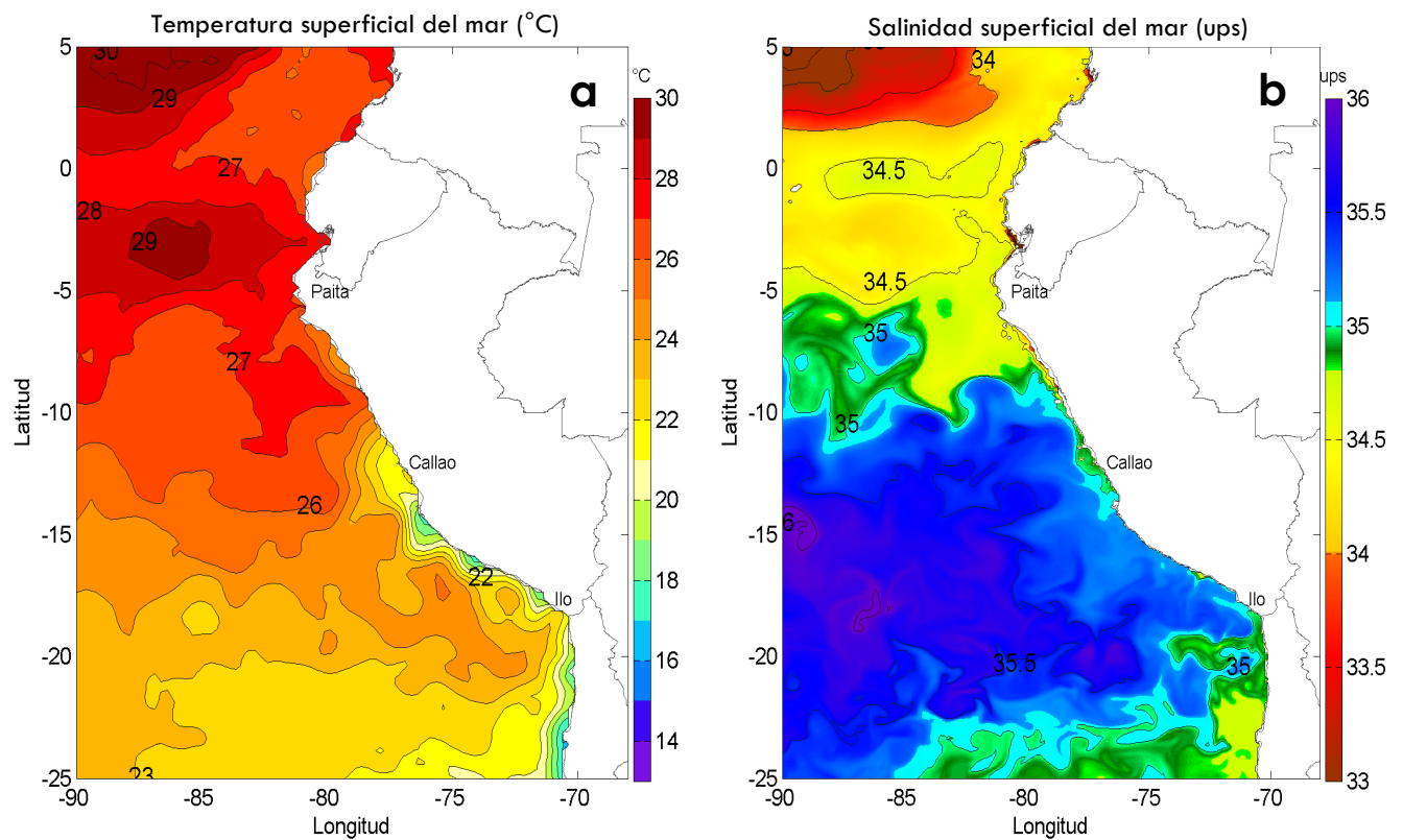
Figura 1. Distribución espacial promedio de: a) Temperatura Superficial del Mar (°C) y b) Salinidad Superficial del Mar, para la semana del 26 de marzo al 01 de abril de 2017 en el océano Pacífico tropical oriental. Datos: AVHRR v2 del Centro Nacional de Datos Climáticos de la Administración Nacional del Océano y la Atmósfera (NCDC/NOAA, según sus siglas en inglés) para (a) y del Hybrid Coordinate Ocean Model (HYCOM; Halliwell et al., 1998; 2000; Bleck, 2001) para (b). Las escalas de colores de la temperatura como de la salinidad superficial del mar se presentan a la derecha de cada gráfico. Procesamiento: LHFM/AFIOF/DGIOCC/IMARPE.
