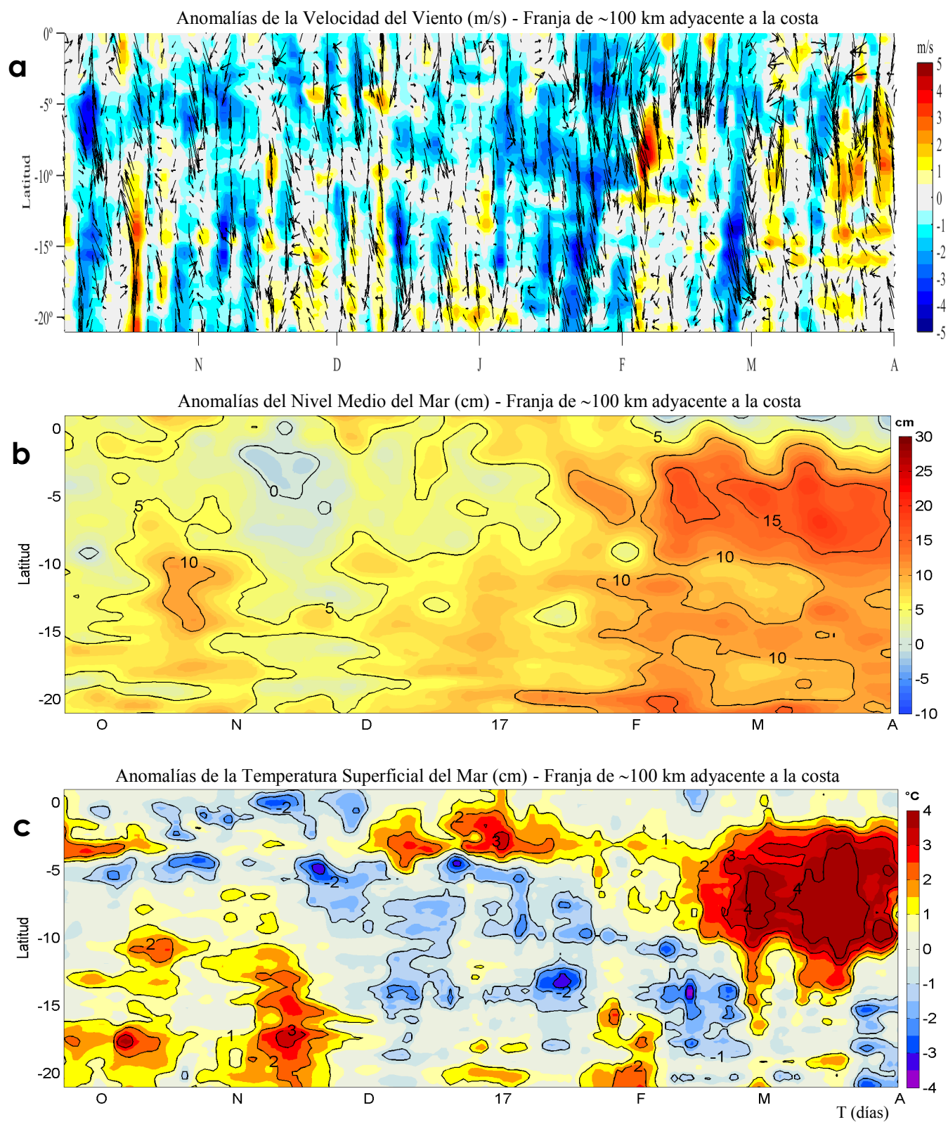
Figura 4. Evolución de las anomalías diarias de: a) velocidad del viento (m/s), b) nivel medio del mar (cm), c) temperatura superficial del mar (°C) para el último semestre actualizado al 01 de abril de 2017. Datos: de IFREMER/CERSAT para (a), del Servicio de Monitoreo del Ambiente Marino Copernicus (CMEMS, según sus siglas en inglés) para (b) del satélite AVHRR v2 del Centro Nacional de Datos Climáticos de la Administración Nacional del Océano y la Atmósfera (NCDC/NOAA, según sus siglas en inglés) para (c). Las anomalías fueron calculadas para una franja de 100 km adyacente a la costa entre el ecuador y 21°S según los promedios climatológicos diarios de 2000-2014 para (a), de 1993-2013 para (b) y de 1982-2011 para (c). La barra de colores a la derecha muestra la escala de las anomalías en cada caso. Procesamiento: LHF/AFIOF/DGIOCC/IMARPE.
