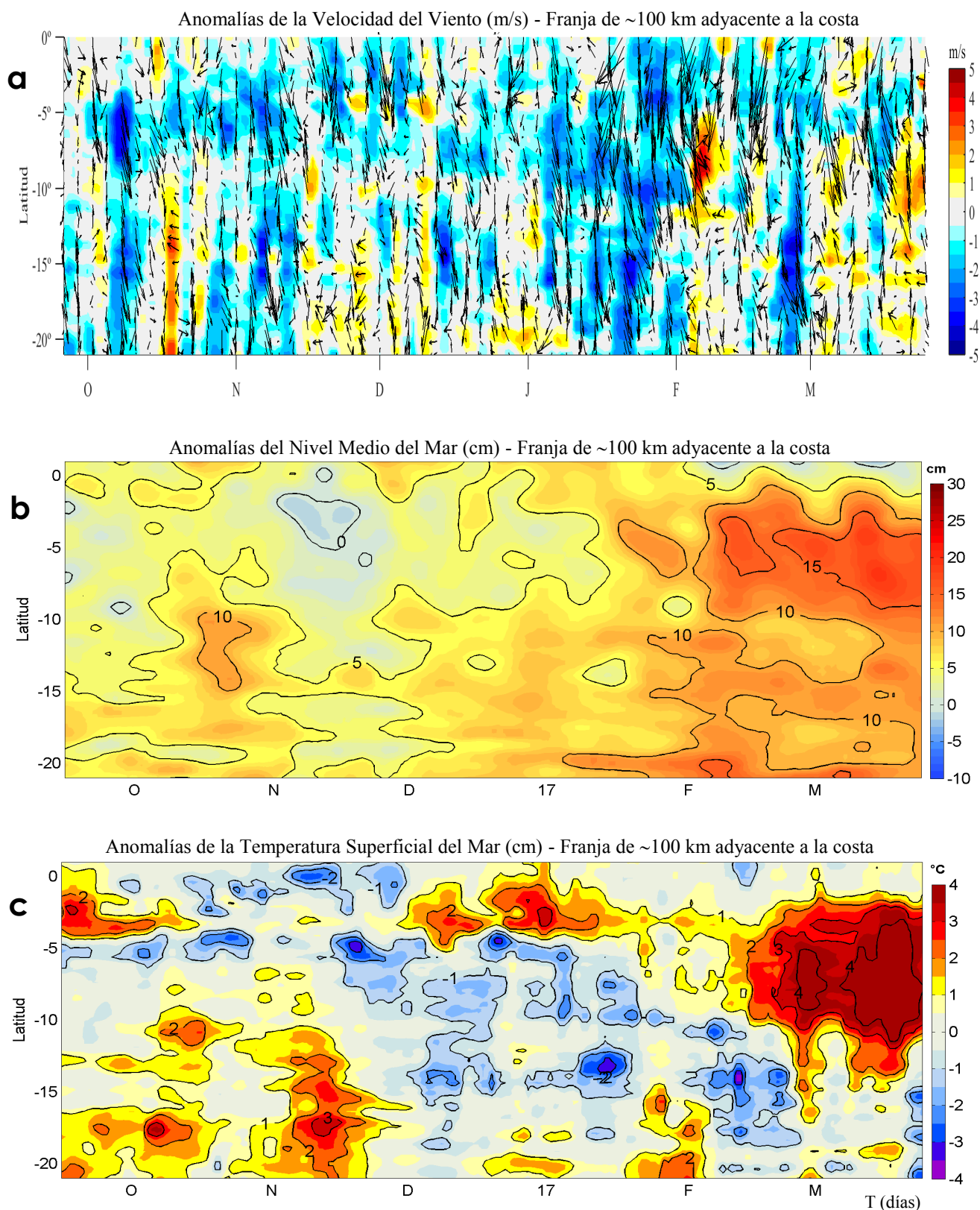
Figura 4. Evolución de las anomalías diarias de: a) velocidad del viento (m/s), b) nivel medio del mar (cm), c) temperatura superficial del mar (°C) para el último semestre actualizado al 25 de marzo de 2017. Datos: de IFREMER/CERSAT para (a), del Servicio de Monitoreo del Ambiente Marino Copernicus (CMEMS, según sus siglas en inglés) para (b) del satélite AVHRR v2 del Centro Nacional de Datos Climáticos de la Administración Nacional del Océano y la Atmósfera (NCDC/NOAA, según sus siglas en inglés) para (c). Las anomalías fueron calculadas para una franja de 100 km adyacente a la costa entre el ecuador y 21°S según los promedios climatológicos diarios de 2000-2014 para (a), de 1993-2013 para (b) y de 1982-2011 para (c). La barra de colores a la derecha muestra la escala de las anomalías en cada caso. Procesamiento: LHFM/AFIOF/DGIOCC/IMARPE.
