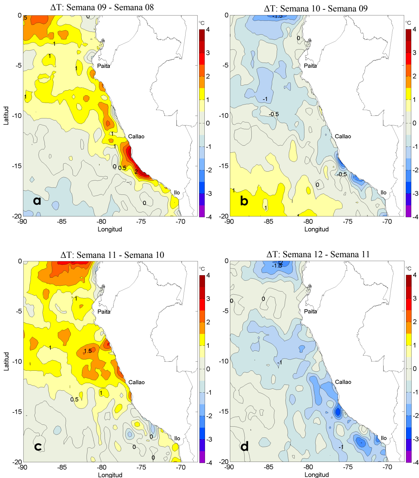
Figura 3. Variación de la anomalía promedio semanal de la temperatura superficial del mar ( ^{\circ}\text{C} ) en el océano Pacífico tropical oriental entre: a) la novena (26 de febrero-04 de marzo) y la octava (19-25 de febrero) semana, b) la décima (05-11 de marzo) y la novena (26 de febrero-04 de marzo) semana, c) la undécima (12-18 de marzo) y la décima (05-11 de marzo) semana, d) la duodécima (19-25 de marzo) y undécima (12-18 de marzo) semana del presente año.
