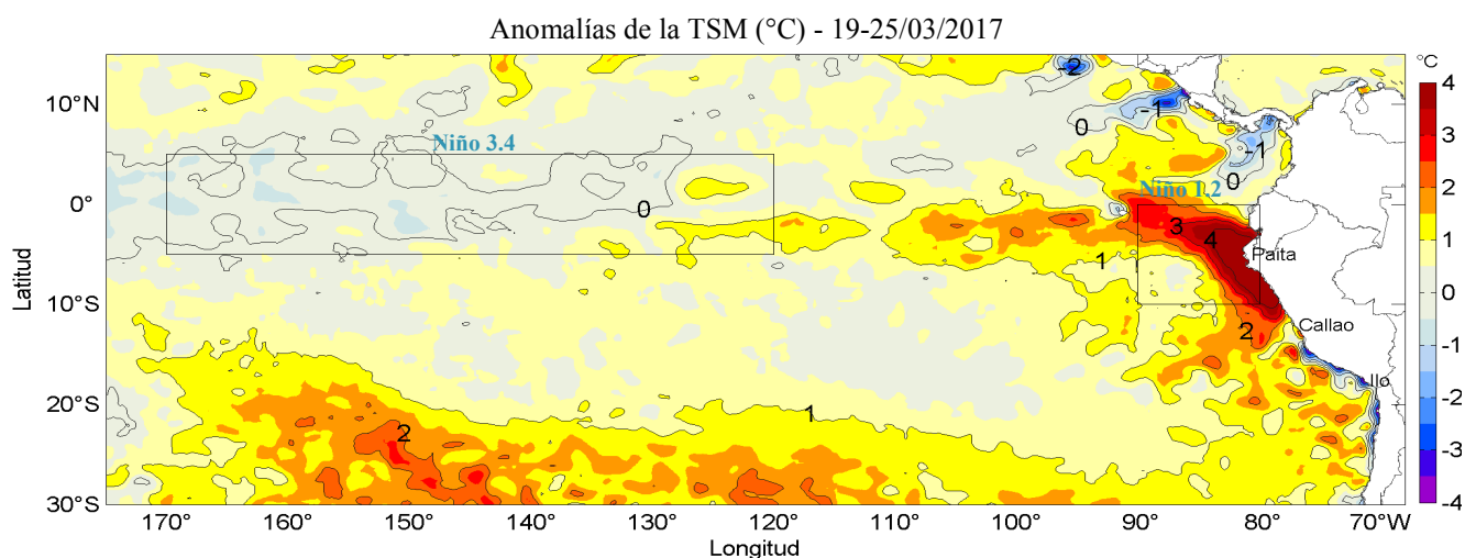
Figura 2. Anomalías promedio de la temperatura superficial del mar (°C) en el océano Pacífico tropical para la semana del 19 al 25 de marzo de 2017. Las regiones Niño 3.4 y Niño 1+2 en los sectores central y oriental del océano, respectivamente, están delimitadas con una línea de color gris. Datos: AVHRR Global Reyn_SmithOIv2R (Reynolds, et. al., 2007) de CMB/EMC/NCEP de la Administración Nacional del Océano y la Atmósfera (NOAA, en inglés). Las anomalías se calcularon con respecto de la climatología para el período 1982-2011. Procesamiento: IMARPE.
