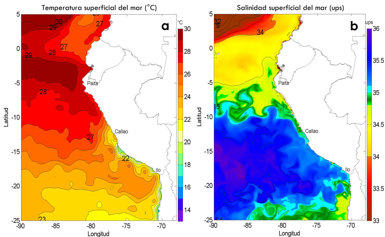
Figura 1. Distribución espacial promedio de: a) Temperatura Superficial del Mar (°C) y b) Salinidad Superficial del Mar, para la semana del 19 al 25 de marzo de 2017 en el océano Pacífico tropical oriental. Datos: AVHRR v2 del Centro Nacional de Datos Climáticos de la Administración Nacional del Océano y la Atmósfera (NCDC/NOAA, según sus siglas en inglés) para (a) y del Hybrid Coordinate Ocean Model (HYCOM; Halliwell et al., 1998; 2000; Bleck, 2001) para (b). Las escalas de colores de la temperatura como de la salinidad superficial del mar se presentan a la derecha de cada gráfico. Procesamiento: LHF/M/AFIOF/DGIOCC/IMARPE.
