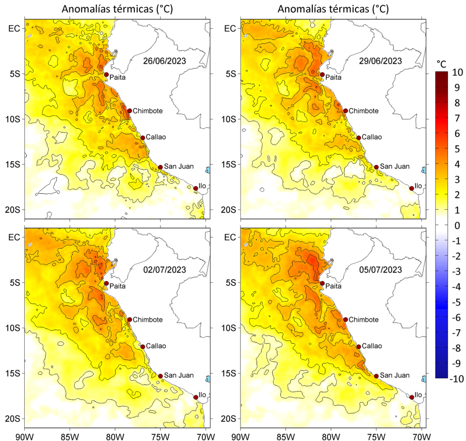
Figura 3. Anomalías de la temperatura superficial del mar ( ^{\circ}\text{C} ) para el a) 26, b) 29 de junio, c) 02 y d) 05 de julio de 2023. Las anomalías se calcularon respecto de la climatología para el periodo 2007-2016. Datos: OSTIA-UKMO-L4-GLOB-v2.0 (UK Met Office, 2012; Donlon et al, 2012).
