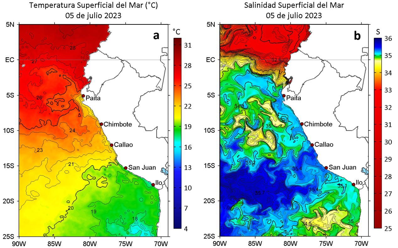
Figura 2. a) Temperatura superficial del mar ( ^{\circ}\text{C} ) y b) Salinidad superficial del mar para el 05 de julio de 2023. Datos: OSTIA-UKMO-L4-GLOB-v2.0 (UK Met Office, 2012; Donlon et al, 2012) y del GLOBAL_ANALYSISFORECAST_PHY_001_024 (Lellouche, J. M. et al, 2013), respectivamente.
