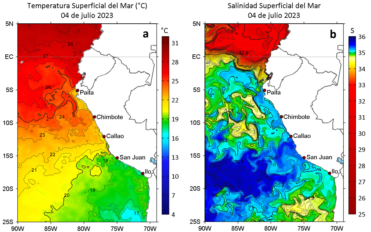
Figura 2. a) Temperatura superficial del mar ( ^{\circ}\text{C} ) y b) Salinidad superficial del mar para el 04 de julio de 2023. Datos: OSTIA-UKMO-L4-GLOB-v2.0 (UK Met Office, 2012; Donlon et al, 2012) y del GLOBAL_ANALYSISFORECAST_PHY_001_024 (Lellouche, J. M. et al, 2013), respectivamente.
