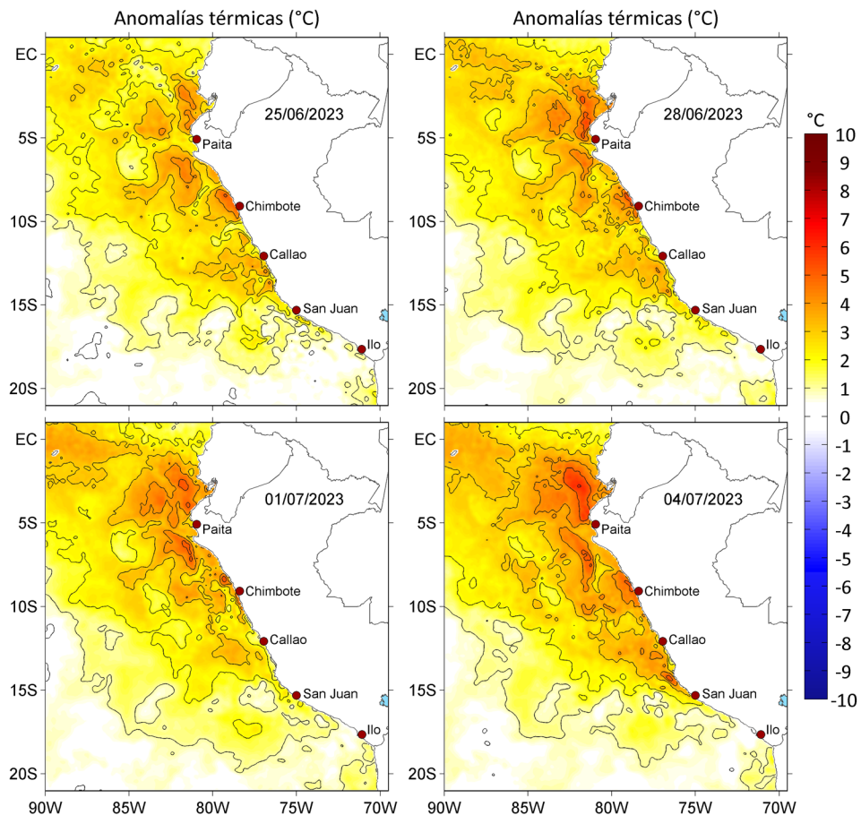
Figura 3. Anomalías de la temperatura superficial del mar ( ^{\circ}\text{C} ) para el a) 25, b) 28 de junio, c) 01 y d) 04 de julio de 2023. Las anomalías se calcularon respecto de la climatología para el periodo 2007-2016. Datos: OSTIA-UKMO-L4-GLOB-v2.0 (UK Met Office, 2012; Donlon et al, 2012).
