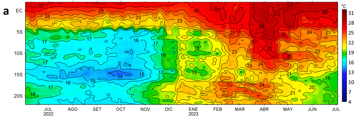
Anomalías de la Temperatura Superficial del mar (°C), franja costera de 60 m.n. 02 de junio 2022 - 03 de julio 2023
