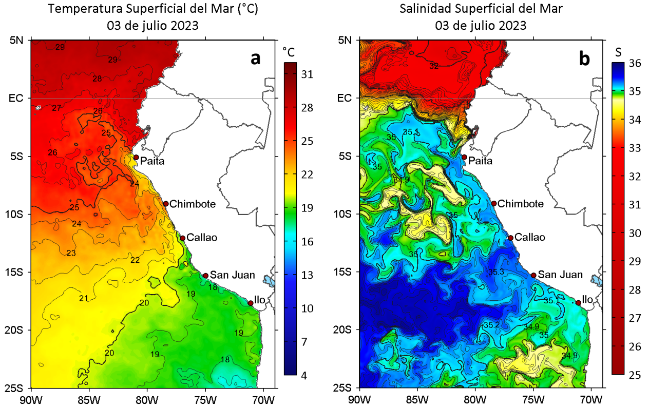
Figura 2. a) Temperatura superficial del mar ( ^{\circ}\text{C} ) y b) Salinidad superficial del mar para el 03 de julio de 2023. Datos: OSTIA-UKMO-L4-GLOB-v2.0 (UK Met Office, 2012; Donlon et al, 2012) y del GLOBAL_ANALYSISFORECAST_PHY_001_024 (Lellouche, J. M. et al, 2013), respectivamente.
