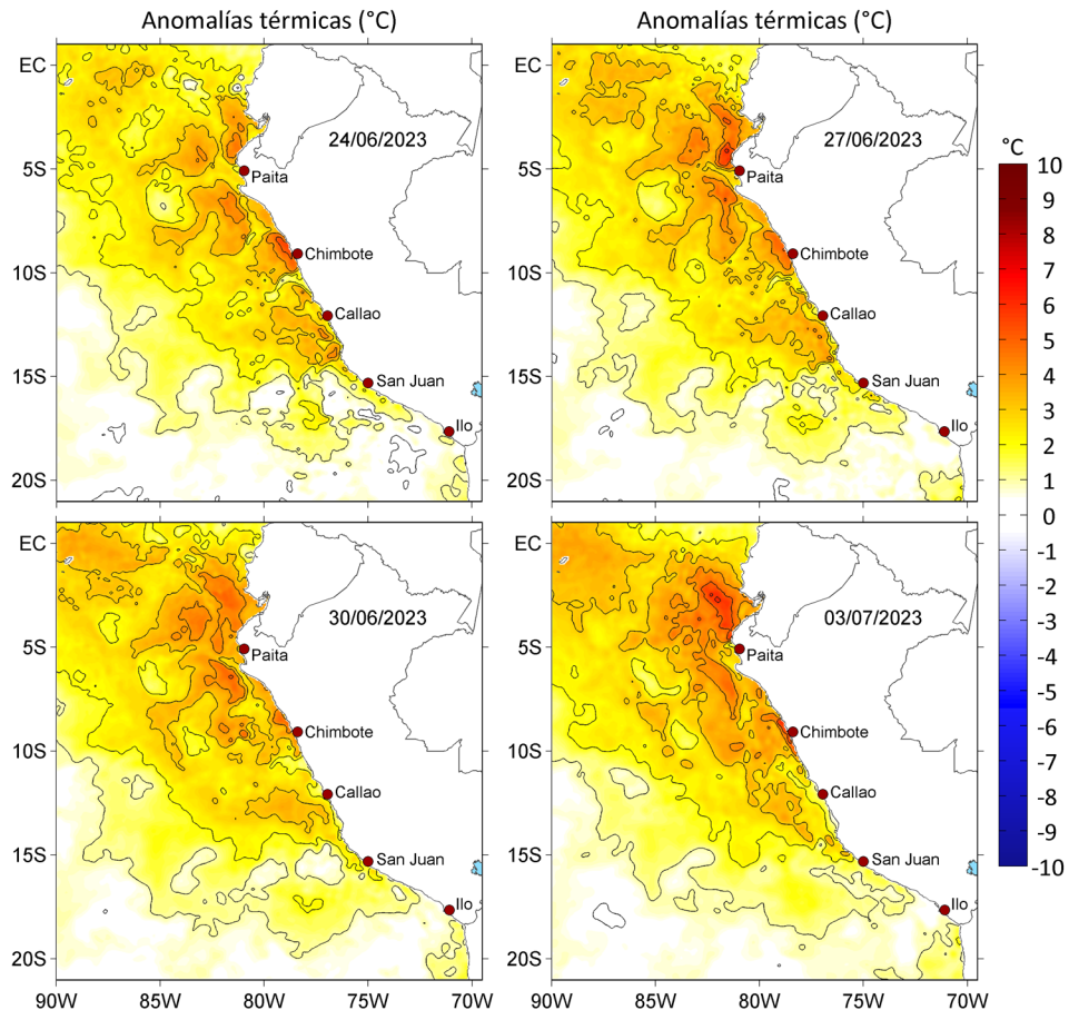
Figura 3. Anomalías de la temperatura superficial del mar ( ^{\circ}\text{C} ) para el a) 24, b) 27, c) 30 de junio y d) 03 de julio de 2023. Las anomalías se calcularon respecto de la climatología para el periodo 2007-2016. Datos: OSTIA-UKMO-L4-GLOB-v2.0 (UK Met Office, 2012; Donlon et al, 2012).
