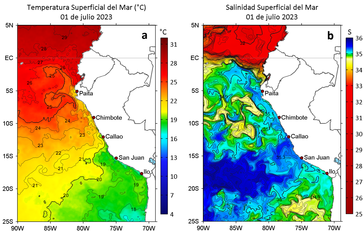
Figura 2. a) Temperatura superficial del mar ( ^{\circ}\text{C} ) y b) Salinidad superficial del mar para el 01 de julio de 2023. Datos: OSTIA-UKMO-L4-GLOB-v2.0 (UK Met Office, 2012; Donlon et al, 2012) y del GLOBAL_ANALYSISFORECAST_PHY_001_024 (Lellouche, J. M. et al, 2013), respectivamente.
