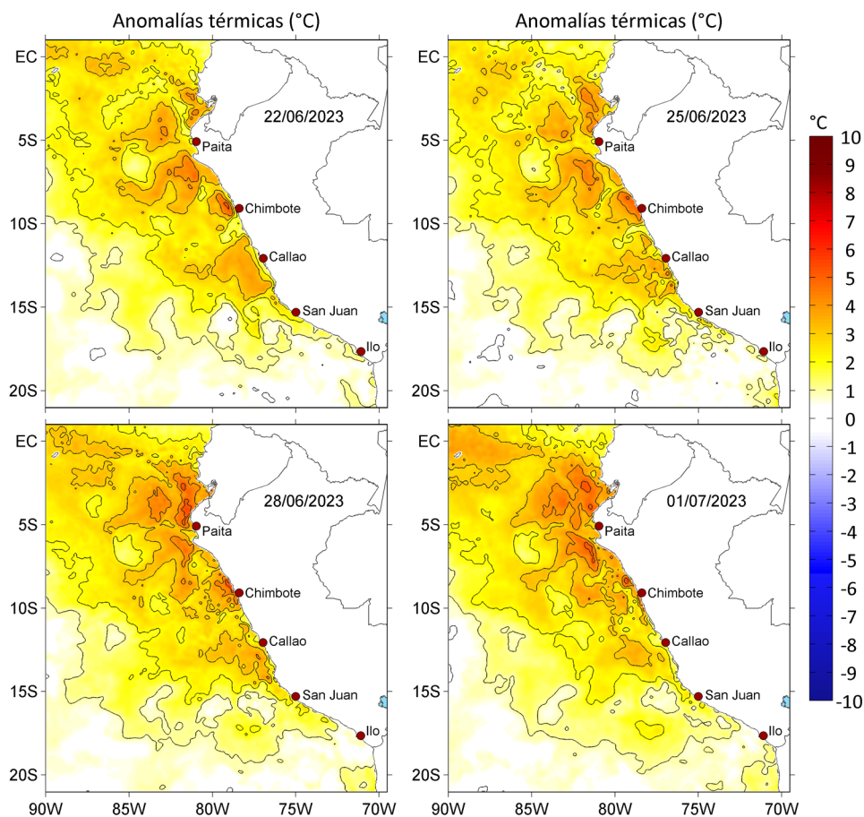
Figura 3. Anomalías de la temperatura superficial del mar ( ^{\circ}\text{C} ) para el a) 22, b) 25, c) 28 de junio y d) 01 de julio de 2023. Las anomalías se calcularon respecto de la climatología para el periodo 2007-2016. Datos: OSTIA-UKMO-L4-GLOB-v2.0 (UK Met Office, 2012; Donlon et al, 2012).
