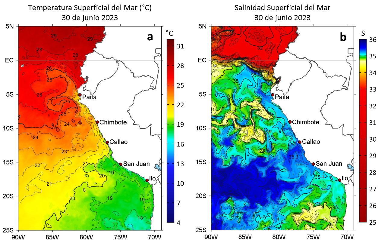
Figura 2. a) Temperatura superficial del mar ( ^{\circ}\text{C} ) y b) Salinidad superficial del mar para el 30 de junio de 2023. Datos: OSTIA-UKMO-L4-GLOB-v2.0 (UK Met Office, 2012; Donlon et al, 2012) y del GLOBAL_ANALYSISFORECAST_PHY_001_024 (Lellouche, J. M. et al, 2013), respectivamente.
