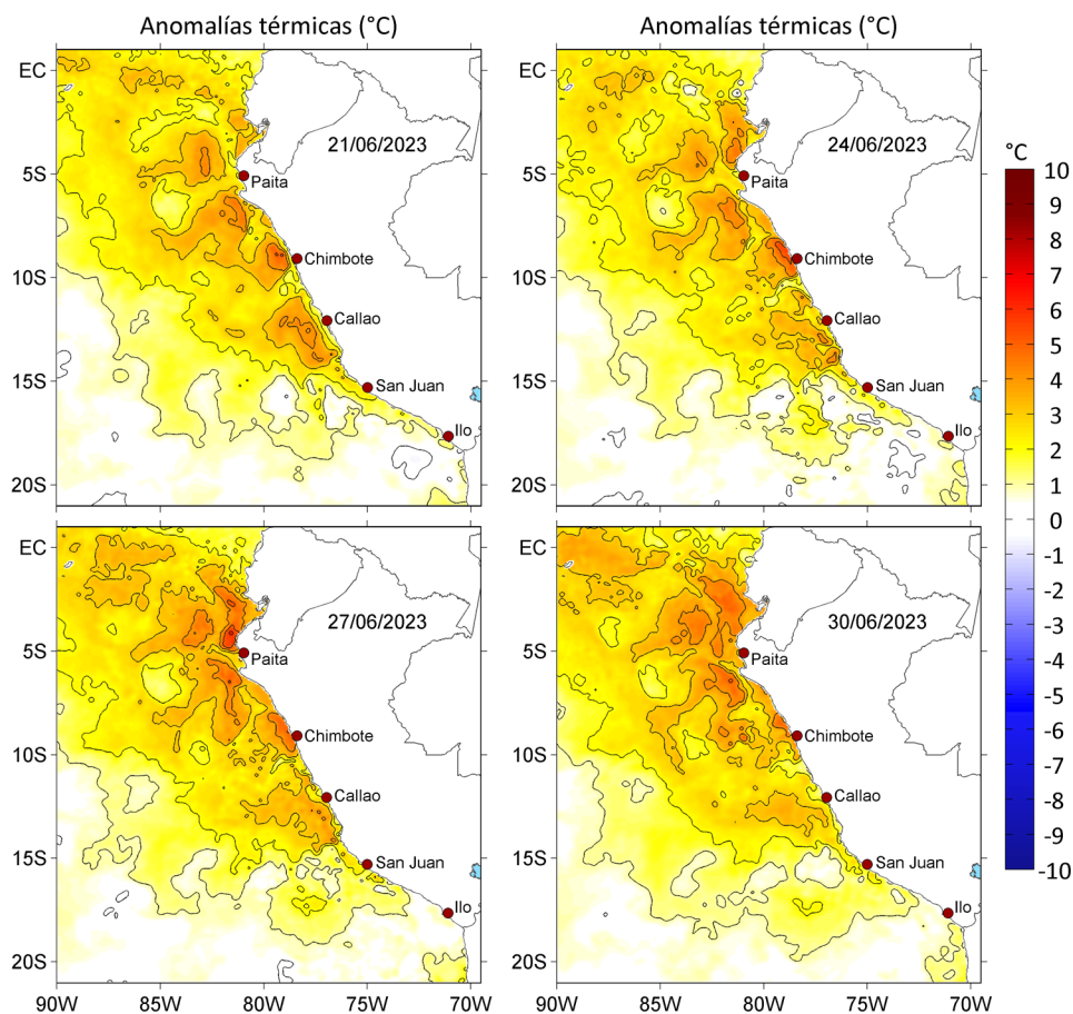
Figura 3. Anomalías de la temperatura superficial del mar ( ^{\circ}\text{C} ) para el a) 21, b) 24, c) 27 y d) 30 de junio de 2023. Las anomalías se calcularon respecto de la climatología para el periodo 2007-2016. Datos: OSTIA-UKMO-L4-GLOB-v2.0 (UK Met Office, 2012; Donlon et al, 2012).
