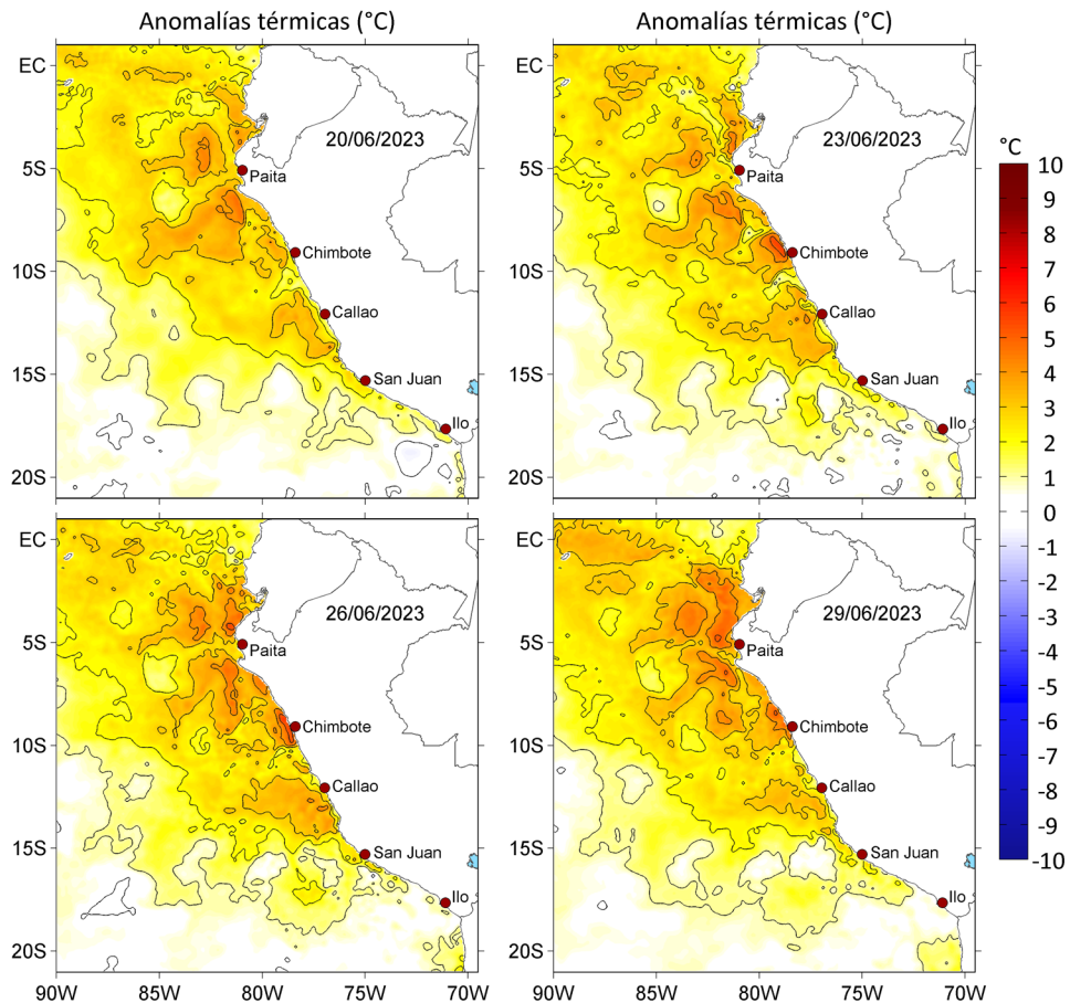
Figura 3. Anomalías de la temperatura superficial del mar ( ^{\circ}\text{C} ) para el a) 20, b) 23, c) 26 y d) 29 de junio de 2023. Las anomalías se calcularon respecto de la climatología para el periodo 2007-2016. Datos: OSTIA-UKMO-L4-GLOB-v2.0 (UK Met Office, 2012; Donlon et al, 2012).
