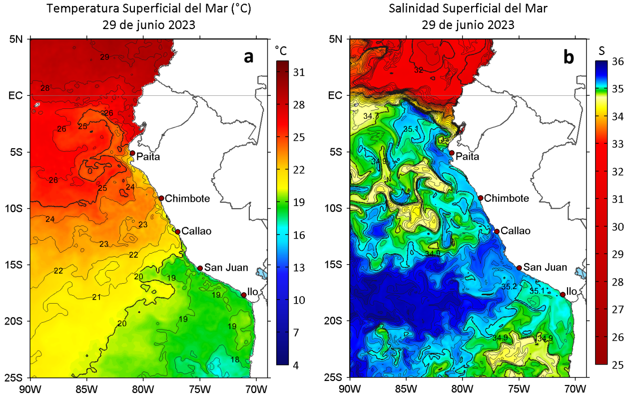
Figura 2. a) Temperatura superficial del mar ( ^{\circ}\text{C} ) y b) Salinidad superficial del mar para el 29 de junio de 2023. Datos: OSTIA-UKMO-L4-GLOB-v2.0 (UK Met Office, 2012; Donlon et al, 2012) y del GLOBAL_ANALYSISFORECAST_PHY_001_024 (Lellouche, J. M. et al, 2013), respectivamente.
