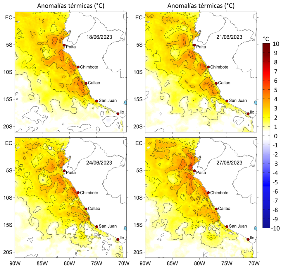
Figura 3. Anomalías de la temperatura superficial del mar ( ^{\circ}\text{C} ) para el a) 18, b) 21, c) 24 y d) 27 de junio de 2023. Las anomalías se calcularon respecto de la climatología para el periodo 2007-2016. Datos: OSTIA-UKMO-L4-GLOB-v2.0 (UK Met Office, 2012; Donlon et al, 2012).
