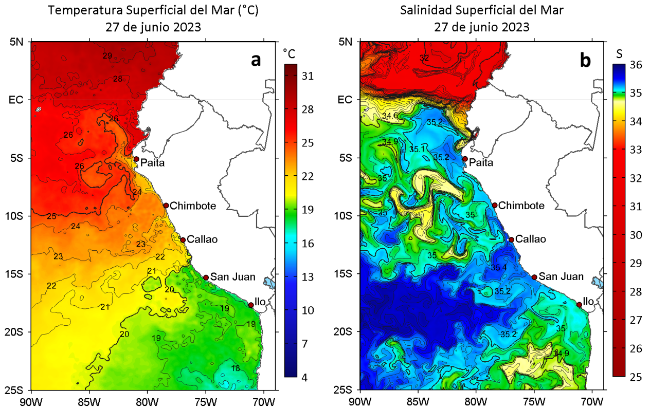
Figura 2. a) Temperatura superficial del mar ( ^{\circ}\text{C} ) y b) Salinidad superficial del mar para el 27 de junio de 2023. Datos: OSTIA-UKMO-L4-GLOB-v2.0 (UK Met Office, 2012; Donlon et al, 2012) y del GLOBAL_ANALYSISFORECAST_PHY_001_024 (Lellouche, J. M. et al, 2013), respectivamente.
