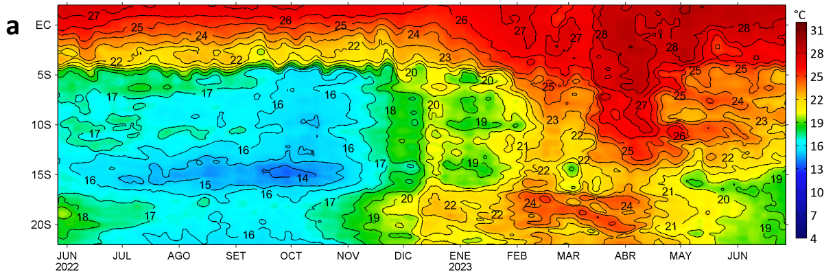
Anomalías de la Temperatura Superficial del mar (°C), franja costera de 60 m.n. 27 de mayo 2022 - 27 de junio 2023
