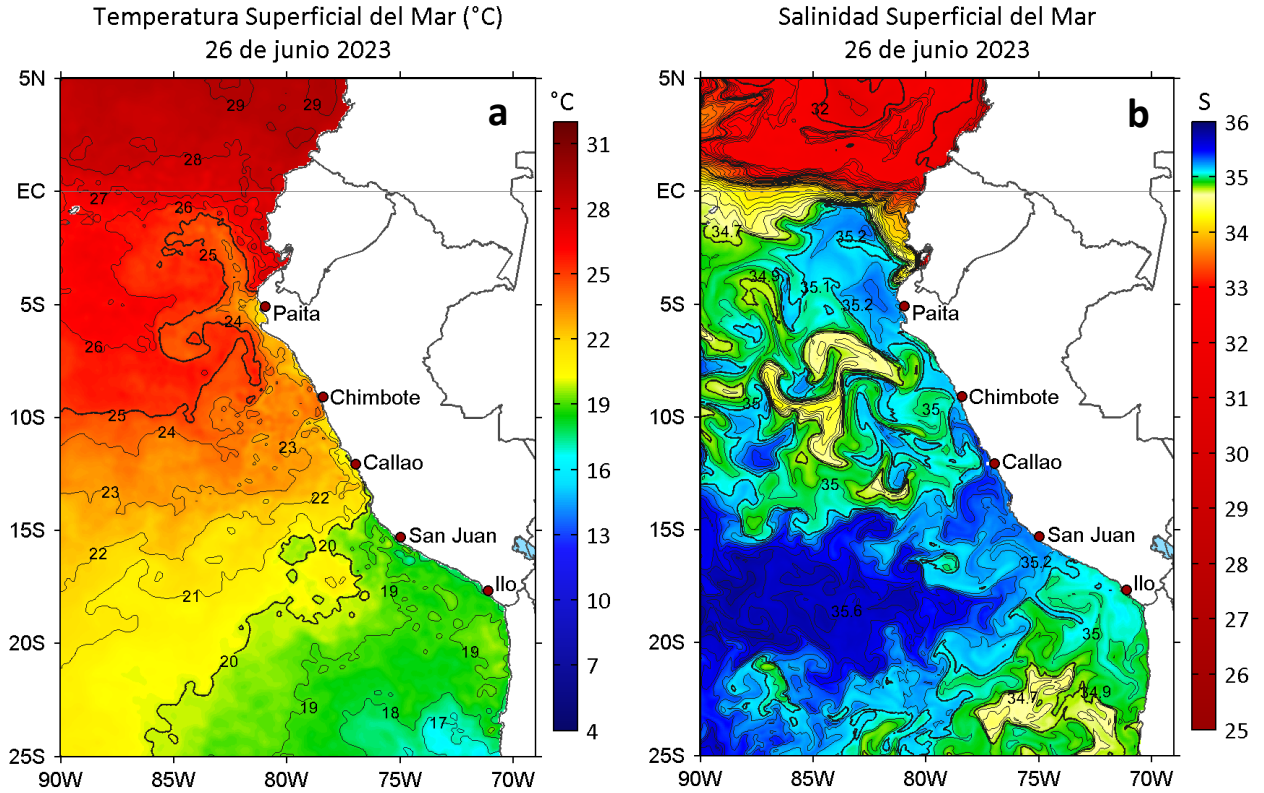
Figura 2. a) Temperatura superficial del mar ( ^{\circ}\text{C} ) y b) Salinidad superficial del mar para el 26 de junio de 2023. Datos: OSTIA-UKMO-L4-GLOB-v2.0 (UK Met Office, 2012; Donlon et al, 2012) y del GLOBAL_ANALYSISFORECAST_PHY_001_024 (Lellouche, J. M. et al, 2013), respectivamente.
