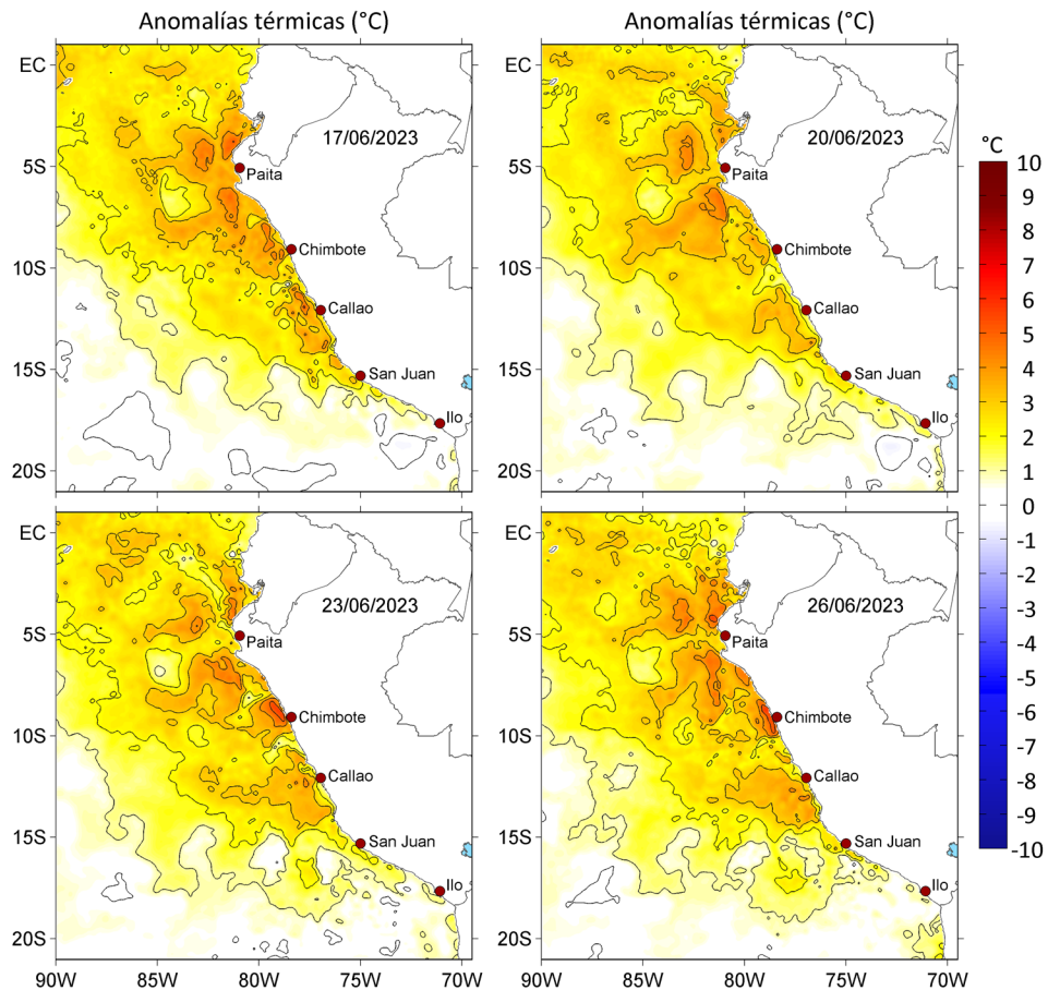
Figura 3. Anomalías de la temperatura superficial del mar ( ^{\circ}\text{C} ) para el a) 17, b) 20, c) 23 y d) 26 de junio de 2023. Las anomalías se calcularon respecto de la climatología para el periodo 2007-2016. Datos: OSTIA-UKMO-L4-GLOB-v2.0 (UK Met Office, 2012; Donlon et al, 2012).
