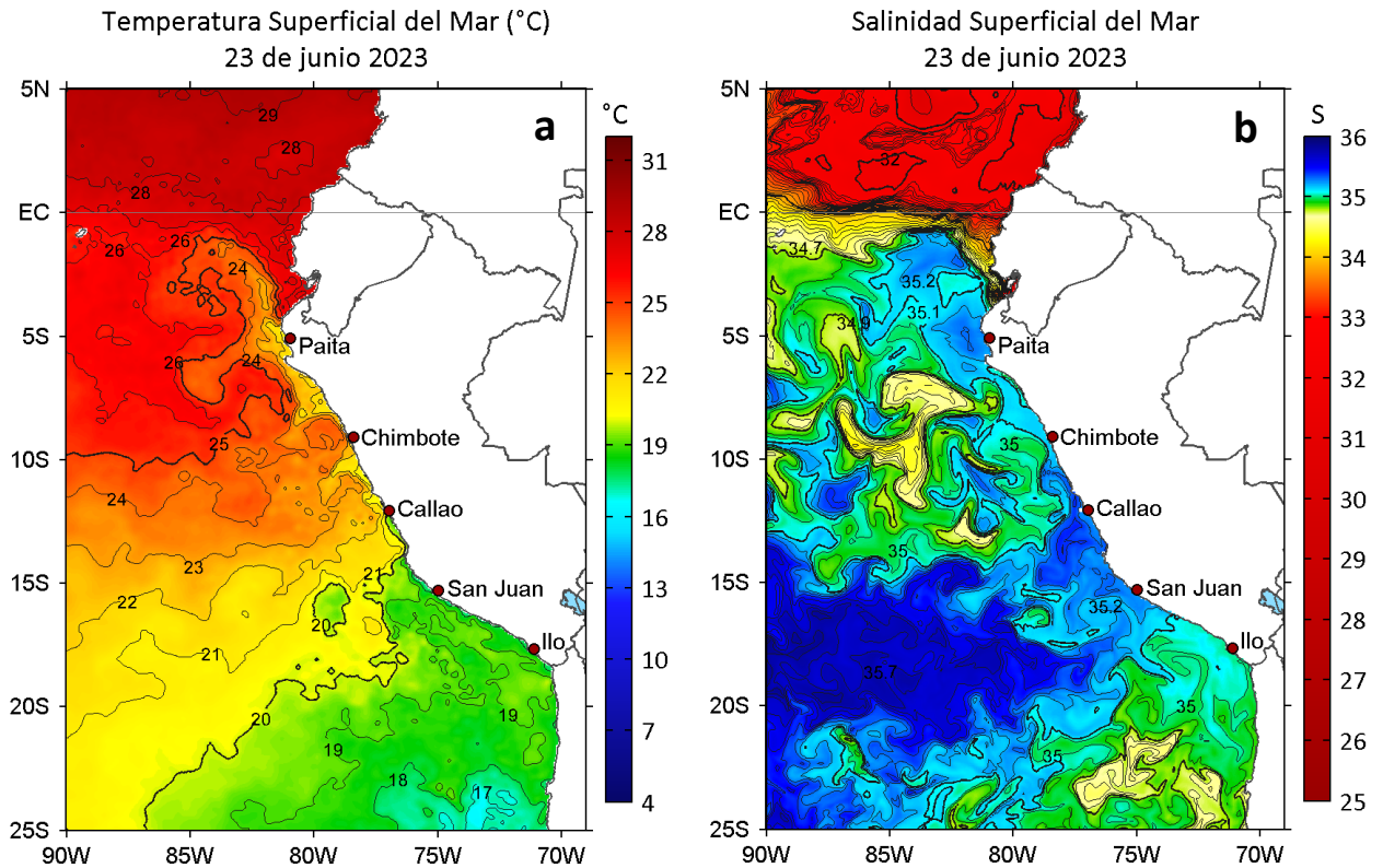
Figura 2. a) Temperatura superficial del mar (°C) y b) Salinidad superficial del mar para el 23 de junio de 2023. Datos: OSTIA-UKMO-L4-GLOB-v2.0 (UK Met Office, 2012; Donlon et al, 2012) y del GLOBAL_ANALYSISFORECAST_PHY_001_024 (Lellouche, J. M. et al, 2013), respectivamente.
