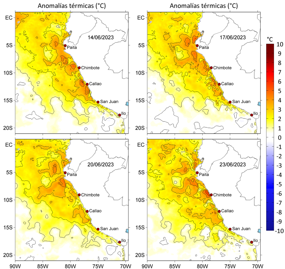
Figura 3. Anomalías de la temperatura superficial del mar (°C) para el a) 14, b) 17, c) 20 y d) 23 de junio de 2023. Las anomalías se calcularon respecto de la climatología para el periodo 2007-2016. Datos: OSTIA-UKMO-L4-GLOB-v2.0 (UK Met Office, 2012; Donlon et al, 2012).
