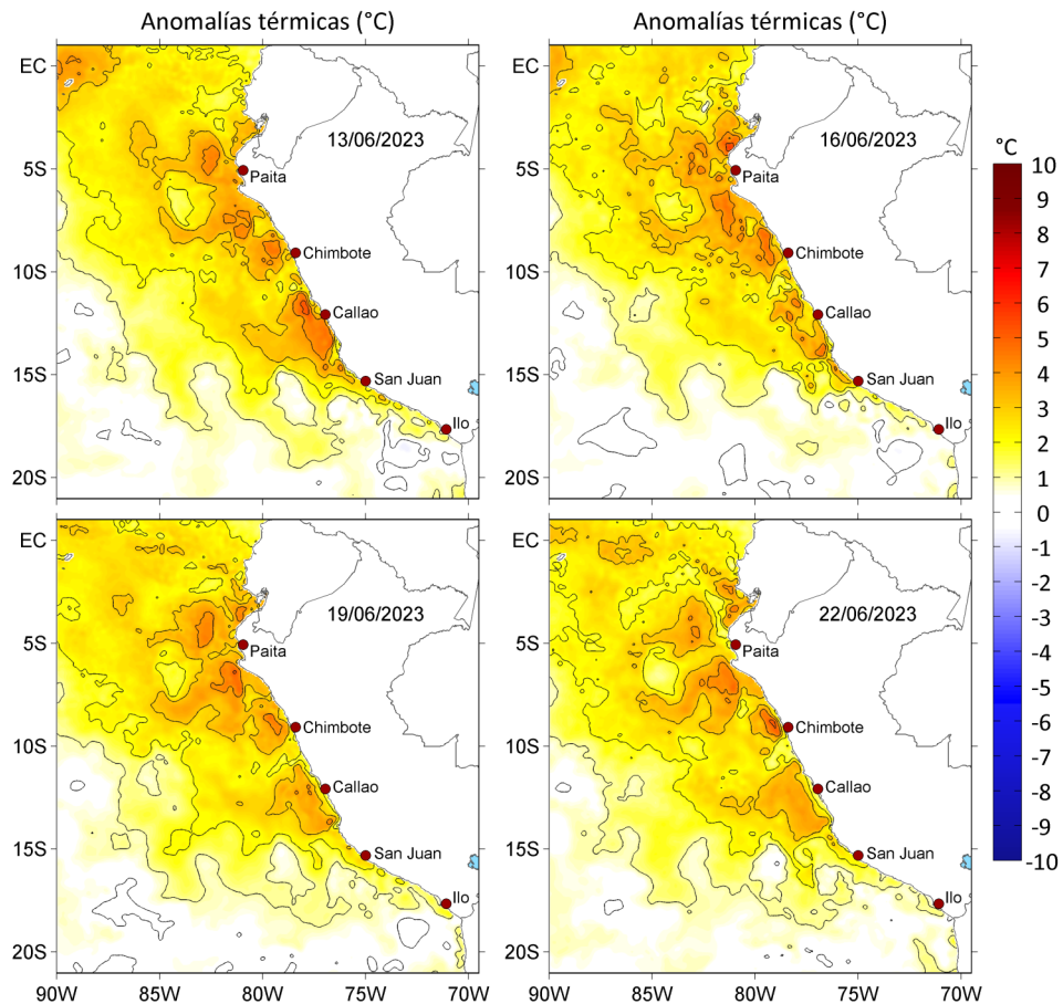
Figura 3. Anomalías de la temperatura superficial del mar ( ^{\circ}\text{C} ) para el a) 13, b) 16, c) 19 y d) 22 de junio de 2023. Las anomalías se calcularon respecto de la climatología para el periodo 2007-2016. Datos: OSTIA-UKMO-L4-GLOB-v2.0 (UK Met Office, 2012; Donlon et al, 2012).
