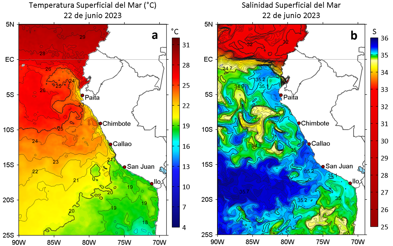
Figura 2. a) Temperatura superficial del mar ( ^{\circ}\text{C} ) y b) Salinidad superficial del mar para el 22 de junio de 2023. Datos: OSTIA-UKMO-L4-GLOB-v2.0 (UK Met Office, 2012; Donlon et al, 2012) y del GLOBAL_ANALYSISFORECAST_PHY_001_024 (Lellouche, J. M. et al, 2013), respectivamente.
