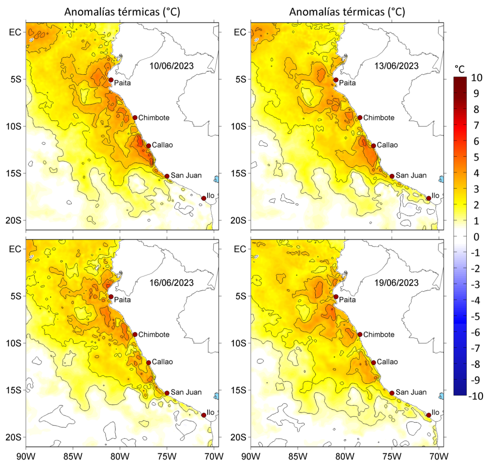
Figura 3. Anomalías de la temperatura superficial del mar ( ^{\circ}\text{C} ) para el a) 10, b) 13, c) 16 y d) 19 de junio de 2023. Las anomalías se calcularon respecto de la climatología para el periodo 2007-2016. Datos: OSTIA-UKMO-L4-GLOB-v2.0 (UK Met Office, 2012; Donlon et al, 2012).
