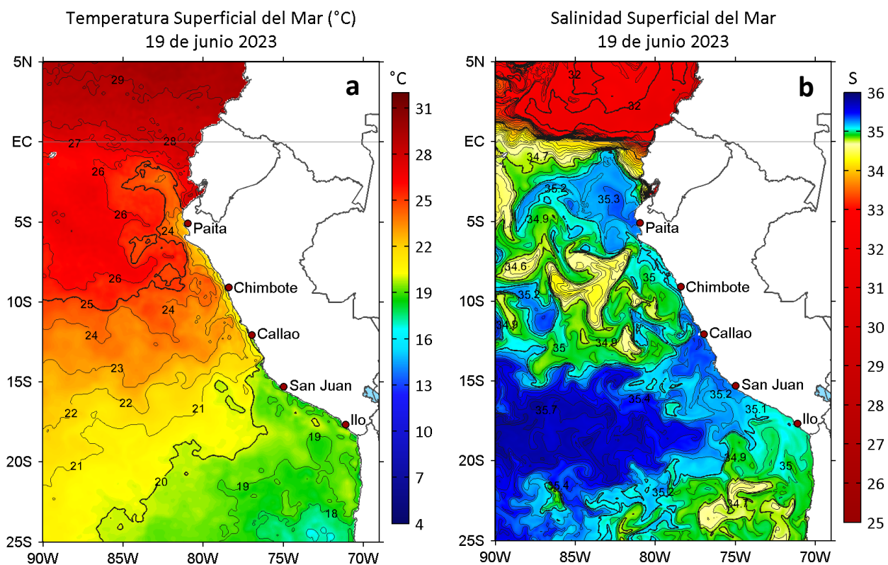
Figura 2. a) Temperatura superficial del mar ( ^{\circ}\text{C} ) y b) Salinidad superficial del mar para el 19 de junio de 2023. Datos: OSTIA-UKMO-L4-GLOB-v2.0 (UK Met Office, 2012; Donlon et al, 2012) y del GLOBAL_ANALYSISFORECAST_PHY_001_024 (Lellouche, J. M. et al, 2013), respectivamente.
