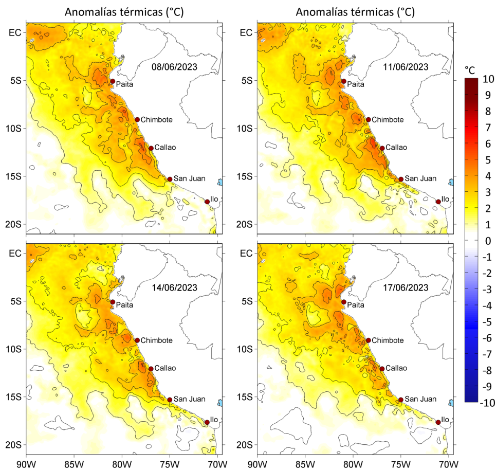
Figura 3. Anomalías de la temperatura superficial del mar ( ^{\circ}\text{C} ) para el a) 08, b) 11, c) 14 y d) 17 de junio de 2023. Las anomalías se calcularon respecto de la climatología para el periodo 2007-2016. Datos: OSTIA-UKMO-L4-GLOB-v2.0 (UK Met Office, 2012; Donlon et al, 2012).
