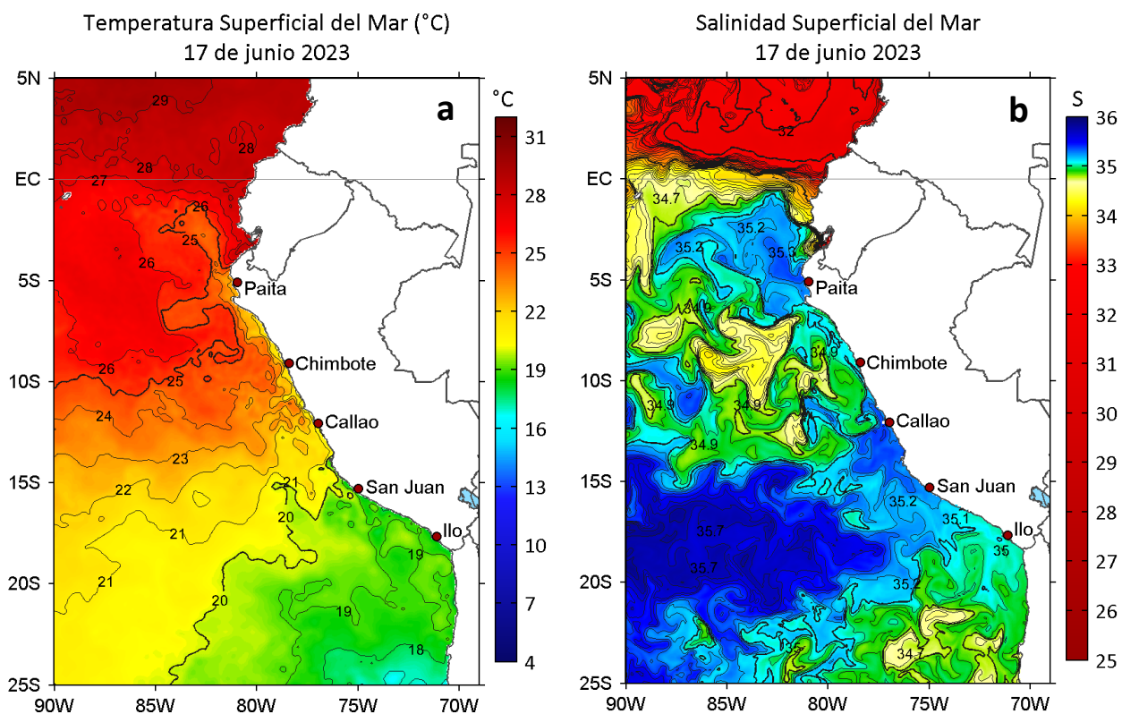
Figura 2. a) Temperatura superficial del mar ( ^{\circ}\text{C} ) y b) Salinidad superficial del mar para el 17 de junio de 2023. Datos: OSTIA-UKMO-L4-GLOB-v2.0 (UK Met Office, 2012; Donlon et al, 2012) y del GLOBAL_ANALYSISFORECAST_PHY_001_024 (Lellouche, J. M. et al, 2013), respectivamente.
