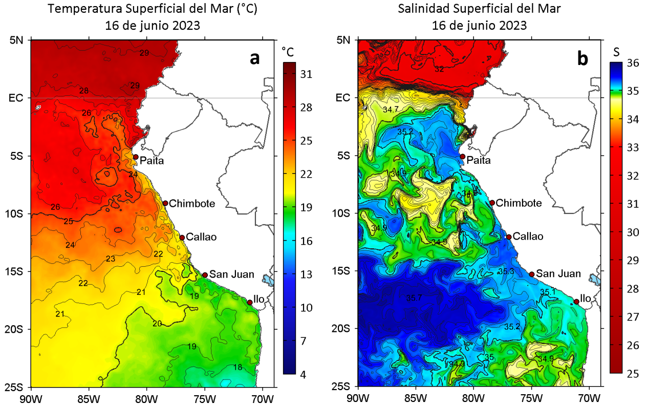
Figura 2. a) Temperatura superficial del mar ( ^{\circ}\text{C} ) y b) Salinidad superficial del mar para el 16 de junio de 2023. Datos: OSTIA-UKMO-L4-GLOB-v2.0 (UK Met Office, 2012; Donlon et al, 2012) y del GLOBAL_ANALYSISFORECAST_PHY_001_024 (Lellouche, J. M. et al, 2013), respectivamente.
