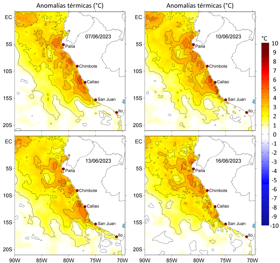
Figura 3. Anomalías de la temperatura superficial del mar ( ^{\circ}\text{C} ) para el a) 07, b) 10, c) 13 y d) 16 de junio de 2023. Las anomalías se calcularon respecto de la climatología para el periodo 2007-2016. Datos: OSTIA-UKMO-L4-GLOB-v2.0 (UK Met Office, 2012; Donlon et al, 2012).
