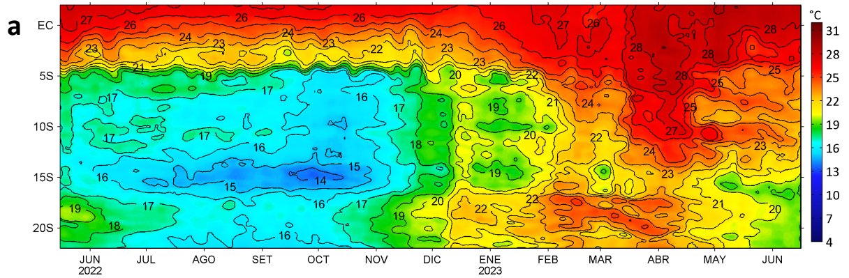
Anomalías de la Temperatura Superficial del mar (°C), franja costera de 60 m.n. 16 de mayo 2022 - 16 de junio 2023
