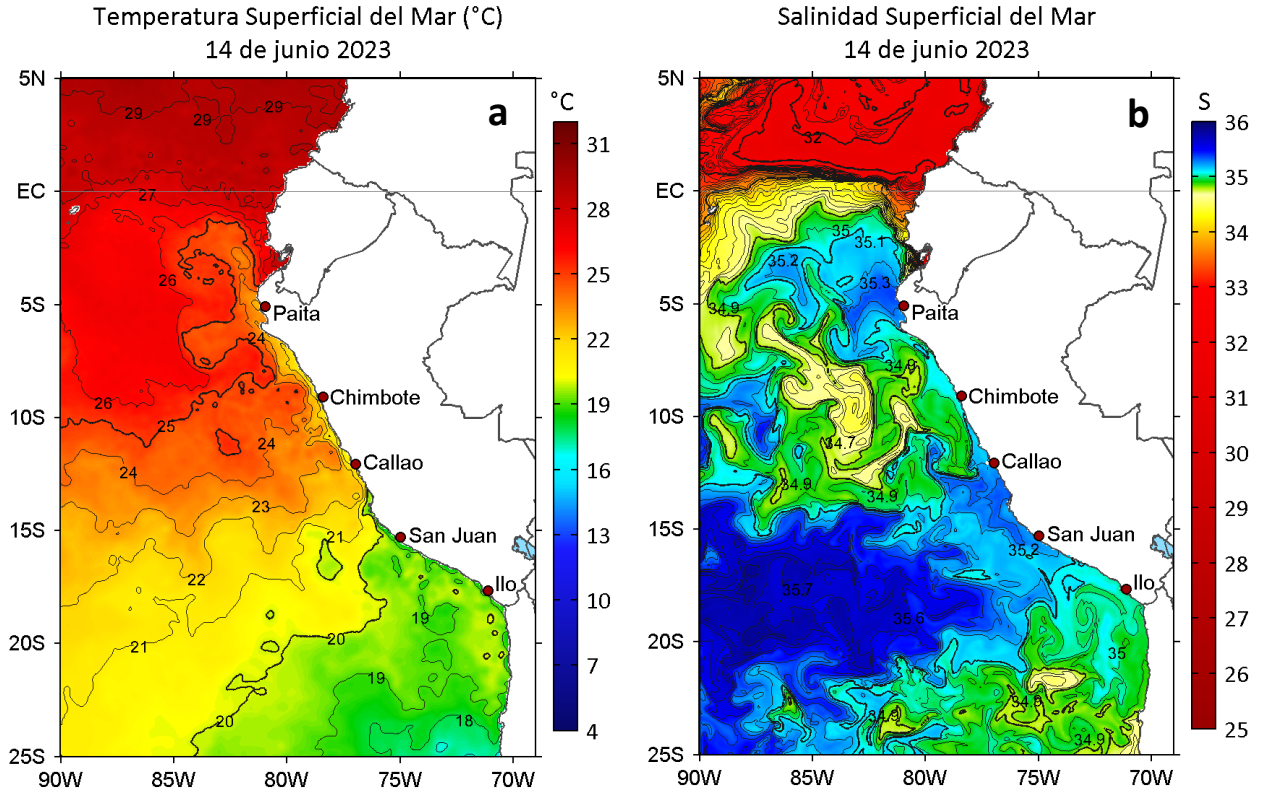
Figura 2. a) Temperatura superficial del mar ( ^{\circ}\text{C} ) y b) Salinidad superficial del mar para el 14 de junio de 2023. Datos: OSTIA-UKMO-L4-GLOB-v2.0 (UK Met Office, 2012; Donlon et al, 2012) y del GLOBAL_ANALYSISFORECAST_PHY_001_024 (Lellouche, J. M. et al, 2013), respectivamente.
