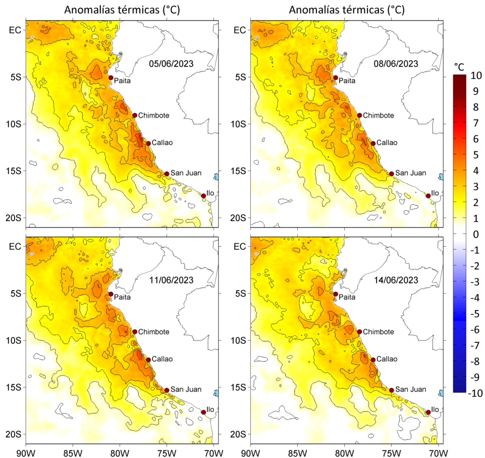
Figura 3. Anomalías de la temperatura superficial del mar ( ^{\circ}\text{C} ) para el a) 05, b) 08, c) 11 y d) 14 de junio de 2023. Las anomalías se calcularon respecto de la climatología para el periodo 2007-2016. Datos: OSTIA-UKMO-L4-GLOB-v2.0 (UK Met Office, 2012; Donlon et al, 2012).
