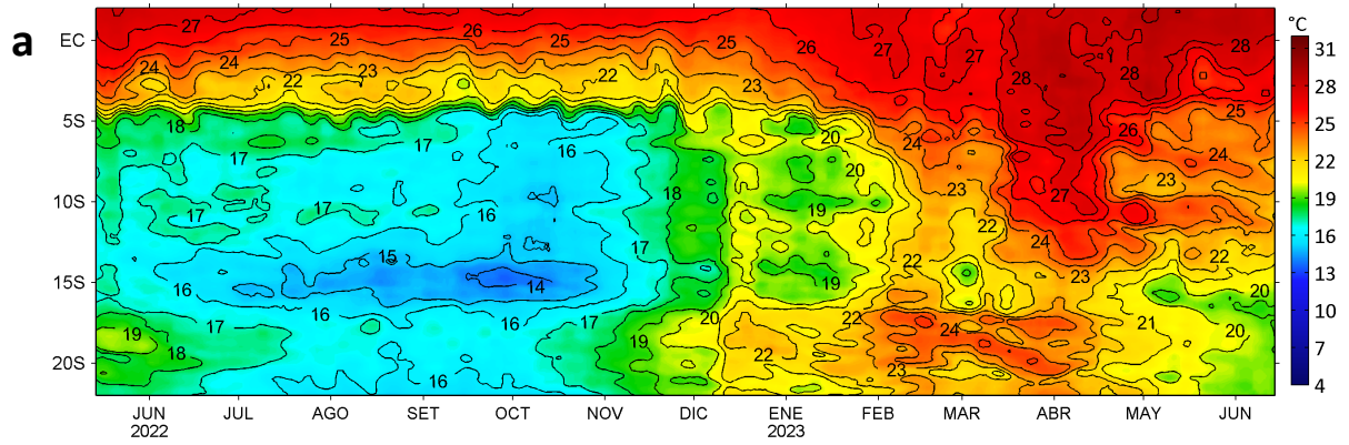
Anomalías de la Temperatura Superficial del mar (°C), franja costera de 60 m.n. 14 de mayo 2022 - 14 de junio 2023
