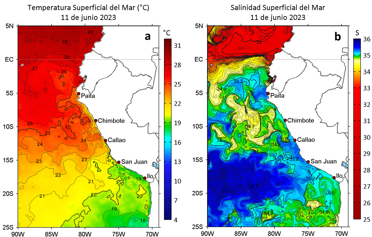
Figura 2. a) Temperatura superficial del mar ( ^{\circ}\text{C} ) y b) Salinidad superficial del mar para el 11 de junio de 2023. Datos: OSTIA-UKMO-L4-GLOB-v2.0 (UK Met Office, 2012; Donlon et al, 2012) y del GLOBAL_ANALYSISFORECAST_PHY_001_024 (Lellouche, J. M. et al, 2013), respectivamente.
