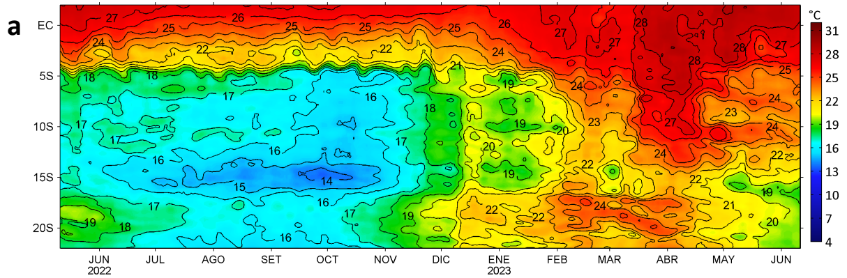
Anomalías de la Temperatura Superficial del mar (°C), franja costera de 60 m.n. 11 de mayo 2022 - 11 de junio 2023
