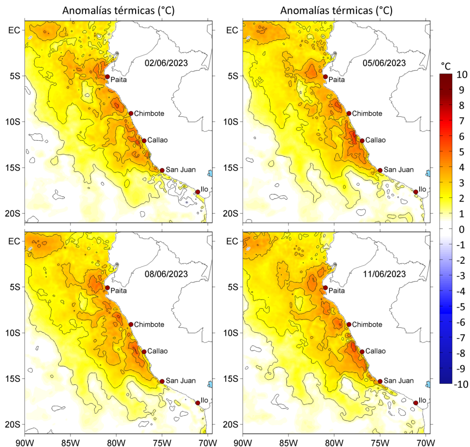
Figura 3. Anomalías de la temperatura superficial del mar ( ^{\circ}\text{C} ) para el a) 02, b) 05, c) 08 y d) 11 de junio de 2023. Las anomalías se calcularon respecto de la climatología para el periodo 2007-2016. Datos: OSTIA-UKMO-L4-GLOB-v2.0 (UK Met Office, 2012; Donlon et al, 2012).
