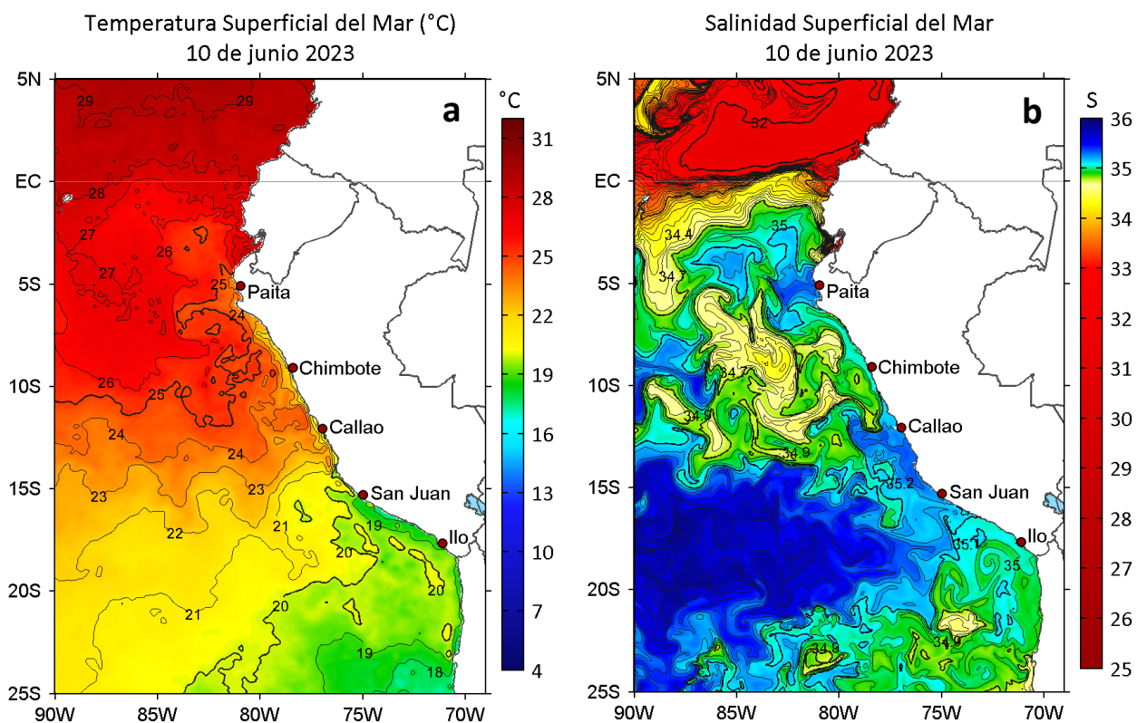
Figura 2. a) Temperatura superficial del mar ( ^{\circ}\text{C} ) y b) Salinidad superficial del mar para el 10 de junio de 2023. Datos: OSTIA-UKMO-L4-GLOB-v2.0 (UK Met Office, 2012; Donlon et al, 2012) y del GLOBAL_ANALYSISFORECAST_PHY_001_024 (Lellouche, J. M. et al, 2013), respectivamente.
