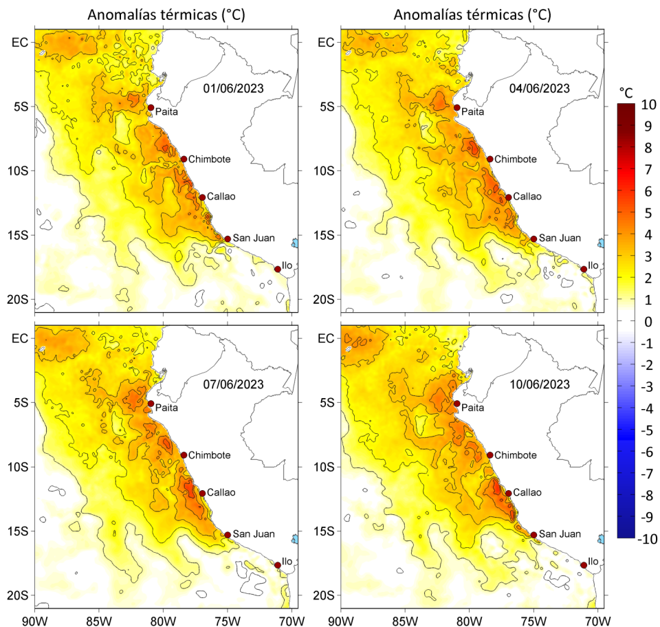
Figura 3. Anomalías de la temperatura superficial del mar ( ^{\circ}\text{C} ) para el a) 01, b) 04, c) 07 y d) 10 de junio de 2023. Las anomalías se calcularon respecto de la climatología para el periodo 2007-2016. Datos: OSTIA-UKMO-L4-GLOB-v2.0 (UK Met Office, 2012; Donlon et al, 2012).
