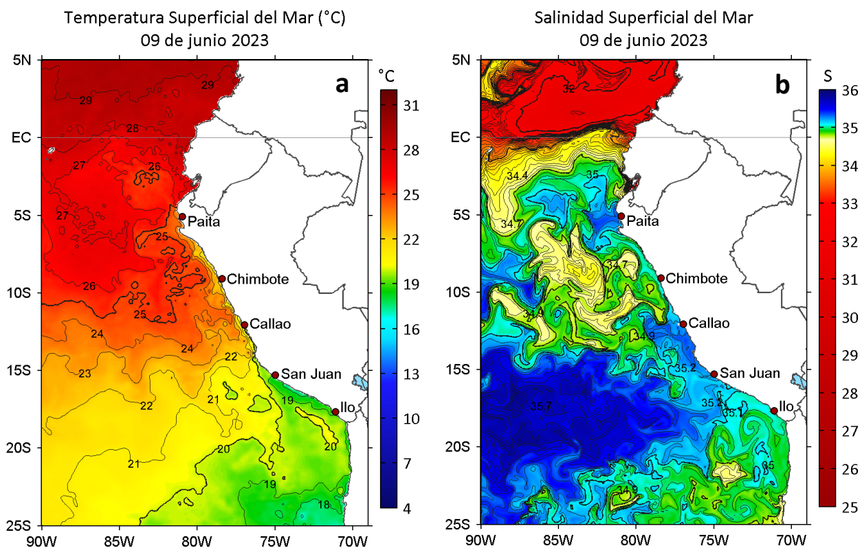
Figura 2. a) Temperatura superficial del mar ( ^{\circ}\text{C} ) y b) Salinidad superficial del mar para el 09 de junio de 2023. Datos: OSTIA-UKMO-L4-GLOB-v2.0 (UK Met Office, 2012; Donlon et al, 2012) y del GLOBAL_ANALYSISFORECAST_PHY_001_024 (Lellouche, J. M. et al, 2013), respectivamente.
