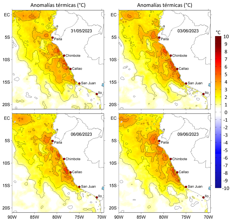
Figura 3. Anomalías de la temperatura superficial del mar ( ^{\circ}\text{C} ) para el a) 31 de mayo, b) 03, c) 06 y d) 09 de junio de 2023. Las anomalías se calcularon respecto de la climatología para el periodo 2007-2016. Datos: OSTIA-UKMO-L4-GLOB-v2.0 (UK Met Office, 2012; Donlon et al, 2012).
