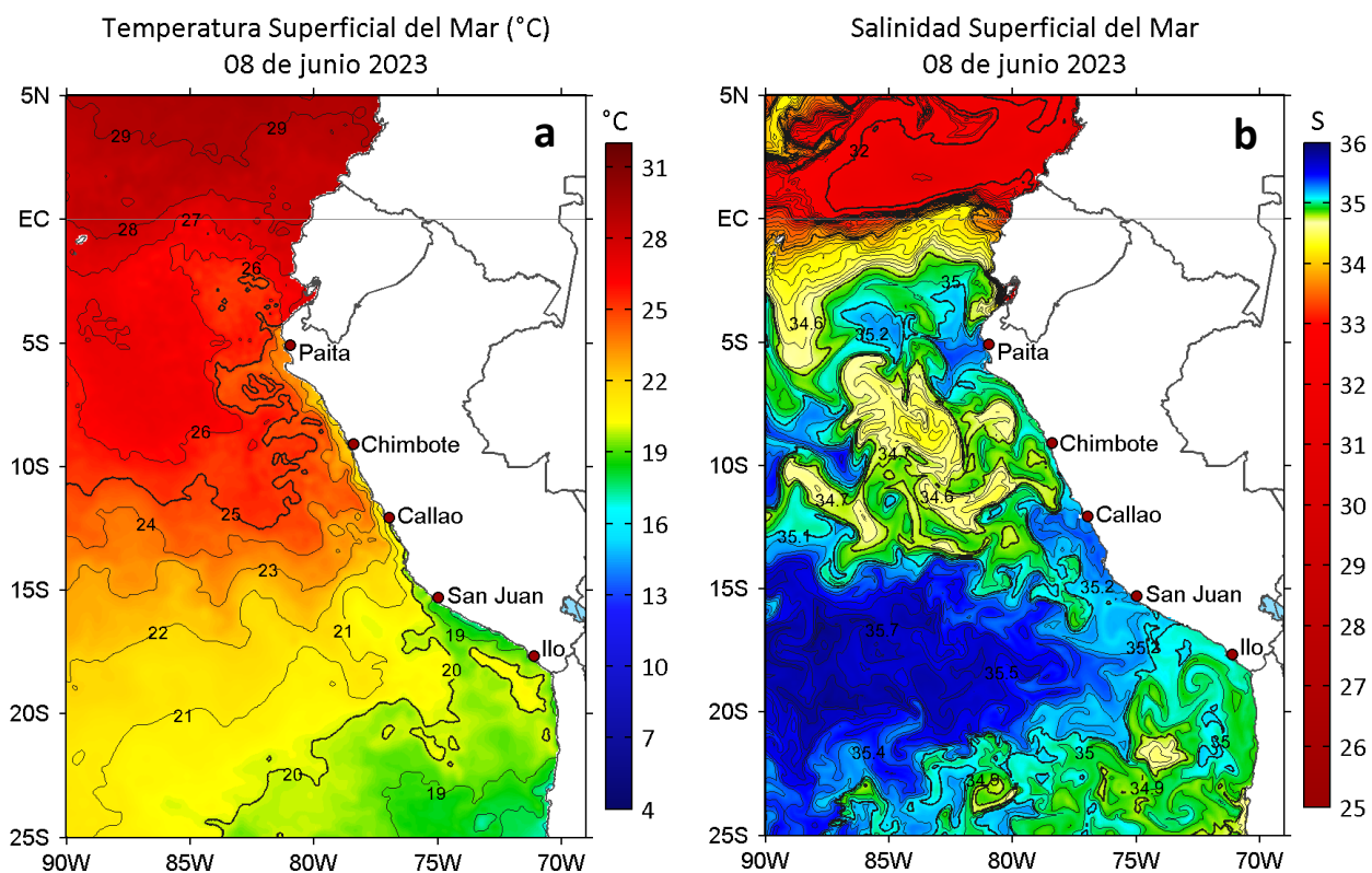
Figura 2. a) Temperatura superficial del mar ( ^{\circ}\text{C} ) y b) Salinidad superficial del mar para el 08 de junio de 2023. Datos: OSTIA-UKMO-L4-GLOB-v2.0 (UK Met Office, 2012; Donlon et al, 2012) y del GLOBAL_ANALYSISFORECAST_PHY_001_024 (Lellouche, J. M. et al, 2013), respectivamente.
