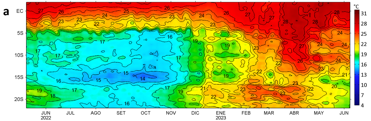
Anomalías de la Temperatura Superficial del mar (°C), franja costera de 60 m.n. 08 de mayo 2022 - 08 de junio 2023
