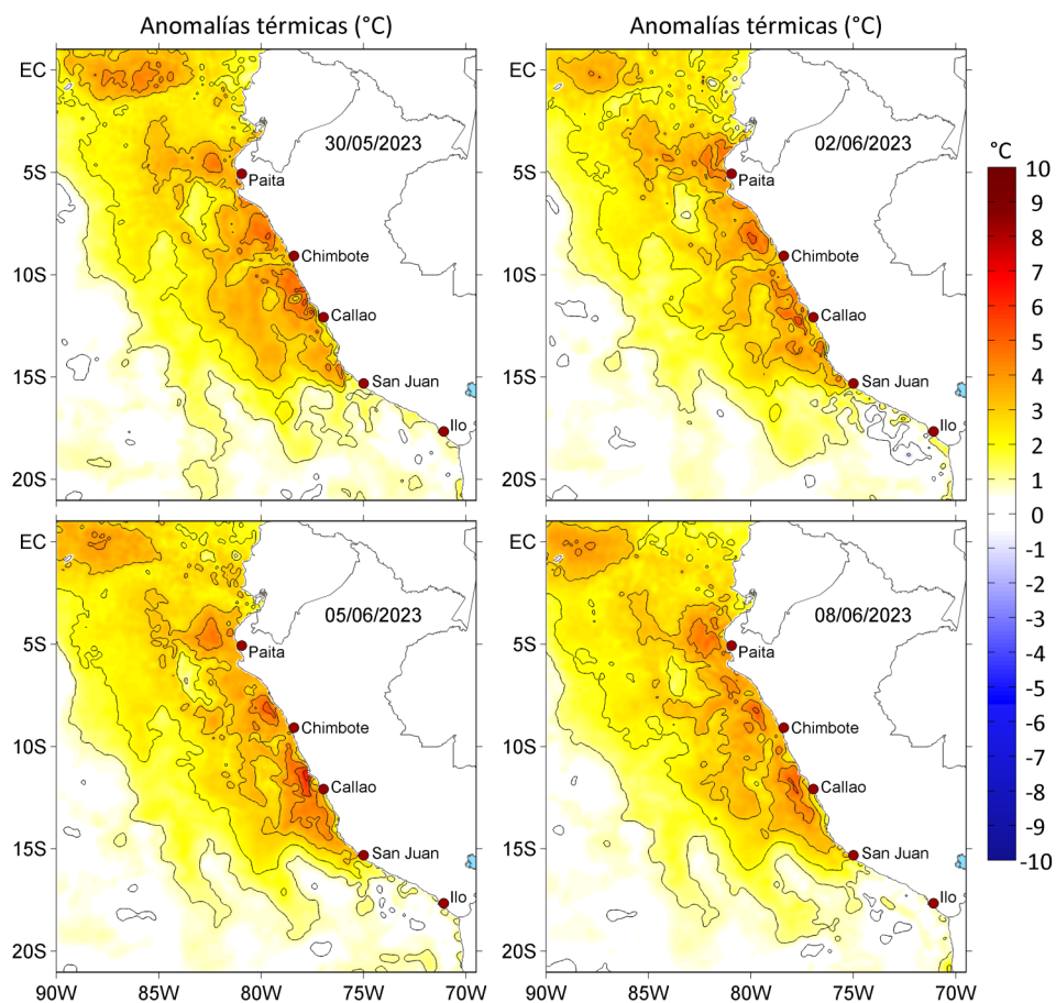
Figura 3. Anomalías de la temperatura superficial del mar ( ^{\circ}\text{C} ) para el a) 30 de mayo, b) 02, c) 05 y d) 08 de junio de 2023. Las anomalías se calcularon respecto de la climatología para el periodo 2007-2016. Datos: OSTIA-UKMO-L4-GLOB-v2.0 (UK Met Office, 2012; Donlon et al, 2012).
