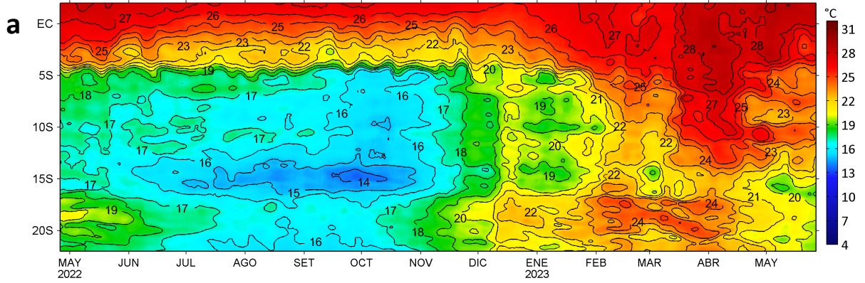
Anomalías de la Temperatura Superficial del mar (°C), franja costera de 60 m.n. 26 de abril 2022 - 27 de mayo 2023
