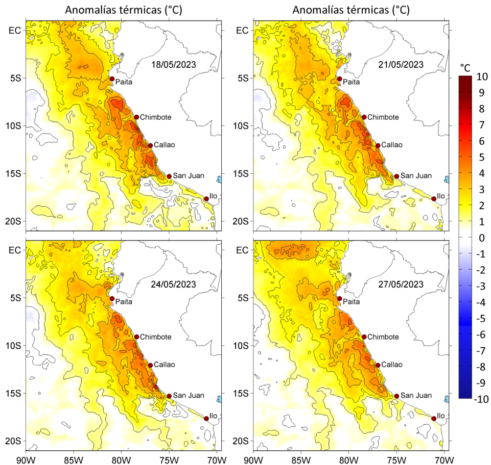
Figura 3. Anomalías de la temperatura superficial del mar ( ^{\circ}\text{C} ) para el a) 18, b) 21, c) 24 y d) 27 de mayo de 2023. Las anomalías se calcularon respecto de la climatología para el periodo 2007-2016. Datos: OSTIA-UKMO-L4-GLOB-v2.0 (UK Met Office, 2012; Donlon et al, 2012).
