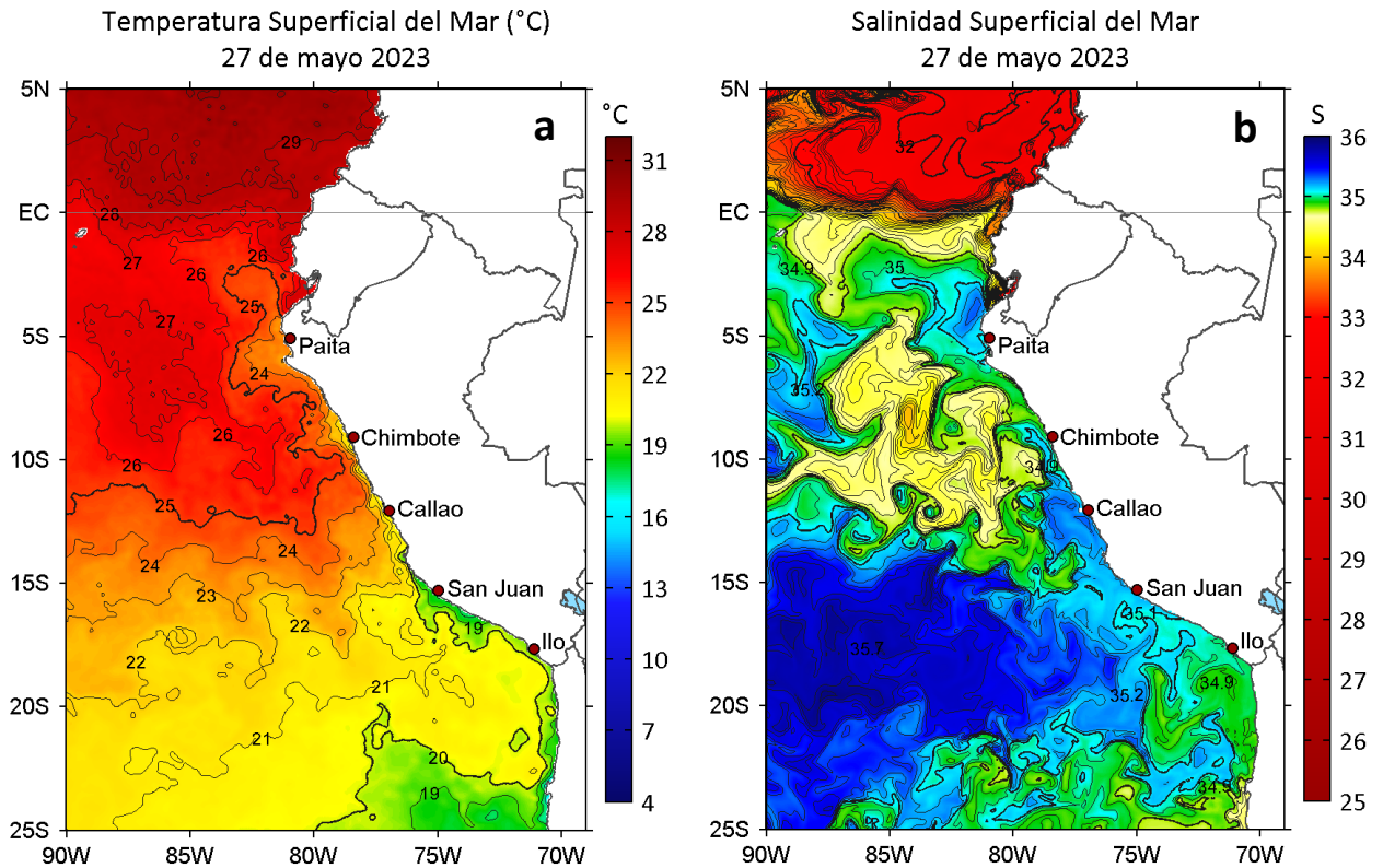
Figura 2. a) Temperatura superficial del mar ( ^{\circ}\text{C} ) y b) Salinidad superficial del mar para el 27 de mayo de 2023. Datos: OSTIA-UKMO-L4-GLOB-v2.0 (UK Met Office, 2012; Donlon et al, 2012) y del GLOBAL_ANALYSISFORECAST_PHY_001_024 (Lellouche, J. M. et al, 2013), respectivamente.
